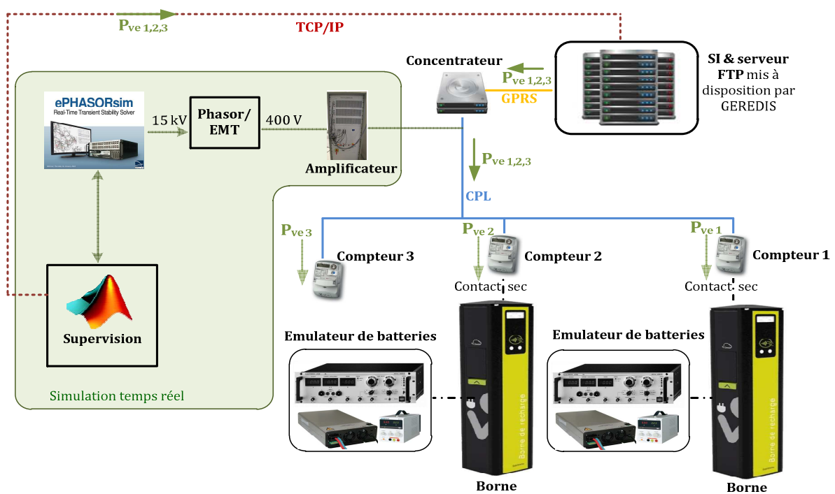
Figure 5.18 : Éléments et architecture du système de puissance et de communication.
