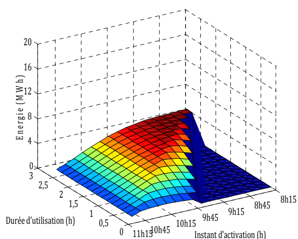
Figure 4.81 : Estimation de l'énergie facturée à l'acteur d'ajustement.
