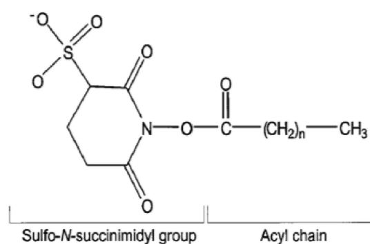
Figure 21 : Structure du SSO (Coort et al., 2002)
