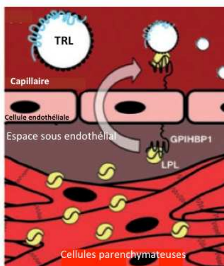
Figure 11 : Synthèse de la LPL et phénomène de lipolyse intravasculaire d'après (S. G. Young et al. 2011). GPIHBP1 : GlycosylPhosphatidylInositol-anchored High density lipoprotein Binding Protein 1 ; LPL : LipoProteine Lipase ; TRL : Triglyceride Rich Protein .
