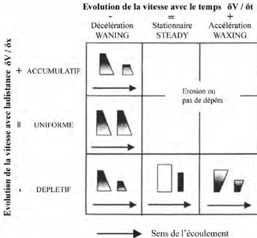
Figure 3 : Modèle de Kneller montrant l'évolution temporelle et spatiale des écoulements (Kneller, 1995, Kneller et Branney, 1995).
