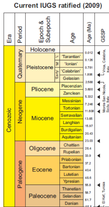
Figure 29 : Stratigraphie détaillée du Cénozoïque actuellement en cours de validité (Gibbard et Head, 2009).
