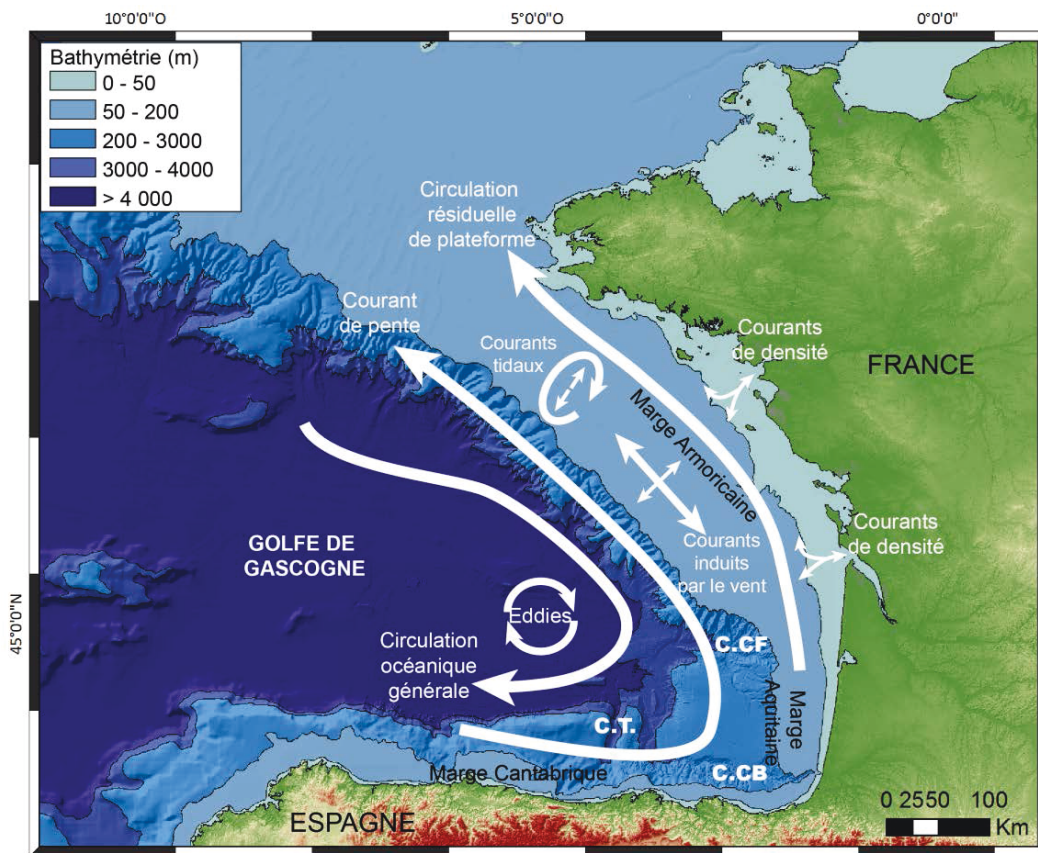
Figure 28 : Schéma de la circulation océanique dans le Golfe de Gascogne. C.CF : Canyon du Cap-Ferret. C.CB : Canyon de Capbreton. C.T. : Canyon de Torrelavega. Adaptée d'après Koustikopoulos et Le Cann (1996) et Mulder et al. (2012).
