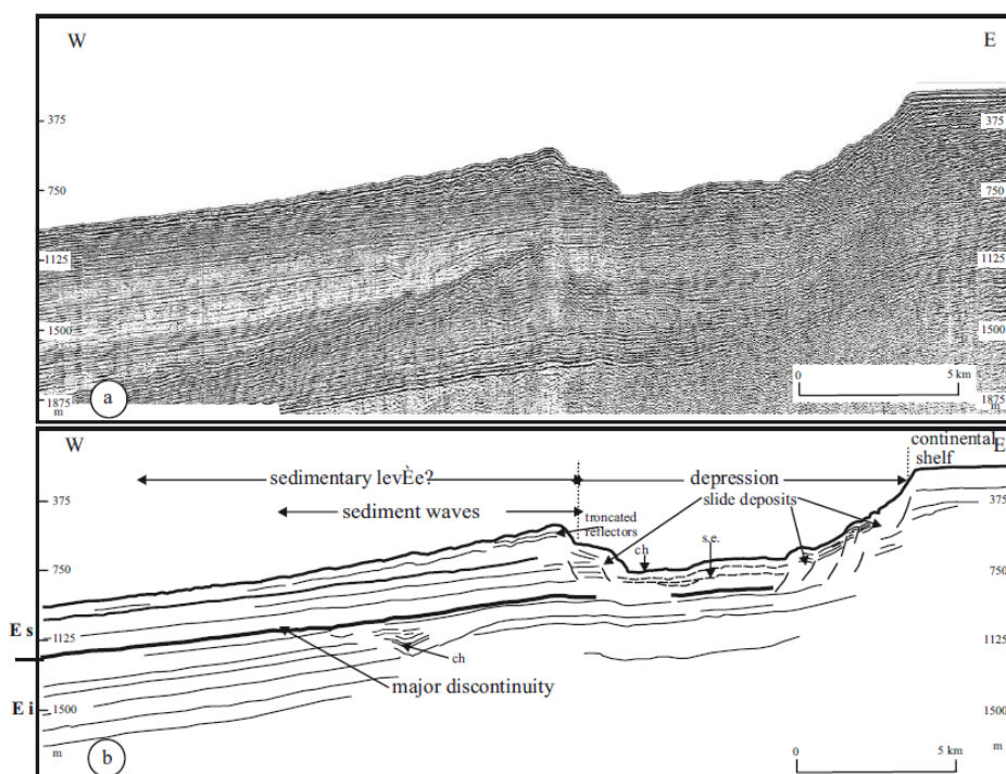
Figure 45 : Profil sismique Itrs29 traversant le glissement landais avec son interprétation (Gonthier et al. , 2006). Localisation en Figure 43.
