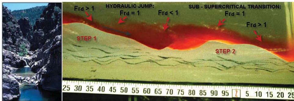
Figure 15 : A : Chutes-and-pools - B : Cyclic steps (Kostic, 2011).
