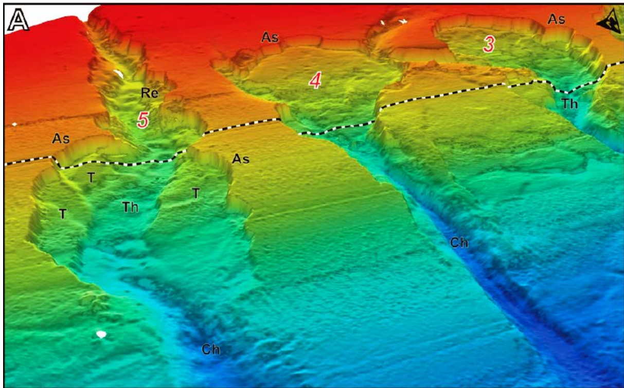
Figure 5 : Morphologie des têtes arrondies des canyons du Petit Banc des Bahamas (Mulder et al. , 2012)
