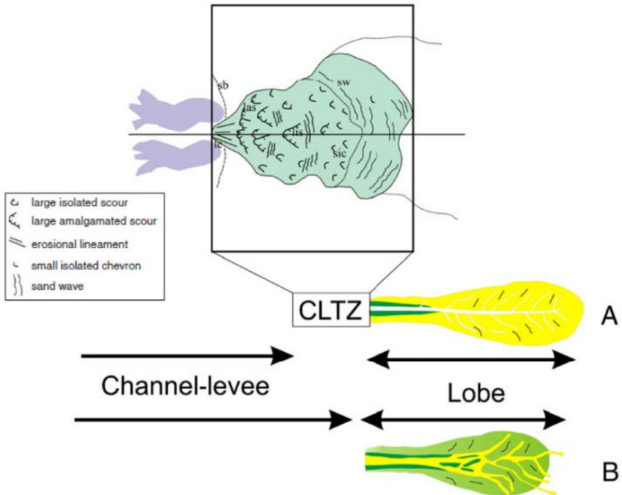
Figure 11 : Représentation d'une zone de transition chenel-lobes (CLTZ (Wynn et al. , 2002)). A : cas d'un lobe sableux. B : cas d'un lobe argileux (Wynn et Stow, 2002, Bonnel, 2005).
