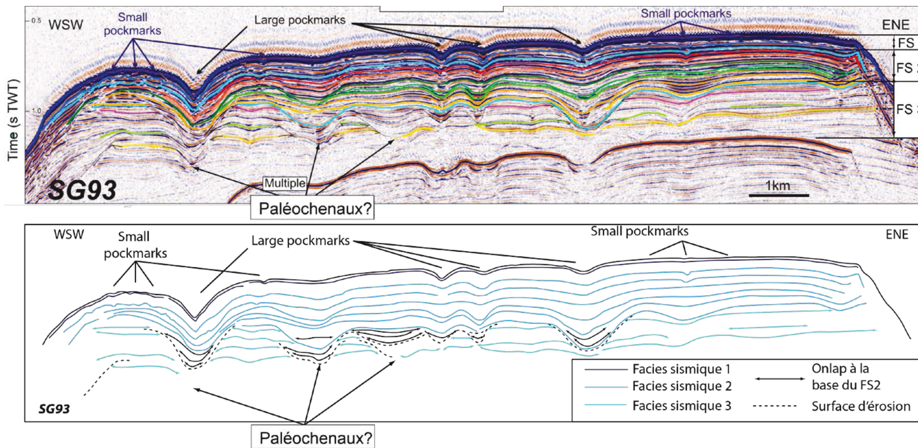
Figure 42 : Interprétation du profil SG93 : y sont représentés les trois faciès sismiques identifiées (le faciès 2 étant prépondérant). Une surface d'érosion est mise en évidence, soulignant l'existence de possibles paléochenaux. Modifié d'après Baudon et al. , 2013.
