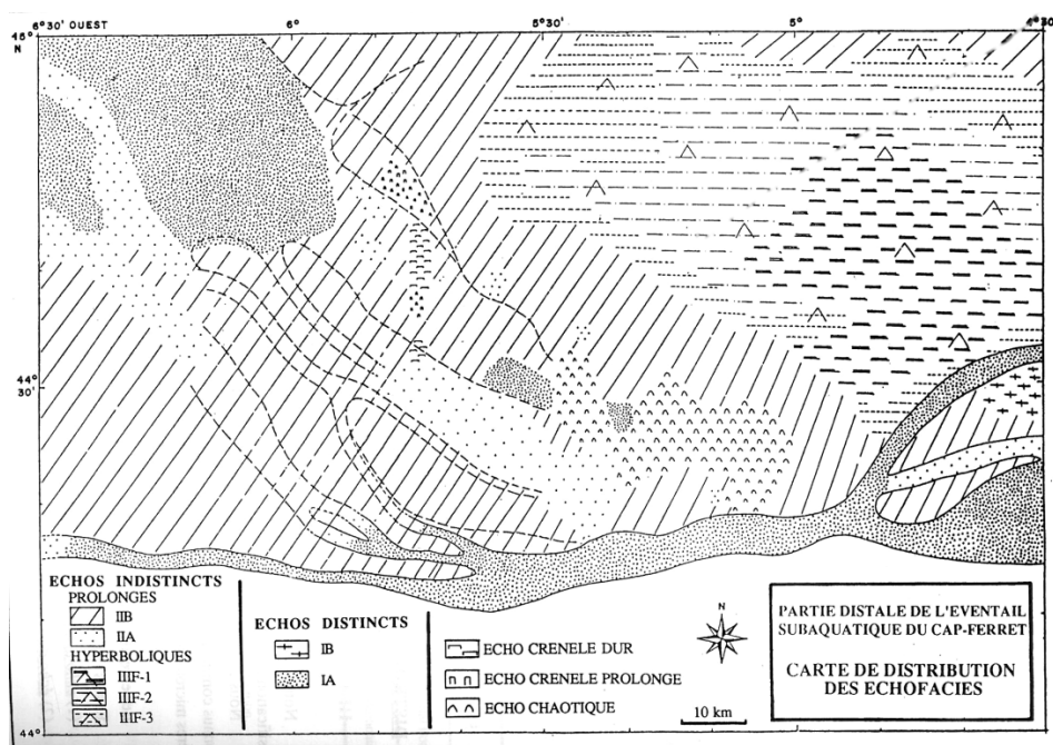
Figure 46 : Carte des écho-faciès 3,5 kHz de la zone distale du système turbiditique Cap-Ferret Capbreton réalisée par Mezerais (1991).
