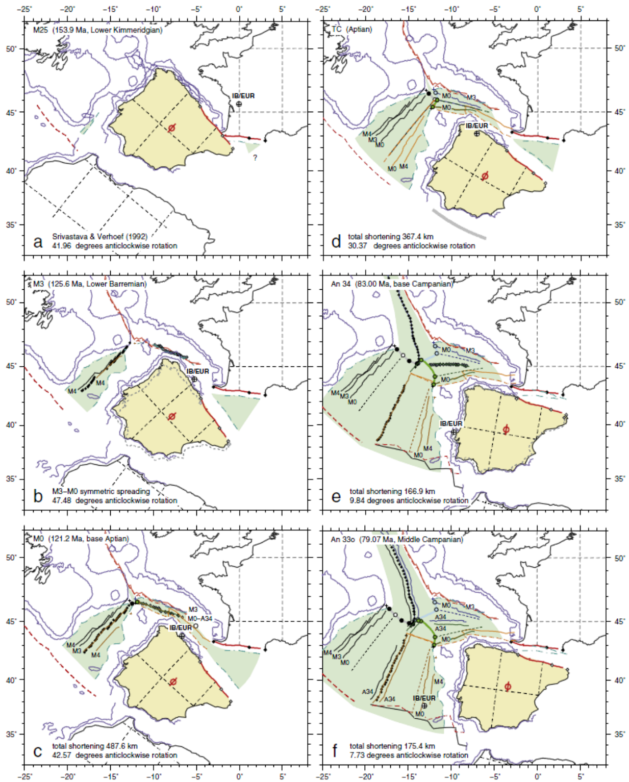
Figure 20 : Reconstitutions de l'Atlantique Nord entre l'Afrique et les îles britanniques en 6 schémas du le Jurassique supérieur au Crétacé terminal selon Vissers (2012b). Ce modèle illustre plutôt la théorie de l'ouverture en ciseaux.
