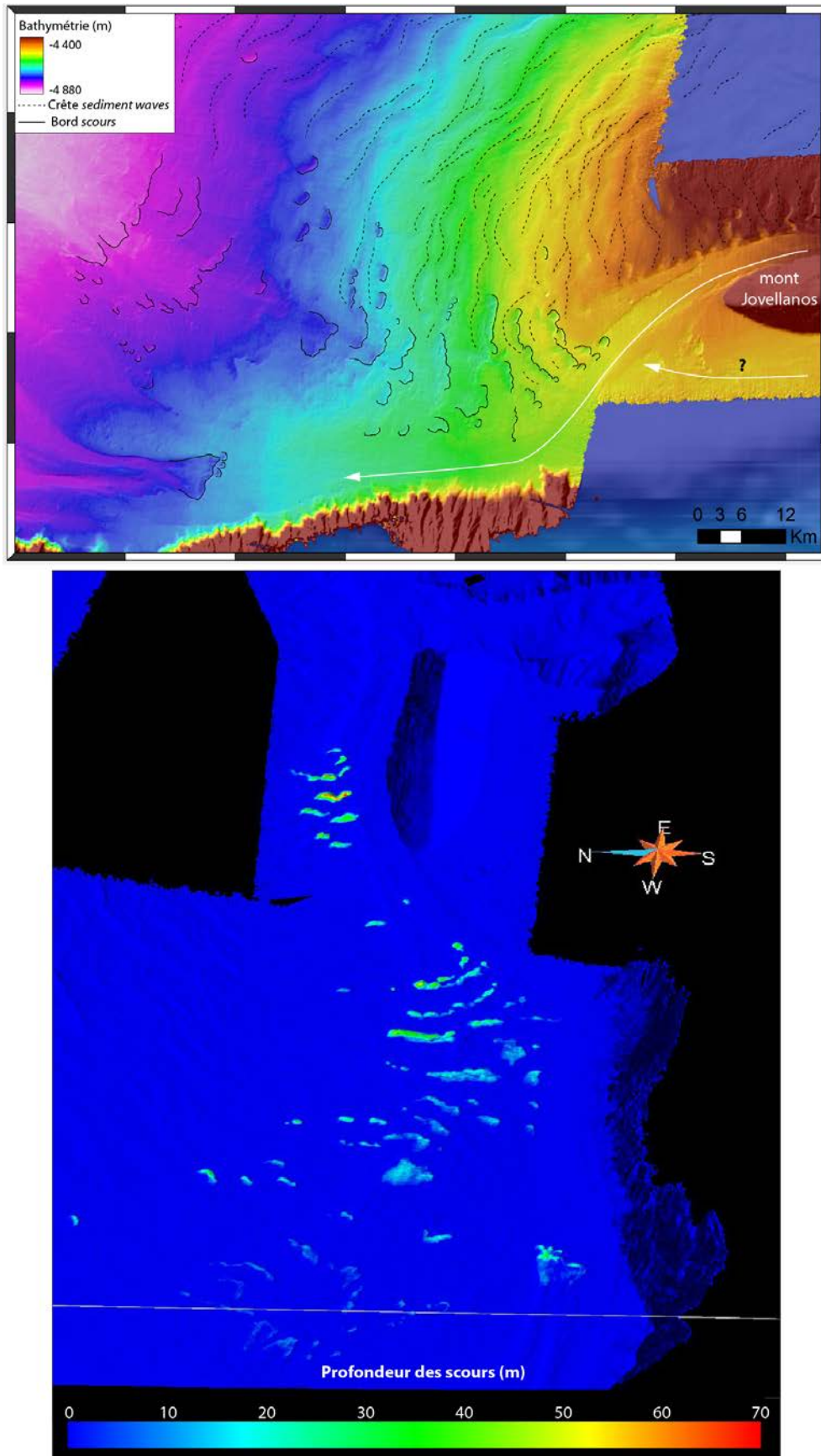
Figure 144 : Zoom sur la CLTZ du Cap-Ferret. En haut : Carte bathymétrique ombrée, les crêtes des sediment waves sont soulignés ainsi que les bordures des scours . Bas : Cartographie 3D de la profondeur des scours (Exagération verticale *2,5).
