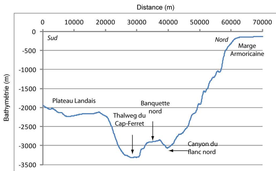
Figure 37 : Le système turbiditique du Cap-Ferret selon les limites et nomenclatures de Cremer (1983) sur fond bathymétrique ombrée ZEE et SARGASS. Le trait en pointillé de la carte bathymétrique correspond à la coupe bathymétrique transversale en bas, montrant la morphologie en U du canyon de Cap-Ferret.
