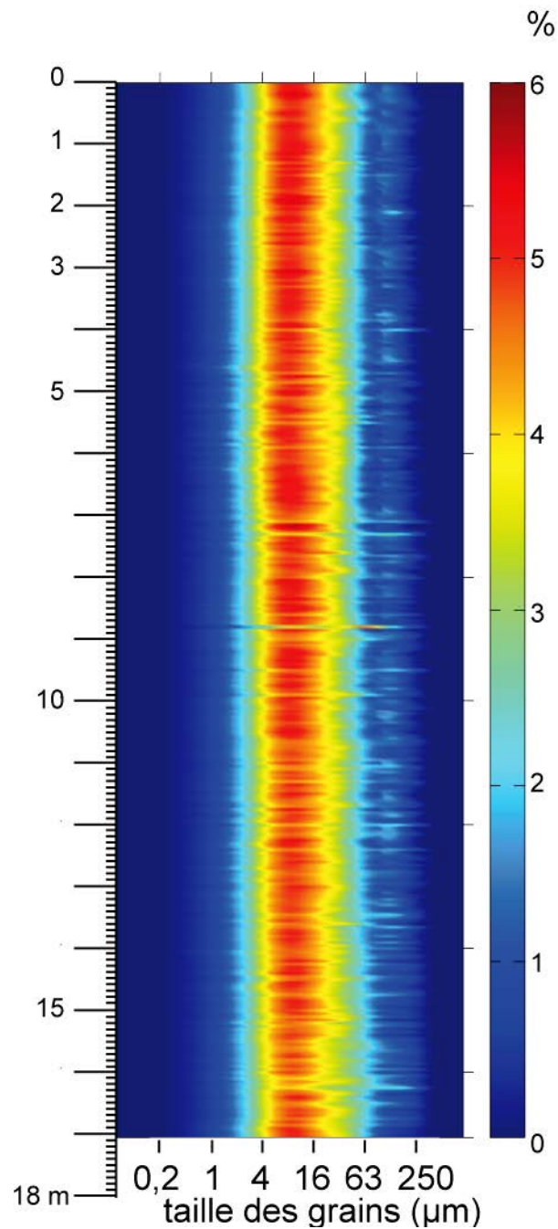
Figure 61 : Exemple de cartographie de la granularité (carotte PP10-09). Pour chaque échantillon analysé (ici tous les 5 cm), la proportion de grains de chaque classe granulométrique est reportée à la quantité totale de grains (%). La profondeur du prélèvement dans la carotte est représentée en ordonnée et les variations colorimétriques de la ligne associées indiquent le pourcentage de représentation de la classe granulométrique représentée en abscisse. Sur cette exemple, l'axe rouge-orangé entre 4 et 16 µm indique que ces classes granulométriques que les plus fortes proportions sont présentes : la carotte contient des sédiments à mode granulométrique dominant silto-argileux. Ponctuellement, l'intensité de couleur se déplace vers des classes plus élevées comme à 980 cm : cela met en évidence un niveau de sables fins.
