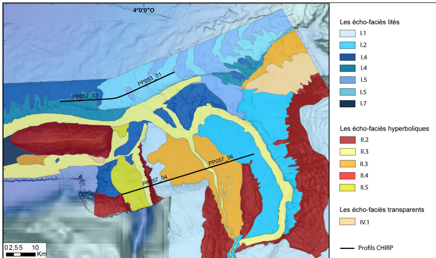
Figure 123 : Carte des écho-faciès de la zone de confluence.
