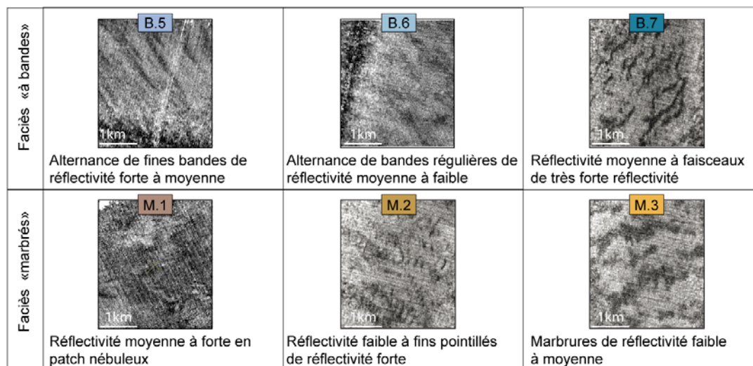
Figure 113 : Suite de la classification des faciès de réflectivité du fond marin dans la zone distale du système turbiditique du Cap-Ferret-Capbreton.
