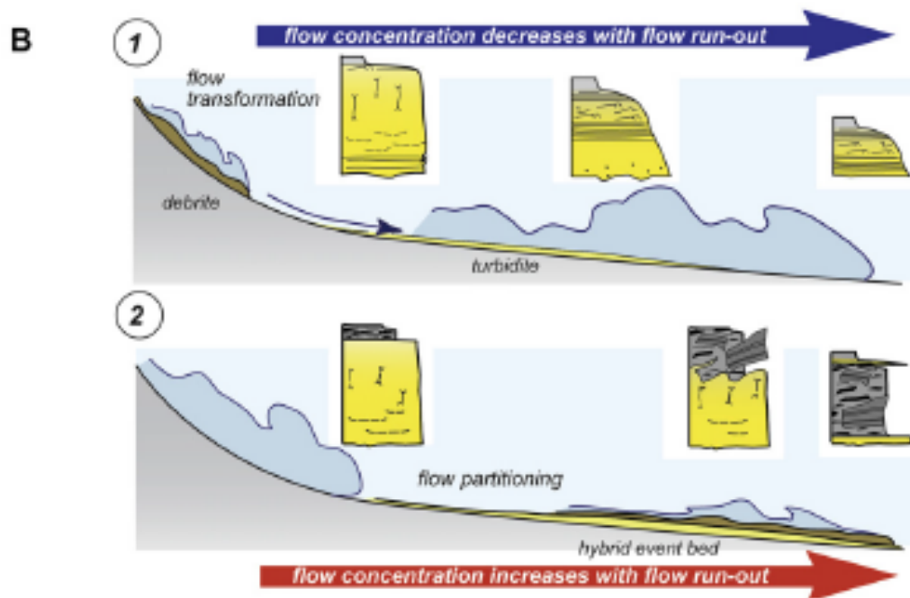
Figure 13 : A : Schéma de classification des dépôts mis en place par écoulements gravitaires en fonction de leur nature cohésive, non-cohésive ou transitionnelle (écoulements hybrides). B : Les dépôts de débris et turbidites dominent les dépôts des systèmes turbiditiques marins profonds et correspondent à une dilution de plus en plus importante de l'écoulement gravitaire vers l'aval. Cependant, certains systèmes montrent des dépôts de type plus cohésif en terminaison de systèmes (frange) qui sont interprétés comme résultant d'écoulements hybrides (Haughton et al. , 2009).
