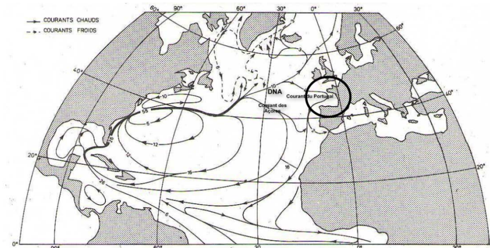
Figure 27 : Circulation des courants dans l'Atlantique Nord. D'après Reffray et al. , 2008.
