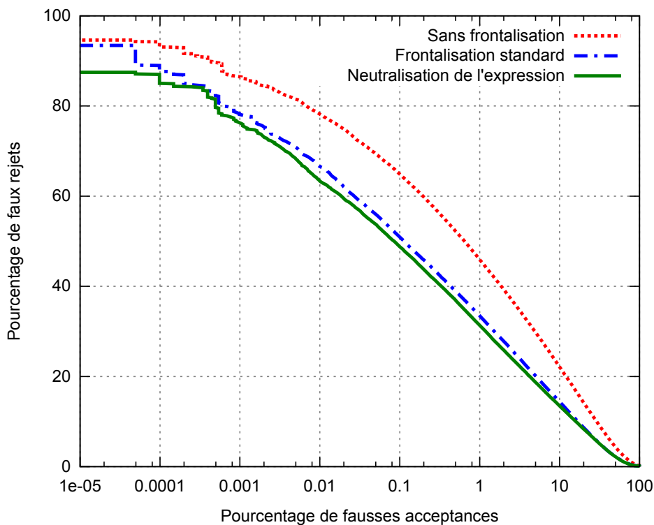
FIGURE 4.35 – Courbes ROC sur la base V
