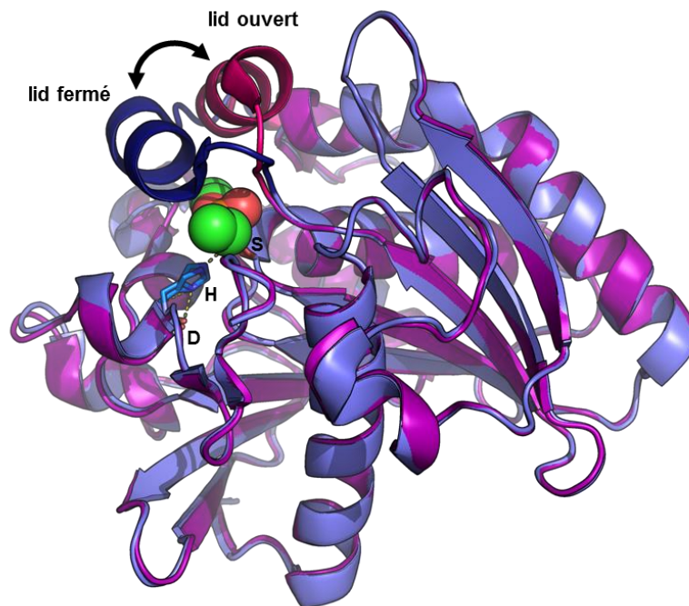
Figure 8. Structure de la lipase de Rhizomucor miehei avec le lid en conformation fermée en bleu (PDB ID : 3GTL) (Brzozowski et al. 1992) et en conformation ouverte en violet (PDB ID : 4GTL) (Derewenda et al. 1992a). L'inhibiteur suicide, le diéthylphosphonate, est représenté en sphères colorées en vert, il est présent uniquement dans la conformation ouverte. Les acides aminés catalytiques représentés en sticks sont indiqués, D pour l'aspartate 203, H pour l'histidine 257 et S pour la sérine 144.
