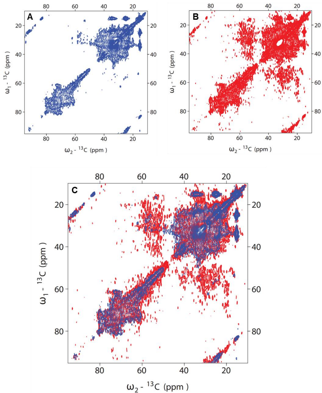
Figure 9. Spectres de corrélation 2D {}^{13}\text{C} - {}^{13}\text{C} DARR obtenus sur des préparations d'enveloppe cellulaires de ( {}^{13}\text{C} , {}^{15}\text{N} )- E. coli avec ou sans induction de KpOmpA. A. Echantillon non-induit. B. Echantillon Induit. C. Superposition des spectres des échantillons non-induit (A), en bleu, et induit (B), en rouge. L'ensemble des données RMN ont été obtenues sur un spectromètre Bruker Avance III HD opérant à une fréquence de Larmor {}^1\text{H} de 700 MHz et équipé d'une sonde MAS E-Free 3.2 mm (Bruker BioSpin). Les expériences 2D {}^{13}\text{C} - {}^{13}\text{C} DARR ont été enregistrées à une fréquence de rotation de 12 KHz et à une température de +2°C en utilisant un temps de mélange de 50 ms et un temps d'acquisition de 38 heures.
