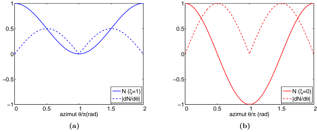
Figure IV.4 : Fonctions directionnelles \mathcal{N} (traits continus) et leur variation \frac{d\mathcal{N}}{d\theta} (traits pontillés) pour : (a) un microphone cardioïde et (b) un microphone bidirectionnel, en fonction de la direction de la source.
