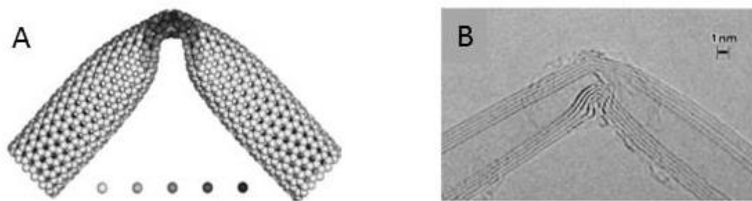
Figure I.3. A) Simulation de la structure atomique d'un coude obtenu par pliure d'un SWCNTs et B) micrographie en champ clair du coude formé sur un MWCNTs sous contraintes mécaniques [24].
