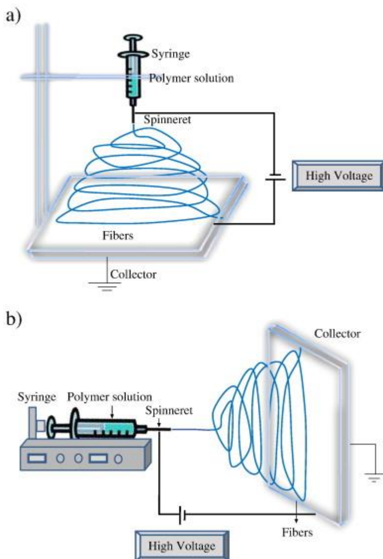
Schéma I.3. Représentation schématique du procédé d'électrofilage. a) installation verticale et b) installation horizontale [99].
