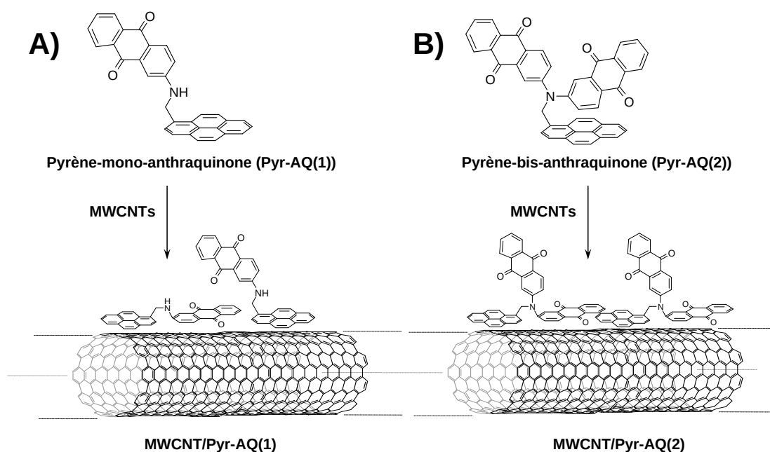
Schéma II.1. Schéma du pyrène-mono-anthraquinone A) et pyrène-bis-anthraquinone B) et de leur greffage sur les nanotubes de carbone multifeuilletés par interactions- \pi .
