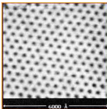
FIGURE 11 – Observation de vortex dans un supraconducteur – Hess et al. [55]
