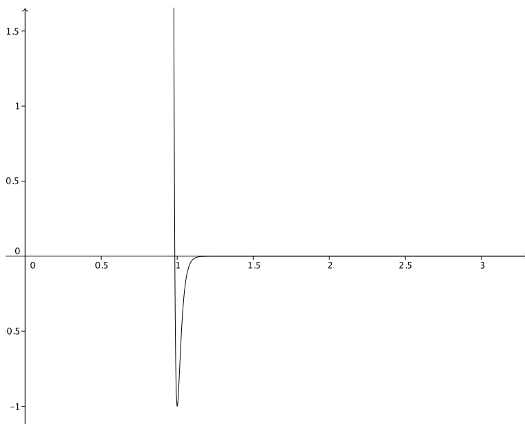
FIGURE 1 – Un exemple de potentiel de Theil V_\alpha
