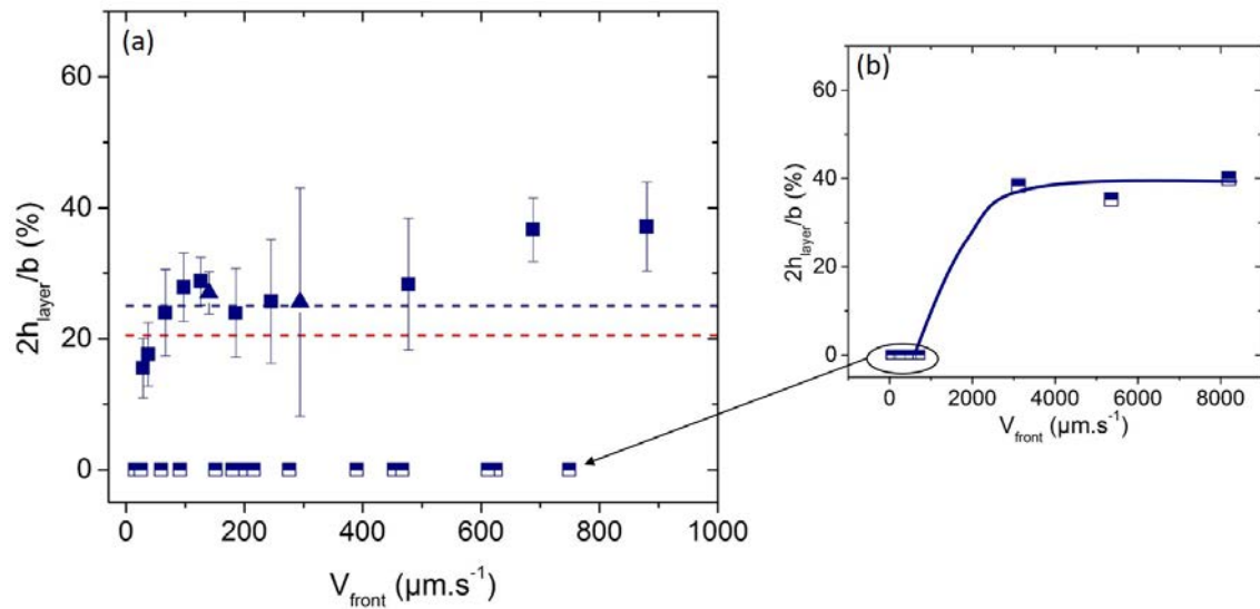
FIGURE E.6 – (a) Epaisseur du film adimensionnée par la demi-largeur du canal qui est laissé aux parois du canal en fonction de la vitesse de l'interface (prise à x = L/2 ) lors du déplacement d'un microgel 2.2 % (carrés) ou 3% (triangles) par une solution de microgel 1.6% dans des systèmes sans (symboles pleins) et avec (symboles mi-pleins) glissement. La ligne en pointillés bleus correspond à la valeur expérimentale asymptotique de l'épaisseur du film lors du déplacement d'un fluide à seuil par un autre déterminée à plus grande échelle dans [58]. La ligne en pointillés rouges correspond au modèle de recirculation présenté dans [58]. (b) Epaisseur du film adimensionnée par la demi-largeur du canal qui est laissé aux parois du canal en fonction de la vitesse de l'interface (prise à x = L/2 ) lors du déplacement d'un microgel 2.2 % (carrés) par une solution de microgel 1.6% dans des systèmes avec glissement. Les lignes continues sont des guides pour les yeux.
