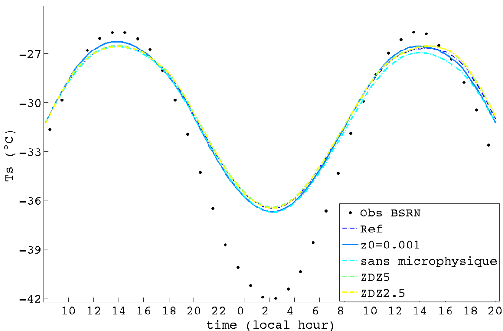
FIGURE 4.24 – Cycle journalier de la température de la surface de neige T_s en (°C) d'après les observations du BSRN et pour plusieurs simulations Méso-NH.
