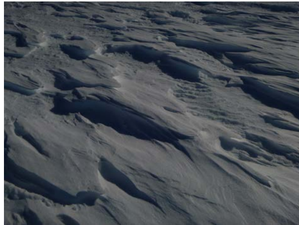
FIGURE 1.10 – Sastrugi à D17 : motifs tranchants de la surface neigeuse résultant de l'érosion par le vent.
