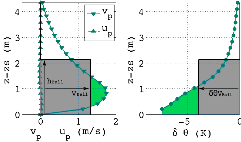
FIGURE 5.15 – Détermination des paramètres pour le modèle de Ball, à partir des profils de vitesse v_p et d'écart à la température \delta\theta .
