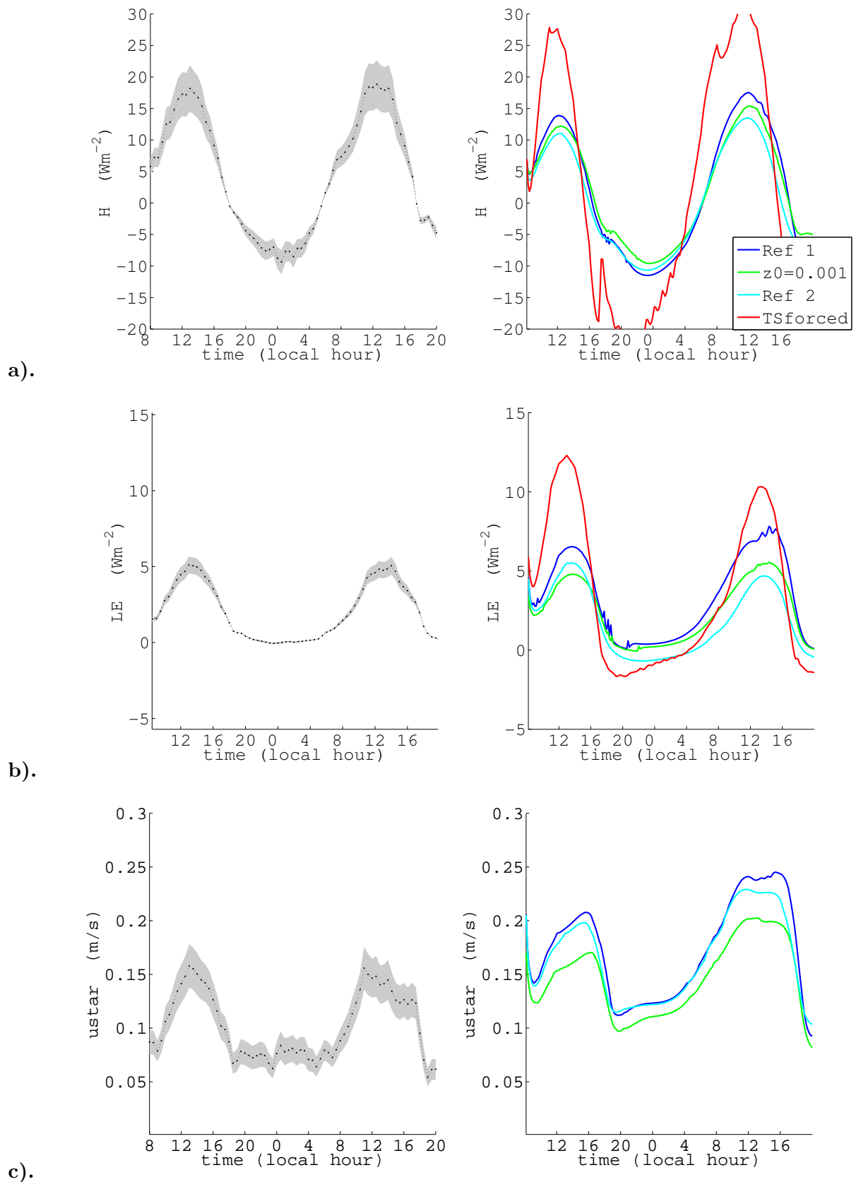
FIGURE 4.34 – Flux de chaleur en surface, et vitesse de frottement.
