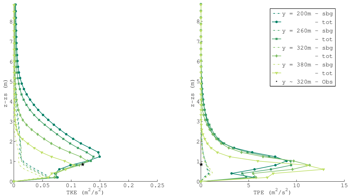
FIGURE 5.17 – Profils verticaux de TKE et TPE sous-maïlle et totales, pour les quatre points d'étude. Les signes \star repèrent les données d'observation.
