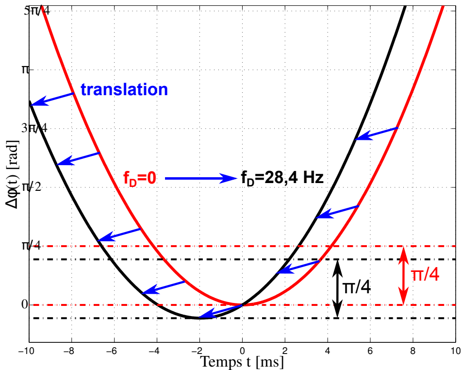
FIGURE 5.7 – Exemples de distribution de phase azimuth calculées à partir de l'expression (5.70) dans la configuration de SWOT. En rouge, le cas où la surface observée est immobile ( f_D = 0 ), en noir, le cas où un vent à 10 m de 6 \text{ m.s}^{-1} souffle ( f_D = 28,4 \text{ Hz} ). La courbe noire est une translation dans le plan (temps, phase) de la courbe rouge.
