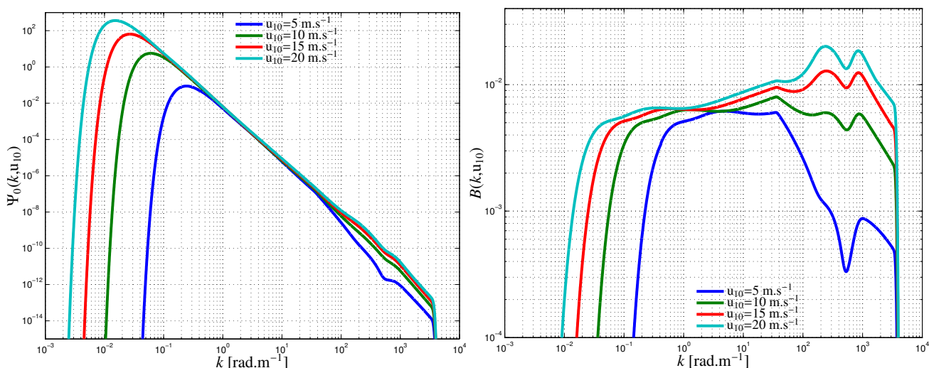
FIGURE 2.4 – Spectres de puissance de l'élévation (à gauche) et de courbures (à droite) omnidirectionnels de Kudryavtsev et al. [1999] pour différentes vitesses de vent à 10 m.
