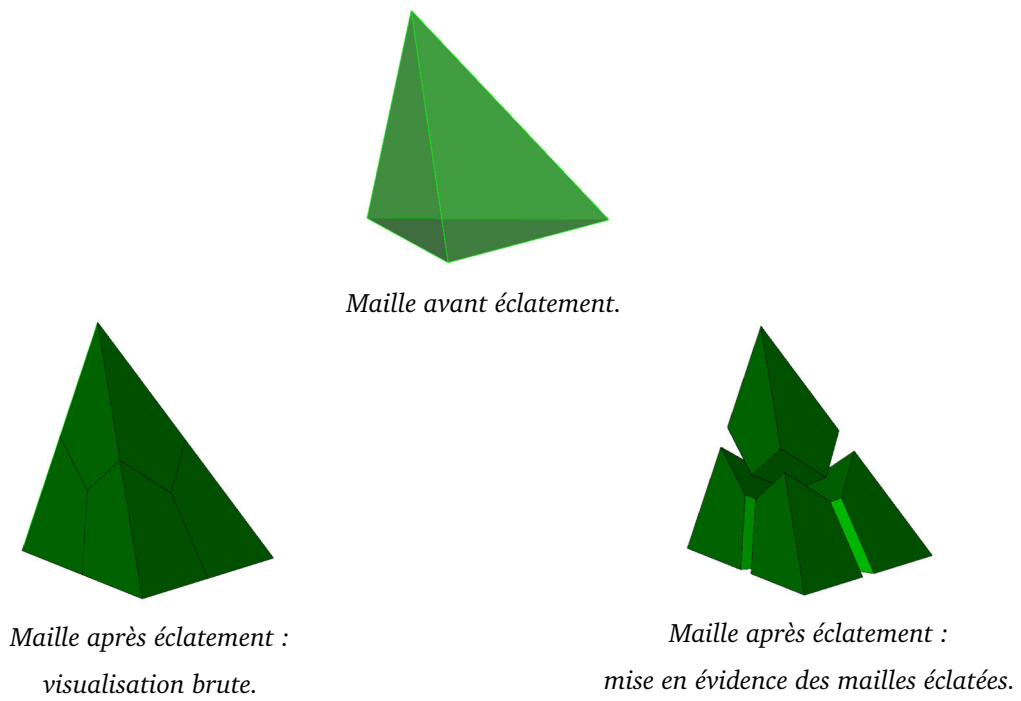
FIG. 51. – Éclatement du tétraèdre à quatre points de Gauss.
