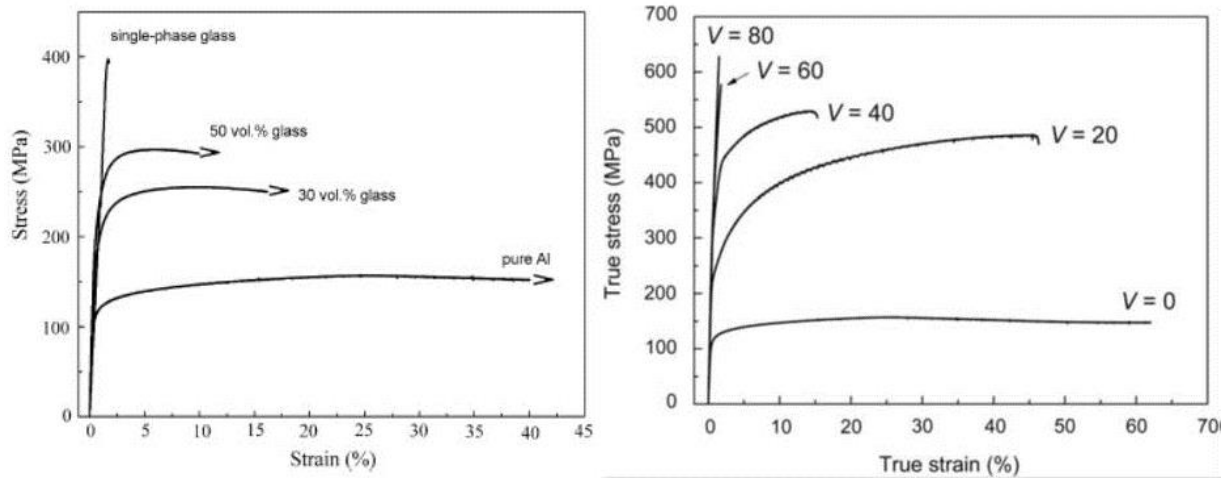
Figure 1.15 :a) Comportement mécanique à température ambiante d'une série de composites Al/ verre métallique AlYNiCo [73] ; b) comportement mécanique à température ambiante d'une série de composites Al/ \beta -Al 3 Mg 2 [74].
