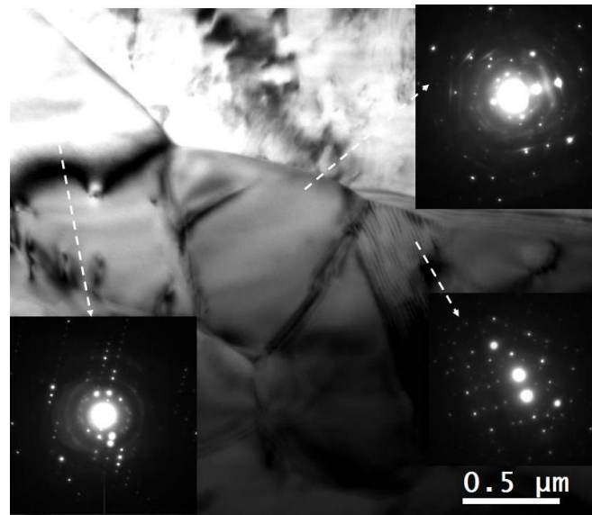
Figure 5.15: Microstructure d'un échantillon Mg- \gamma 50% après déformation \varepsilon = 0.3 à 300^\circ\text{C} ( t = 35 min) (image MET en champ clair) : le liseré \gamma -Mg 17 Al 12 est formé des particules séparées par des joints de grains de forte désorientation d'après les diagrammes de diffraction.
