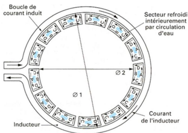
Figure 3.6 : Vue de dessus d'un creuset froid sectorisé et de son inducteur.
