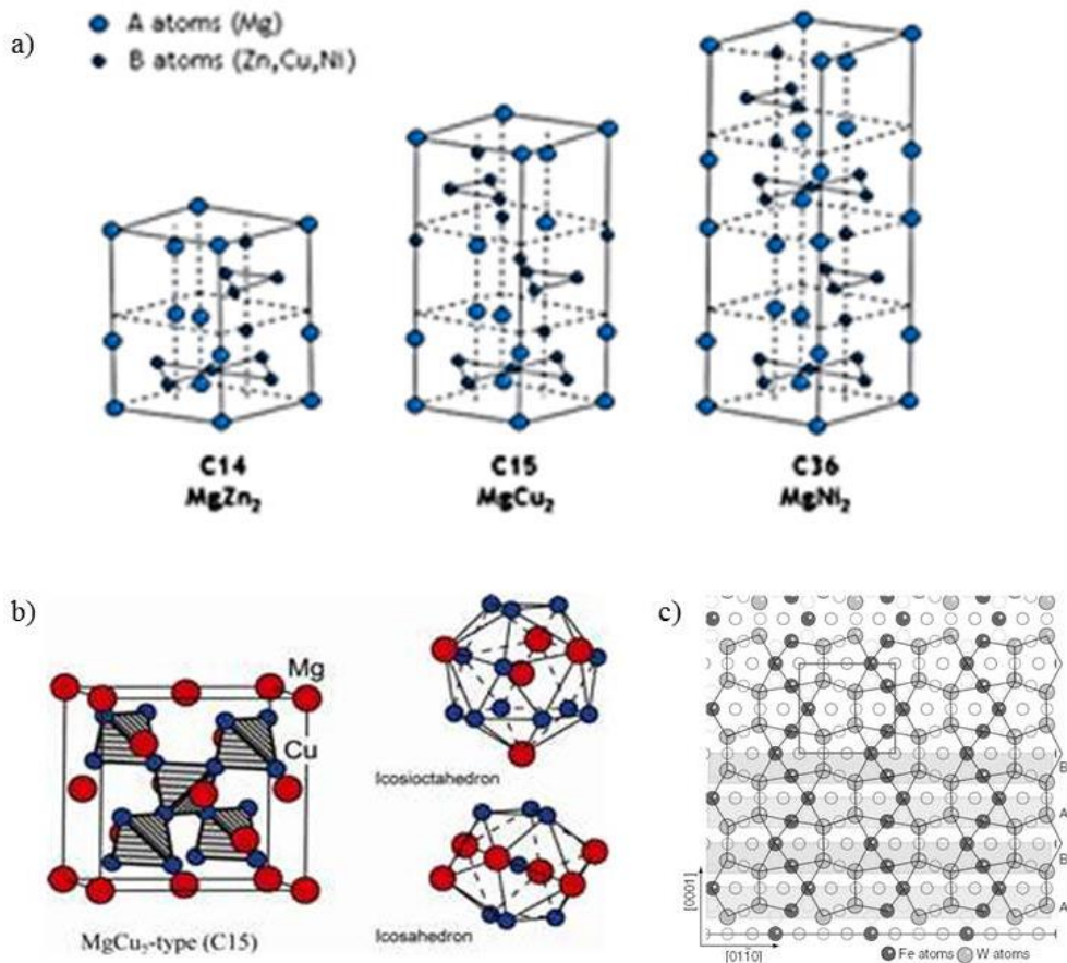
Figure 1. 2 : Phases de Laves et motifs icosaoédriques. a) empilement des atomes dans les phases de Laves (C14, C15, C36). b) Phase de Laves C15 et ses différents ordres locaux : un icosaèdre et un polyèdre dérivé de l'icosaèdre. c) Phase de Laves C14 : projection dans la direction [11-20] montrant des motifs pentagonaux [6].
