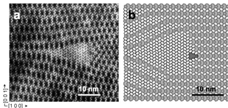
Figure 1.8: Méta-dislocation de la phase \epsilon -AlPdMn ; a) image HRTEM de la méta-dislocation ; b) schéma de la réorganisation au cœur du défaut [17].
