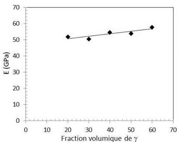
Figure 3.20: Modules de Young des composites mesurés par une méthode d'ultrasons en fonction de la fraction volumique de la phase \gamma -Mg 17 Al 12 .
