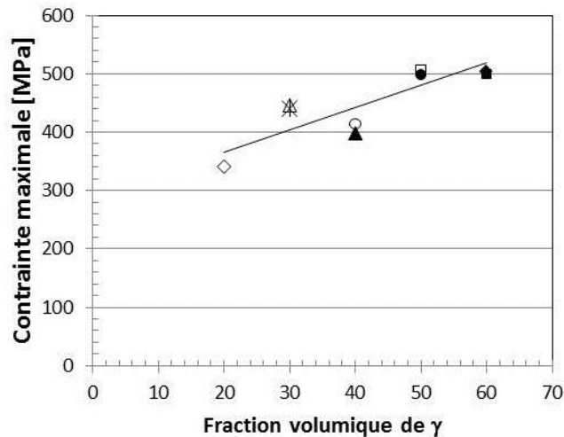
Figure 4.2: Evolution de la contrainte maximale ou de la contrainte à rupture (pour les échantillons fragiles) en fonction de la fraction volumique de la phase \gamma -Mg 17 Al 12 (les points correspondent à différents essais de compression).
