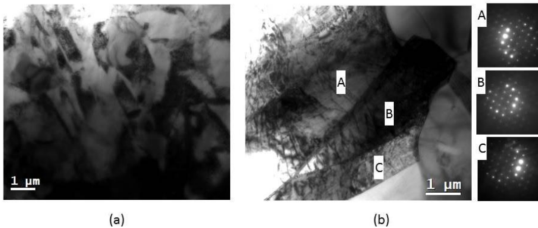
Figure B.10 : Microstructures dans les dendrites de Mg des échantillons extrudés ( T=350^{\circ}\text{C} , V=0.9\text{ mm/min} ), déformés à l'ambiante (Images MET en champ clair). a) dislocations et macles ( 0.5\text{-}1\text{ }\mu\text{m} ) dans différents plans (échantillon: Mg- \gamma 30%) ; b) grains Mg désorientés les uns par rapport aux autres d'après les diagrammes de diffraction: recristallisation des dendrites (échantillon Mg- \gamma 40%).
