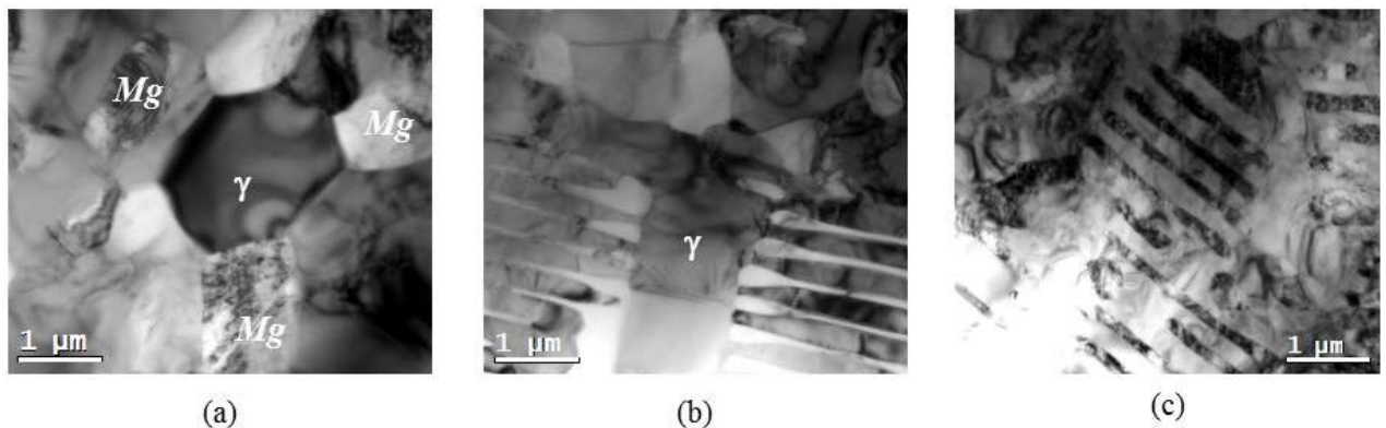
Figure B.3 : Microstructure d'un échantillon Mg- \gamma 60% après extrusion à 350°C – V=0.9 mm/min- rapport d'extrusion 5:1 (image MET en champ clair) : a) dans les zones eutectiques complètement coalescées, grains \gamma -Mg 17 Al 12 facettés et sans dislocation, grains Mg approximativement facettés avec dislocation. b) et c) dans les anciennes zones eutectiques peu coalescées, début de coalescence de la phase \gamma -Mg 17 Al 12 (1 \mu m) perpendiculairement aux fibres Mg; formation des paquets de fibres Mg non coalescées avec contrastes de dislocation.
