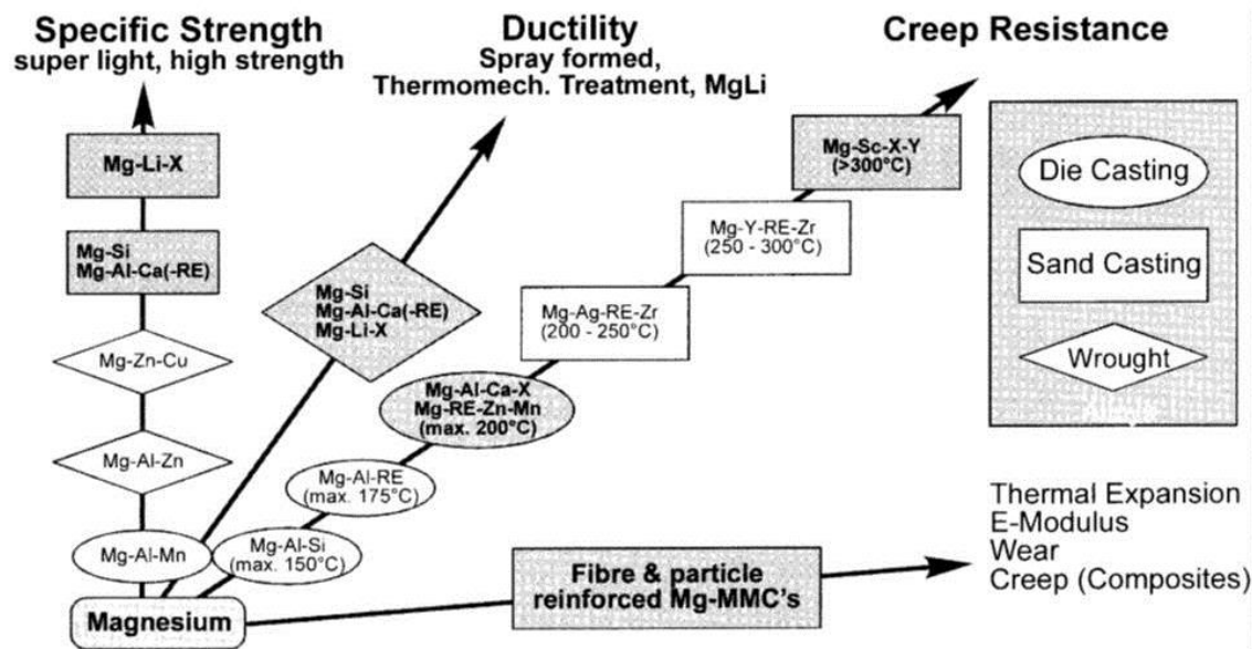
Figure 2.1: Possibles directions de développement des alliages et composites de Mg pour améliorer leurs performances [84]. Les principaux alliages commerciaux de magnésium sont des alliages Mg-Al-Zn (séries AZ), Mg-Al-Mn (série AM), Mg-Al-RE (série AE), Mg-RE-Zn (série EZ), Mg-Zn-Zr (série ZK), et Mg-RE-Zr (série WE).
