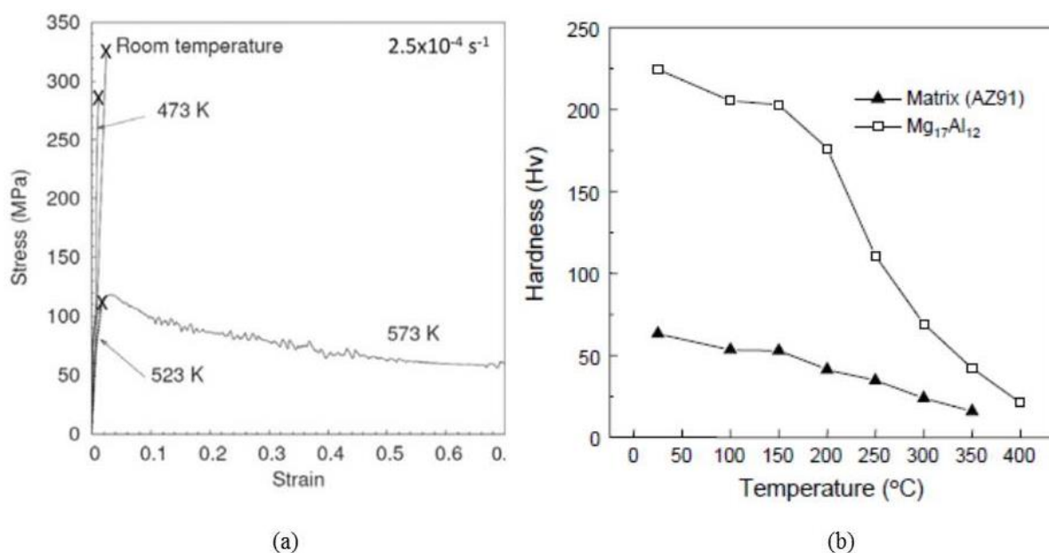
Figure 2.7 : Comportement mécanique à chaud de la phase \gamma -Mg 17 Al 12 ; a) test de compression [114] ; b) test de microdureté [115].
