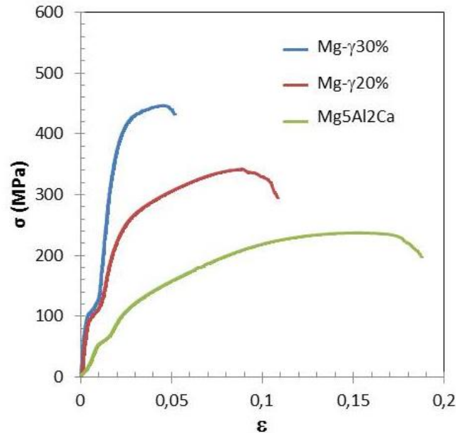
Figure 4.3: Courbes de compression à température ambiante des composites Mg- \gamma 30% et Mg- \gamma 20% et d'un alliage Mg5Al2Ca (Mg5wt%Al2wt%)- vitesse déformation 2.5 \cdot 10^{-4} \text{ s}^{-1} .
