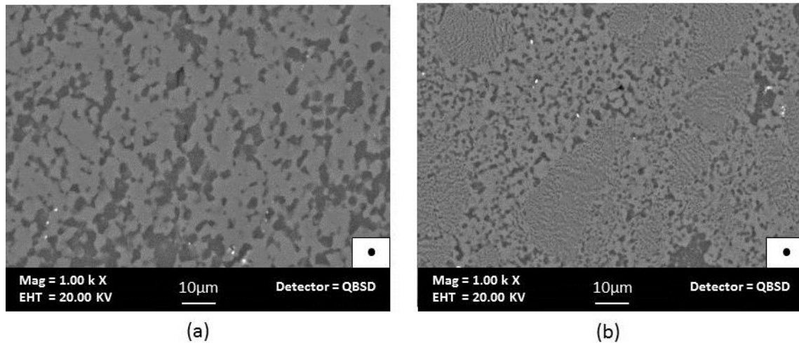
Figure B.15: Microstructures des échantillons déformés ( T=300^{\circ}\text{C} , t=1\text{h } 30\text{ min} , \varepsilon=1 , Vitesse de déformation =2.5 \cdot 10^{-4}\text{ s}^{-1} ) du composite extrudé Mg- \gamma 60% ( T=350^{\circ}\text{C} , V=0.9\text{ mm/min} ) vue dans une section perpendiculaire à la direction de déformation. a) Microstructure d'un échantillon prélevé en haut : un mélange des grains Mg et \gamma\text{-Mg}_{17}\text{Al}_{12} (3-10 \mu\text{m} ). b) Microstructure d'un échantillon prélevé en bas : reste des dendrites morcelées par précipitation de \gamma\text{-Mg}_{17}\text{Al}_{12} , des bandes de particules \gamma\text{-Mg}_{17}\text{Al}_{12} et Mg (3-5 \mu\text{m} ), et des anciennes zones eutectiques peu coalescées.
