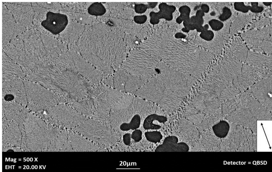
Figure 5.14: Microstructure d'un échantillon Mg- \gamma 50% déformé à 300^\circ\text{C} ( \varepsilon = 0.3 ; t = 35 \text{ min} ) (image MEB en électrons rétrodiffusés) – direction de déformation (indiquée en insert) dans le plan de la section: observation de bandes des particules Mg et \gamma\text{-Mg}_{17}\text{Al}_{12} selon deux directions perpendiculaires et à \sim 45^\circ de la direction de déformation.
