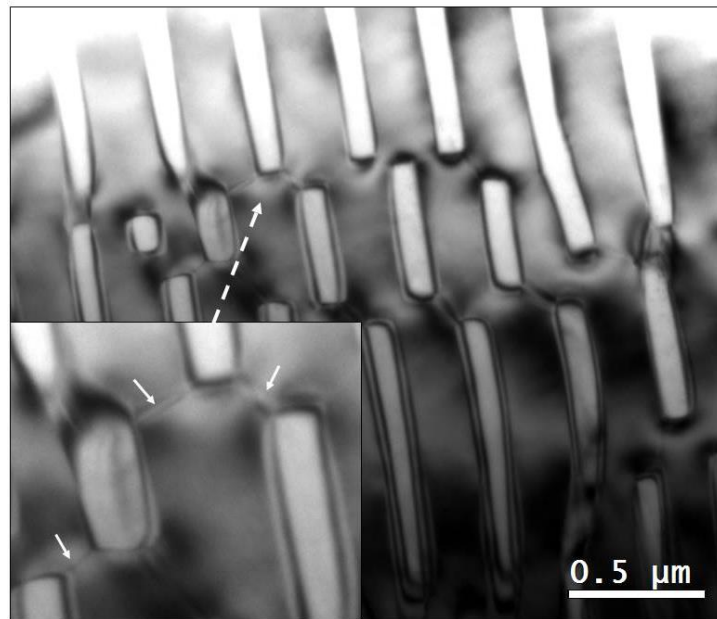
Figure 4.7: Microstructure observée dans les zones eutectiques d'un échantillon déformé à l'ambiante (Image MET en champ clair). Zone eutectique en vue selon un axe de zone perpendiculaire aux fibres Mg dans une zone présentant un défaut d'arrangement : des traces de dislocations sont observées dans les segments joignant les fibres Mg (échantillon: Mg- \gamma 60%).
