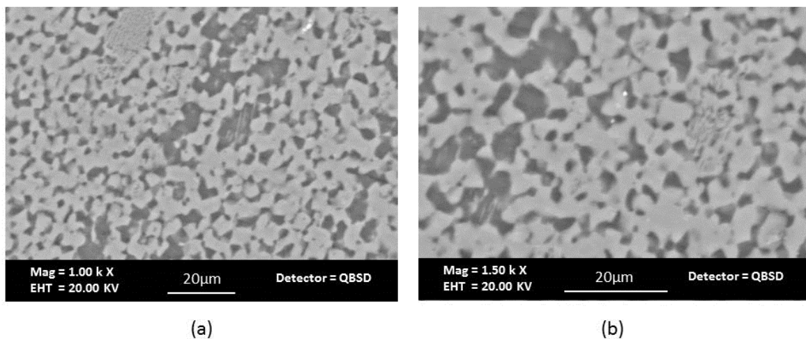
Figure B.18 : Microstructures d'un échantillon déformé ( T=300^{\circ}\text{C} , t= 1\text{h } 30\text{ min} , \varepsilon=1 , Vitesse de déformation =2.5 \cdot 10^{-4} \text{ s}^{-1} ) du composite préalablement déformé à 300^{\circ}\text{C} Mg- \gamma 60%. Vue dans une section parallèle à la direction de déformation : microstructure homogène consiste d'un mélange de grains Mg et \gamma -Mg 17 Al 12 de taille entre 3 et 10 \mu\text{m} issus soit des zones eutectiques soit des zones dendritiques.
