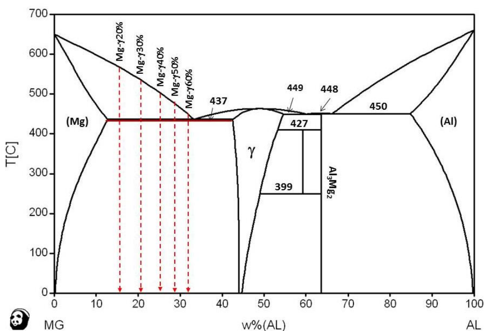
Figure 3.2 : Diagramme de phases du système Mg-Al, calculé à l'aide du logiciel Pandat et de la base de données PanMg8 [105], les flèches en pointillé indiquent la composition initiale en Al des composites Mg/ \gamma -Mg 17 Al 12 visés.
