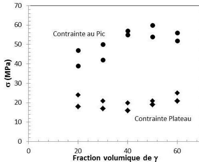
Figure 5.4: Contraintes au pic et contraintes plateau en fonction de la fraction volumique de la phase \gamma -Mg 17 Al 12 . Pour chaque composition, deux essais de compression (à 300°C) ont été réalisés – vitesse de déformation: 2.5 \cdot 10^{-4} \text{ s}^{-1}
