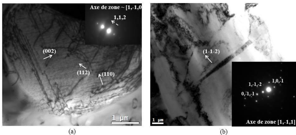
Figure 4.5: Microstructures dans les dendrites de Mg d'un échantillon déformé à l'ambiante (Images MET en champ clair). a) Dislocations dans le plan de base et les plans pyramidaux et prismatiques (échantillon: Mg-γ60%) ; b) Macle fine (épaisseur : 0.1 à 0.5 μm) dans un plan pyramidal (échantillon: Mg-γ40%).
