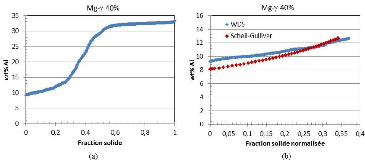
Figure 3.7 : a) Profil expérimental de la composition en fonction de la fraction solide obtenue par analyse WDS d'une grille de 400 points d'analyses avec un pas entre les points de 20 \mu m. b) Micro-ségrégation dans les dendrites de (Mg) comparée avec les prédictions issues du modèle de Scheil-Gulliver (échantillon Mg- \gamma 40%).
