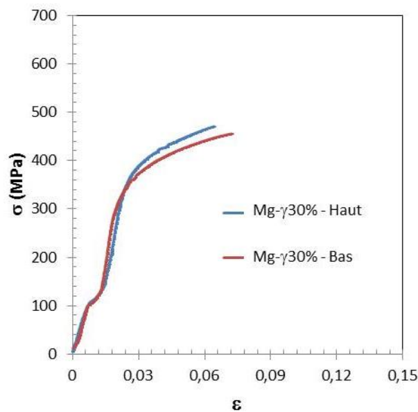
Figure B.8: Courbes contrainte – déformation à température ambiante du composite Mg- \gamma 30% en haut et en bas - vitesse de déformation: 2.5 \cdot 10^{-4} \text{ s}^{-1} ;
