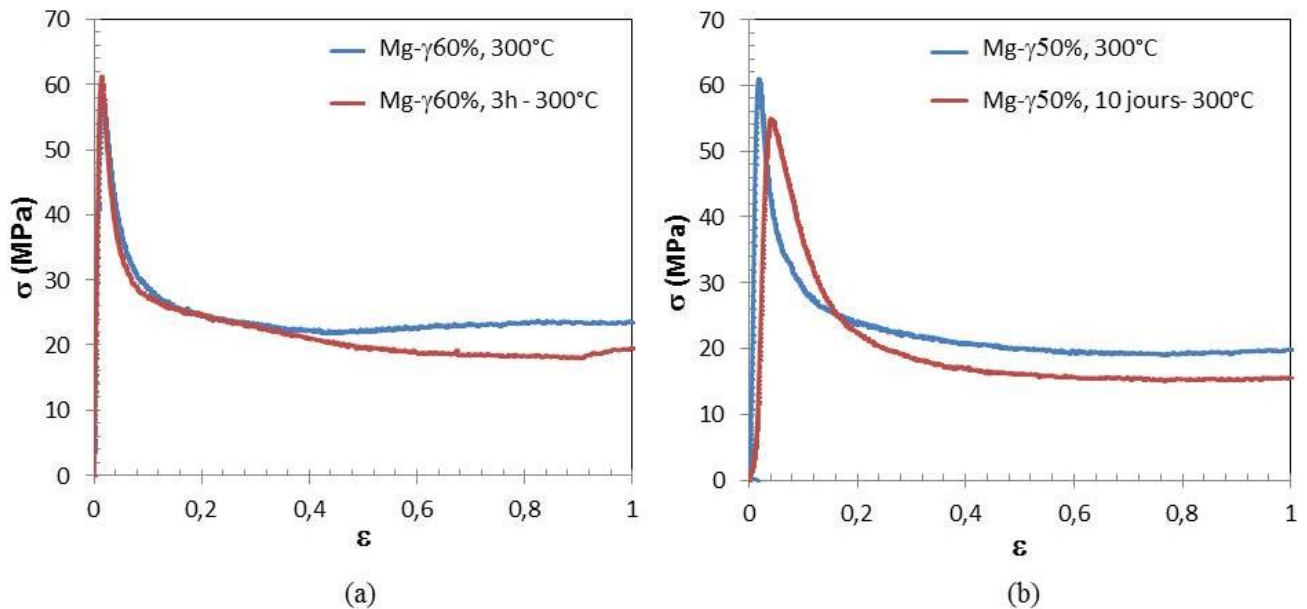
Figure 5.20: Comparaison des courbes contrainte-déformation à 300°C - 2.5 \cdot 10^{-4} \text{ s}^{-1} de composites à l'état brut d'élaboration et recuits à 300°C. a) Mg- \gamma 60%: recuit 3h. b) Mg- \gamma 50%: recuit 10 jours.
