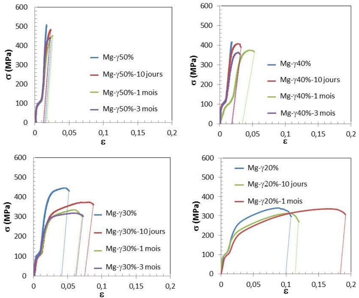
Figure 4.10: Courbes contrainte-déformation à température ambiante de composites Mg- \gamma 50%, Mg- \gamma 40%, Mg- \gamma 30%, Mg- \gamma 20% à l'état brut d'élaboration et après recuits à 300°C (10 jours, 1 mois, 3 mois)- vitesse de déformation: 2.5 \cdot 10^{-4} \text{ s}^{-1} .
