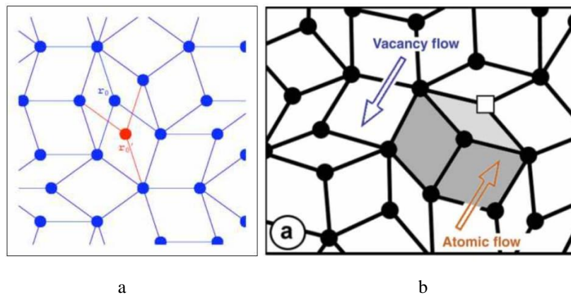
Figure 1.7: a) Défaut de Phason et réorganisation locale possible. b) Diffusion des lacunes assistées par des phasons [27], [28].
