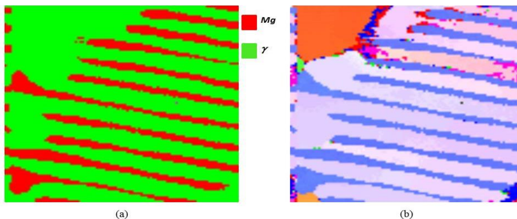
Figure 3.13 : Zone eutectique imagée en microscopie en transmission à l'aide de l'outil ACOM. a) Cartographie de phase : en rouge phase (Mg), en vert phase \gamma -Mg 17 Al 12 . b) Cartographie orientation montrant l'existence d'une même relation d'orientation sur toute la zone.
