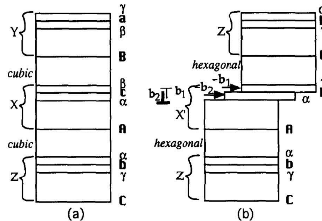
Figure 1.6: Schéma des empilements et transformation des phases par « Synchro-shear » [21].
