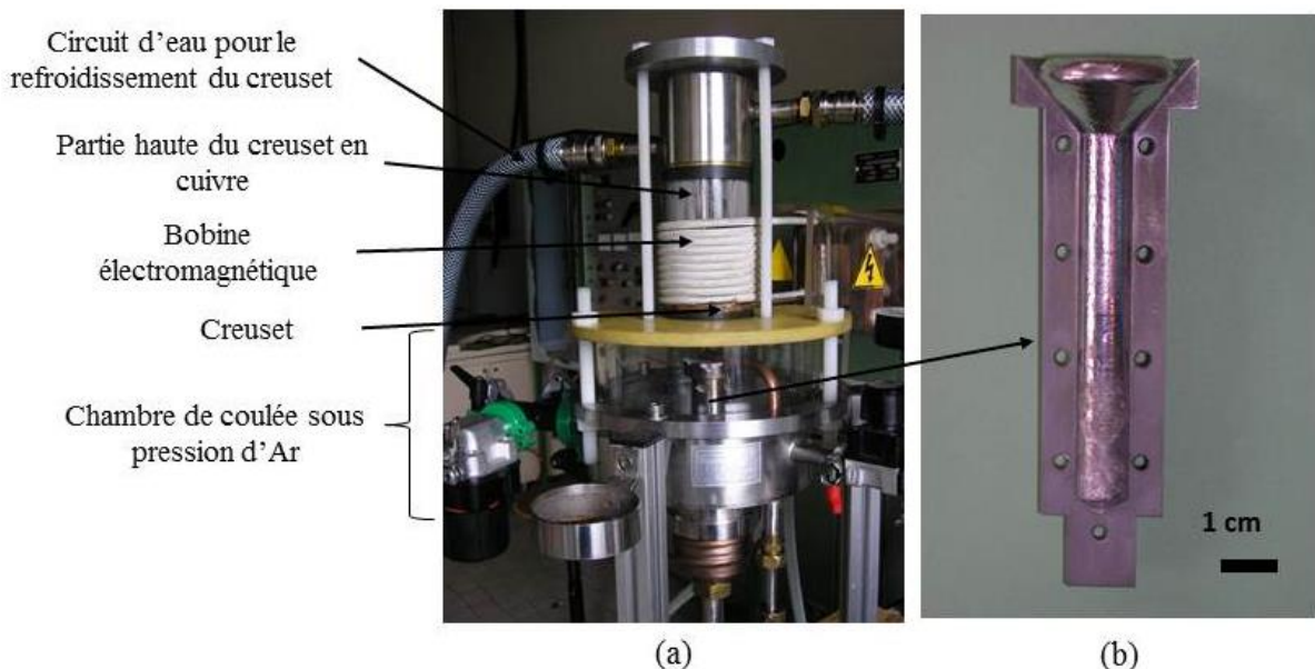
Figure 3.5 : a) Dispositif du creuset froid inductif, SIMAP; b) Lingotière en acier inoxydable ferritique contenant le lingot d'un composite Mg/ \gamma -Mg 17 Al 12 .
