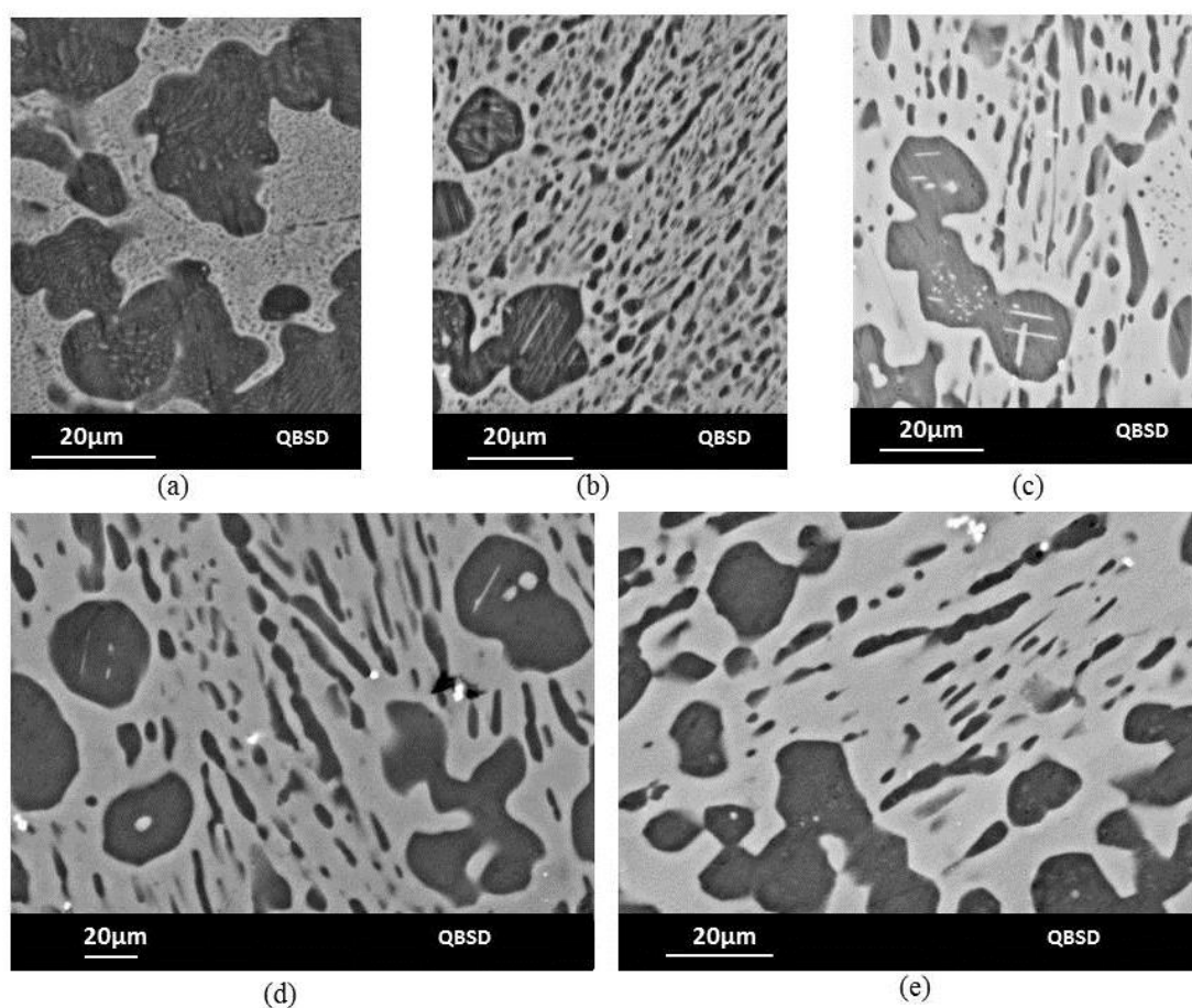
Figure 3.17: Microstructure d'échantillons Mg- \gamma 50% traités à 300°C; a) recuit 1h30 ; b) recuit 10 jours ; c) recuit 1 mois ; d) recuit 3 mois ; e) recuit 5 mois.
