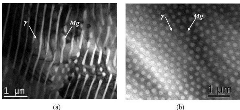
Figure 3.11 : Microstructure des cellules eutectiques (image MET champ clair): a) Vue selon un axe de zone perpendiculaire à l'axe des fibres (Mg). b) Vue selon un axe de zone parallèle à l'axe des fibres (Mg) : la phase \gamma -Mg 17 Al 12 (contraste sombre) est la matrice, les fibres Mg (contraste clair); les fibres (Mg) sont de diamètre 0.2 \mu\text{m} , la distance inter-fibre est de 0.4 \mu\text{m}
