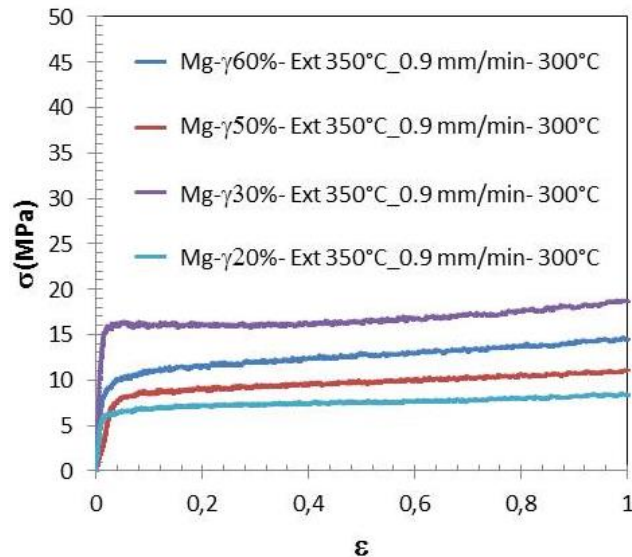
Figure B.14 : Courbes contrainte-déformation de composites Mg- \gamma 60%, Mg- \gamma 50%, Mg- \gamma 30%, Mg- \gamma 20% extrudés ( T=350^{\circ}\text{C} , V=0.9\text{ mm/min} ) déformés à 300^{\circ}\text{C} –vitesse de déformation 2.5\ 10^{-4}\text{ s}^{-1} .
