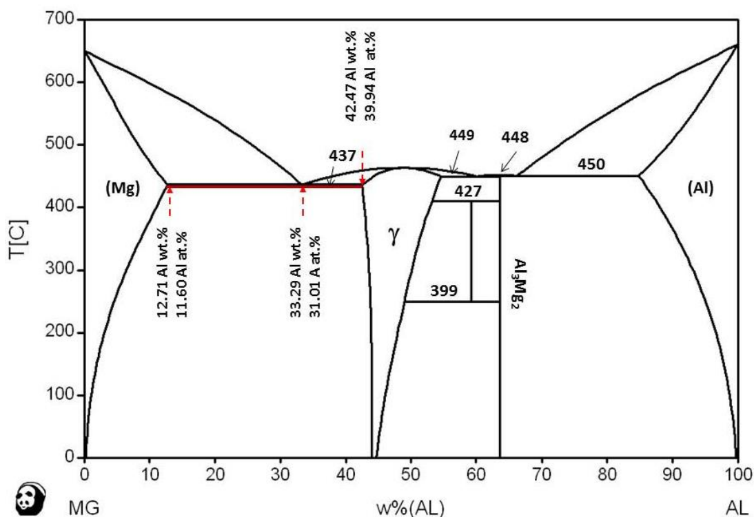
Figure 2.4 : Diagramme des phases Mg-Al calculé avec le logiciel Pandat à partir de la base des données thermodynamique PanMg8.
