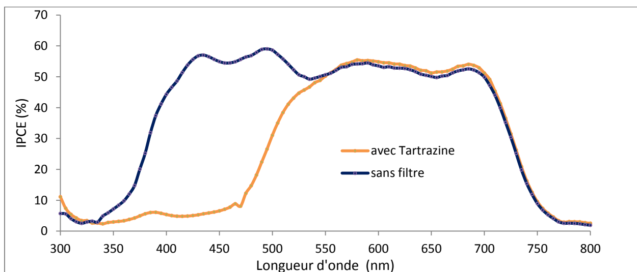
Figure 3.4.5 : IPCE du dispositif avec et sans filtre
