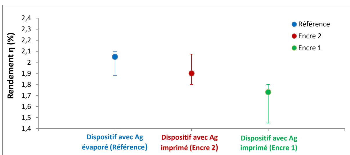
Figure 2.5.3 : Comparaison des performances de dispositifs à base d'ETL 1 pour différentes électrodes supérieures
