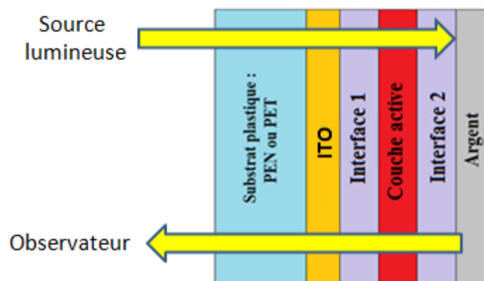
Figure 2.2.1 : Perception de la couleur d'une cellule
