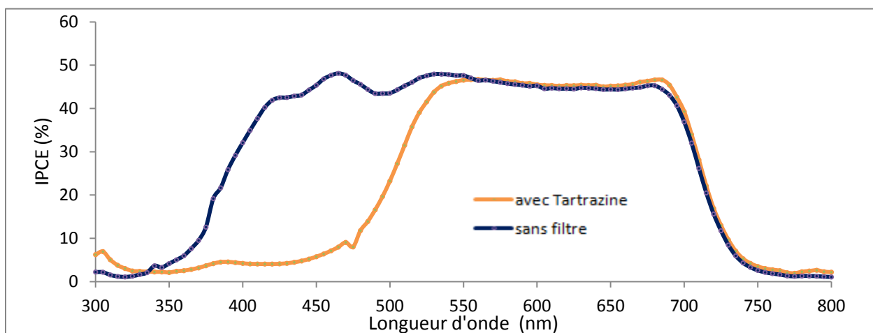
Figure 3.4.9 : Performances et IPCE du dispositif à base d'OPV 1:PC 60 BM avec et sans tartrazine
