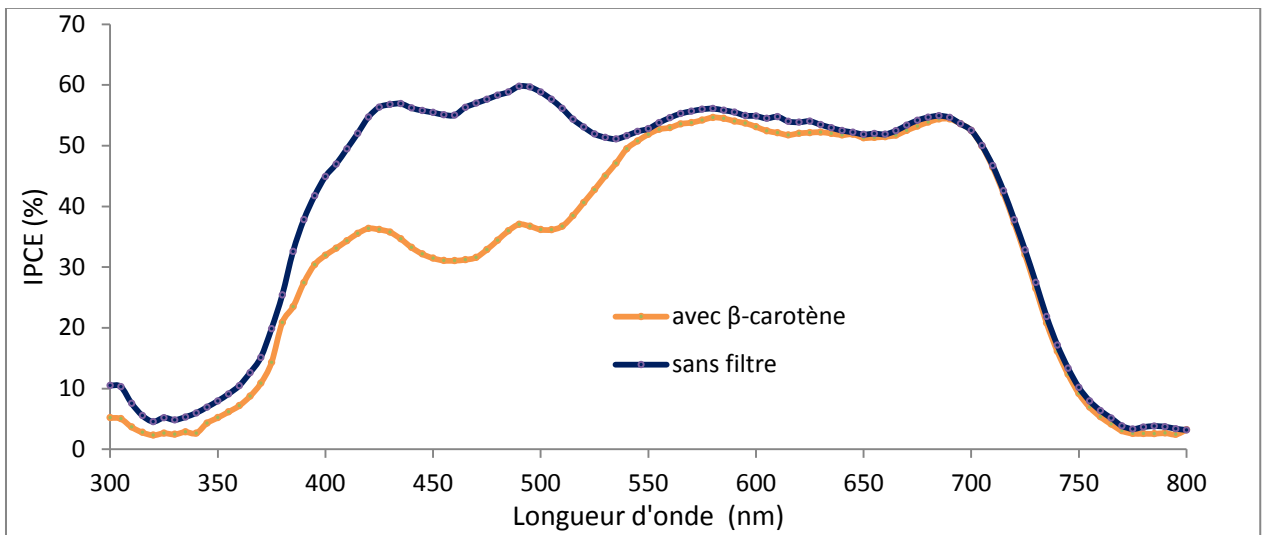
Figure 3.4.2 : IPCE du dispositif avec et sans filtre
