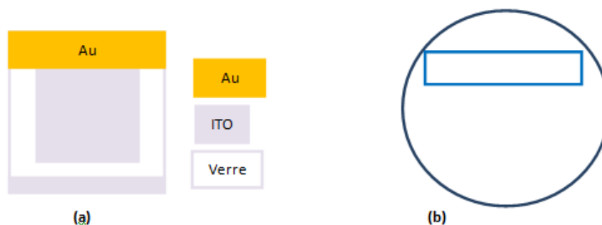
Figure 3 : (a) Schéma de dépôt de la bande d'or d'une épaisseur de 60 nm sur substrat gravé d'ITO
