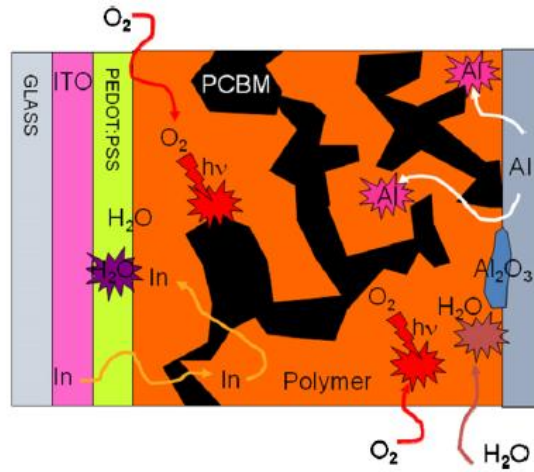
Figure 4.1.7 : Vue transversale schématique d'une cellule solaire en structure standard présentant les mécanismes de dégradation répertoriés précédemment [68]
