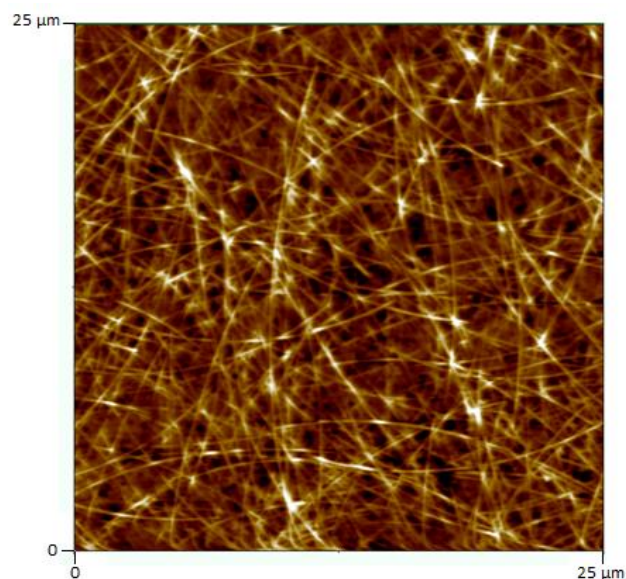
Figure 3.3.10 : Cartographie AFM d'un film de nanofils d'argent d'épaisseur moyenne de 90 nm
