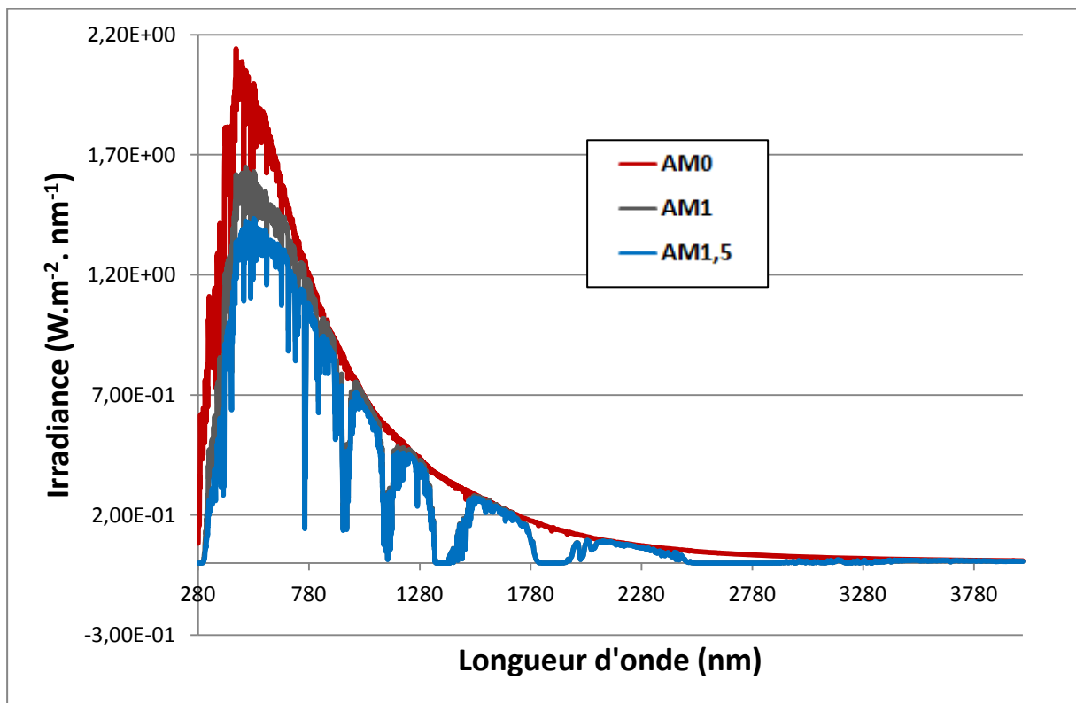
Figure 3.1.2 : Distribution spectrale des conditions AM0, AM1 et AM1.5
