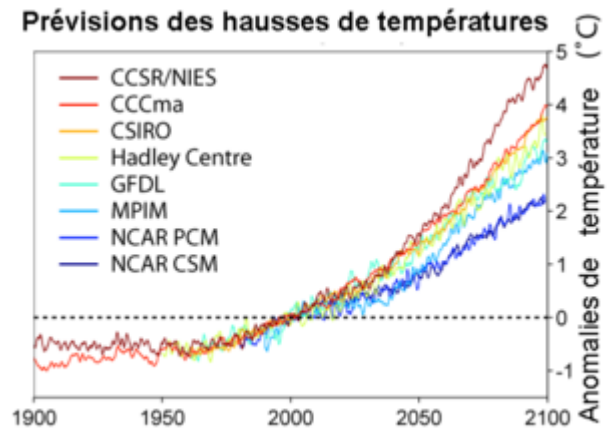
Figure 1.1.5 : Prévion sur le réchauffement climatique [5]
