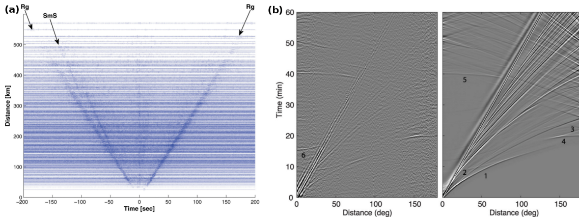
FIGURE 1.10 – Émergence des ondes de volume dans la corrélation de bruit. (a) Corrélations des composantes verticales filtrées entre 0.5 et 1 H_z . Rg : Onde de Rayleigh. SmS : Ondes S réfléchies sur le Moho. D’après Poli et al. (2012b). (b) À gauche : Inter-corrélations entre 339 stations réparties sur la totalité du globe (57 000 paires de stations) en fonction de la distance épacentrale filtrées entre 25 et 100 s . L’onde S réfléchi sur le noyau ( ScS ) est noté 6. À droite : Sismogrammes synthétiques générés dans le modèle PREM. 1 : P directe ; 2 : PcP ; 3 : PKP ; 4 : PKIKP ; 5 : PKIKP plus PKIKP soit P'P' l’onde P réfléchi à la surface. D’après Boué et al. (2013).
