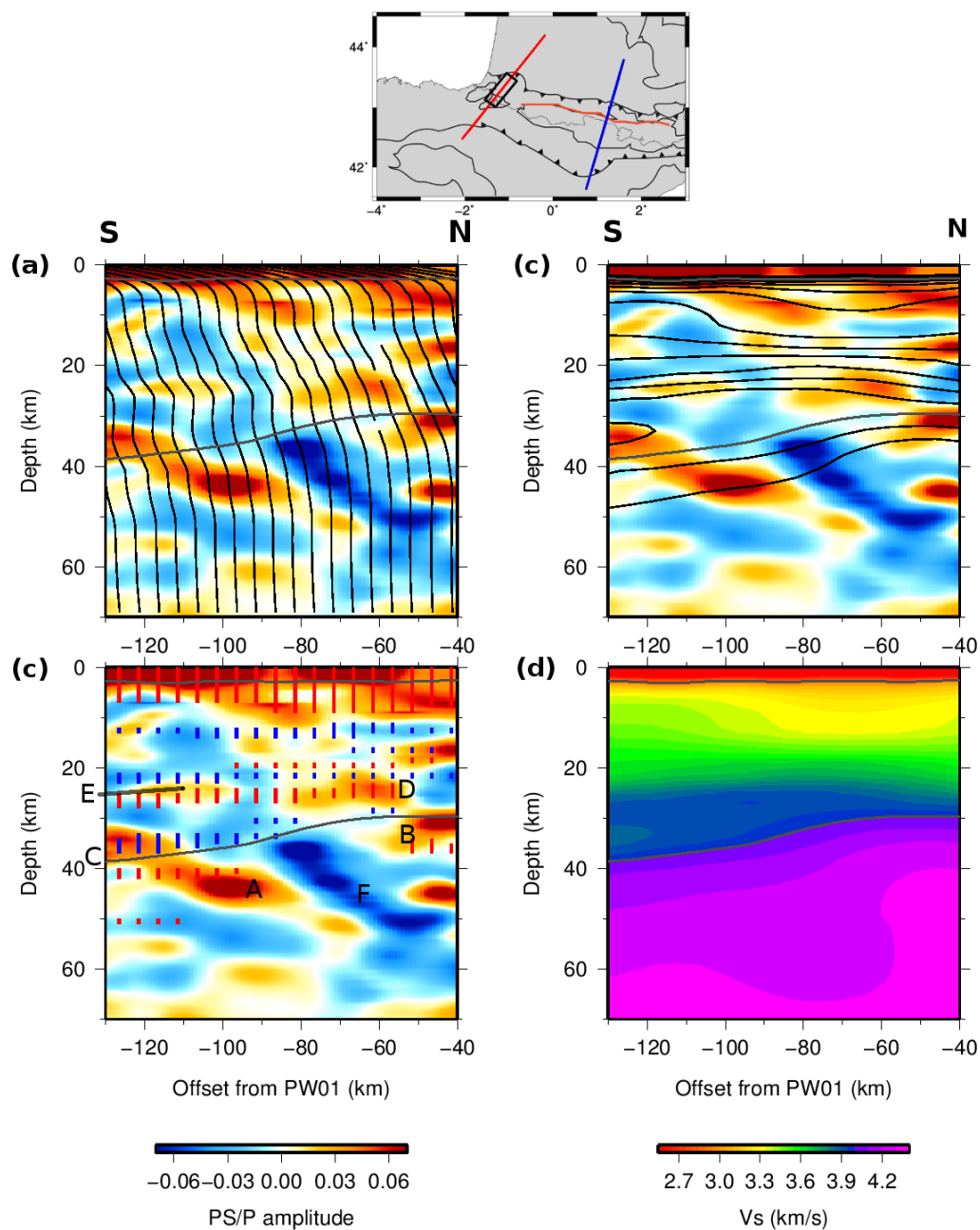
FIGURE 3.14 – Région du Labourd-Mauléon (profil Ouest, voir localisation Figure 3.10). Voir légende de la Figure 3.11.
