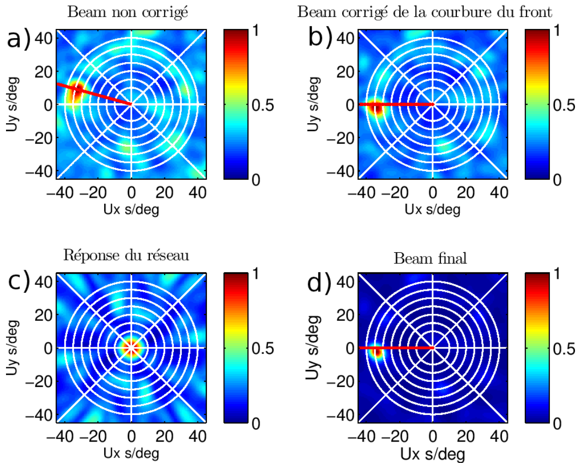
FIGURE 4.7 – Différentes corrections appliquées au résultat du beamforming. E146 est la source, E920 la station centre du réseau. Les corrélations sont filtrées entre 15 et 18s. (a) Beam sans correction. (b) Beam corrigé de la courbure du front. (c) Réponse du sous-réseau. (d) Beam final, corrigé de la courbure du front et déconvolué de la réponse du réseau. La ligne rouge est l’azimut le long du grand cercle entre la station source et la station centre du sous-réseau. Les résultats du beam sont normalisés.
