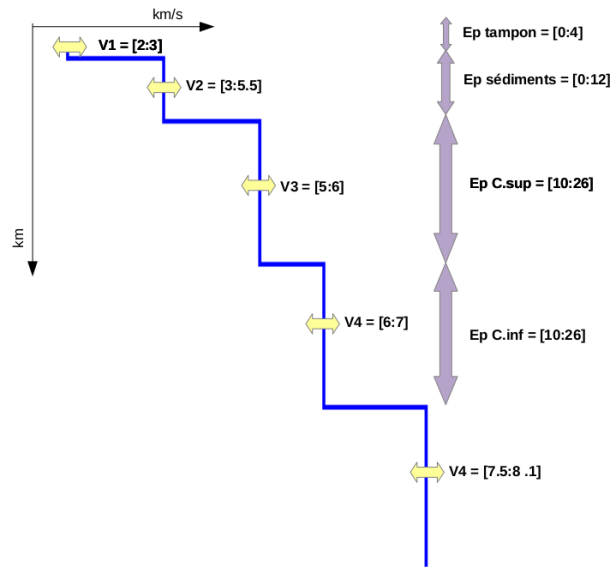
FIGURE 3.1 – Gammes de variation des paramètres de chaque couche utilisées pour la construction de la bibliothèque de modèles initiaux. Le pas de variation des vitesses est de 0.5\ km.s^{-1} , excepté pour le manteau où il est de 0.2\ km.s^{-1} . Le pas de variation des épaisseurs est de 1\ km pour la couche tampon et la couche sédimentaire, et de 2\ km pour les croûtes supérieure et inférieure.
