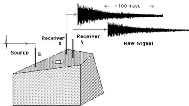
Figure 15 : Une source impulsionnelle crée un champ diffus de longue durée qui est détecté aux récepteurs x et y. Après une compensation de l'absorption, la corrélation entre les signaux détectés est comparée à une autre forme d'onde : celle qui est détectée en y lorsque x émet un pulse. D'après Weaver and Lobkis 2002.
