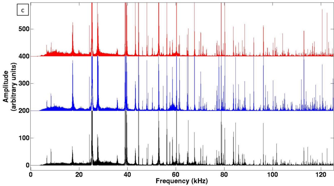
Figure 33: Trois spectres correspondant à trois sommations différentes de (a) 5, (b) 10, (c) 15 corrélations différentes. Un filtre passe-haut (5kHz) est appliqué à chaque paire de signaux avant qu'ils soient corrélés ensemble. Le lot de corrélations choisies pour être sommées ensemble est totalement différent d'une sous figure à l'autre.
