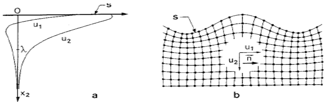
Figure 5 : onde de Rayleigh dans un milieu isotrope semi-infini. Vecteur s : sens de propagation. a) décroissance de la composante longitudinale u_1 et de la composante transversale u_2 en fonction de la profondeur. b) déformation de la surface. (modifié d'après Royer-Dieulesaint 1996)
