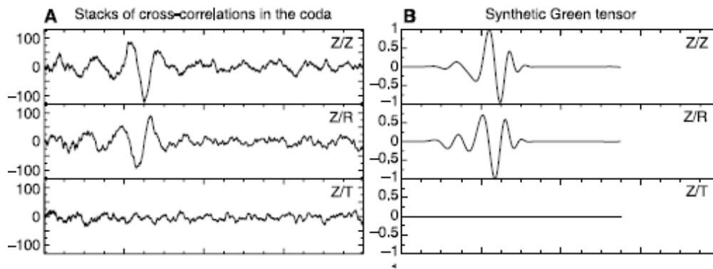
Figure 16 : Comparaison entre stacks de corrélations d'enregistrements aux stations PLIG et YAIG (A) et composantes du tenseur de Green théorique (B), calculé pour des distances entre station et source de 69 km. Ici il s'agit des corrélations entre la composante verticale Z et, de haut en bas : elle-même, la composante radiale R, la composante toroïdale T. (modifié d'après Campillo et Paul 2003).
