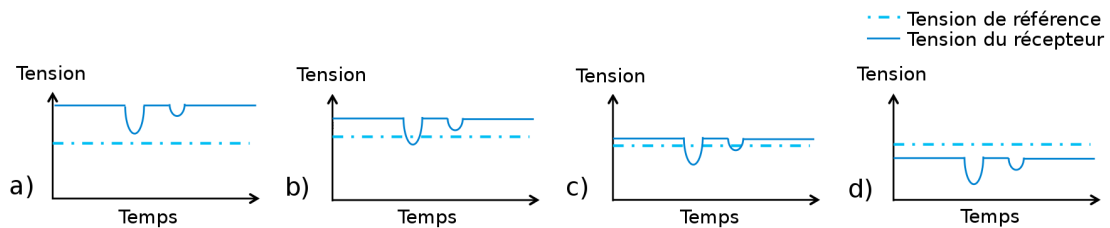
FIGURE 3.20 – Mode de fonctionnement des fourches optiques Wenglor. a) La tension du récepteur photoélectrique est trop éloignée de la tension de référence, le capteur ne détecte aucune particule. b) La tension du récepteur est suffisamment proche de la tension de référence pour détecter la grosse particule, mais pas la petite. c) Le capteur détecte les deux particules. d) La tension du récepteur est toujours inférieure à la tension de référence, le capteur ne fonctionne plus. Source : Vocanson (2014).
