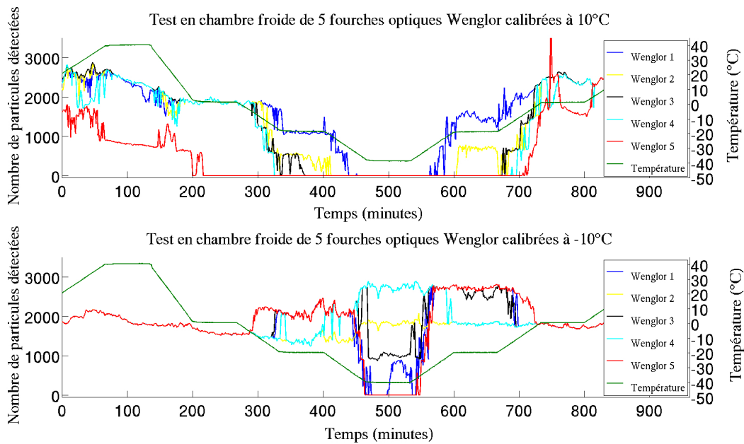
FIGURE 3.21 – Test de 5 fourches optiques Wenglor étalonnées à des températures différentes : 10 ° C pour le graphe du haut, et -10 ° C pour le graphe du bas. Lors de ce test, nous avons installé trois fils de diamètres différents sur le moteur : 0,06 mm, 0,25 mm, et 0,57 mm.
