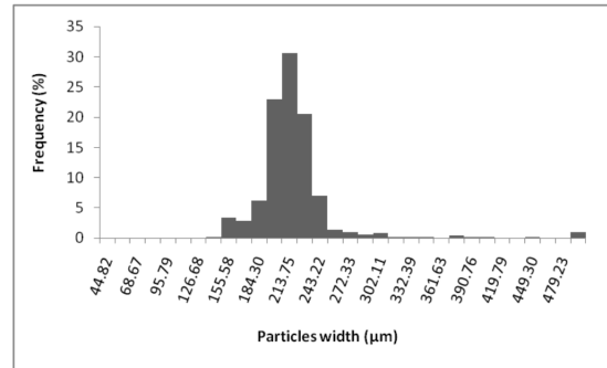
FIGURE 3.12 – Taille minimum des particules détectées par les fourches optiques Wenglor déterminée en comparant les mesures issues d'une fourche optique Wenglor aux mesures issues d'un Snow Particle Counter durant la période du 2 au 29 février 2012. La figure montre la fréquence de taille minimum de particule détectée par la fourche optique Wenglor, le calcul ayant été réalisé pour chaque pas de temps de 10 minutes. Les périodes avec une vitesse de vent inférieure à 6 \text{ m.s}^{-1} , et celles où le nombre de particules détectées par la fourche optique Wenglor était inférieur à 20 \text{ particules.cm}^{-2}.\text{min}^{-1} ont été exclues. Source : Naaim-Bouvet et al. (2014).
