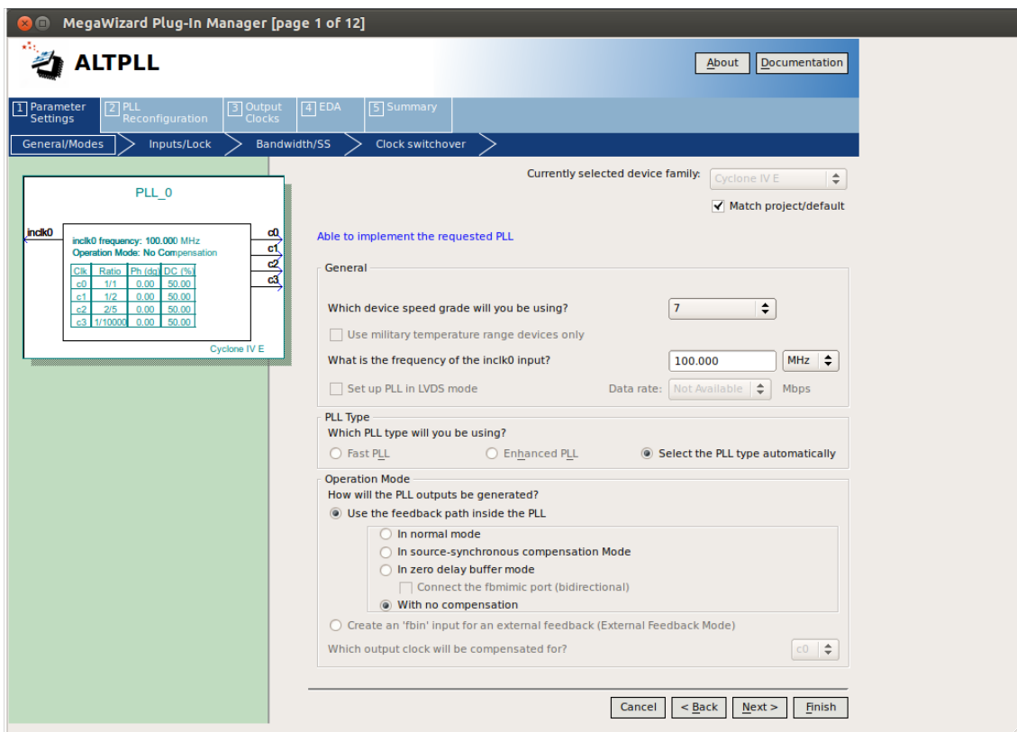
FIGURE C.18 – Capture d'écran de l'interface de configuration de la PLL.
