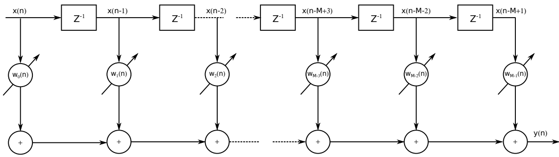
FIGURE 3.3 – Structure d'un filtre FIR (transversal) de M coefficients.
