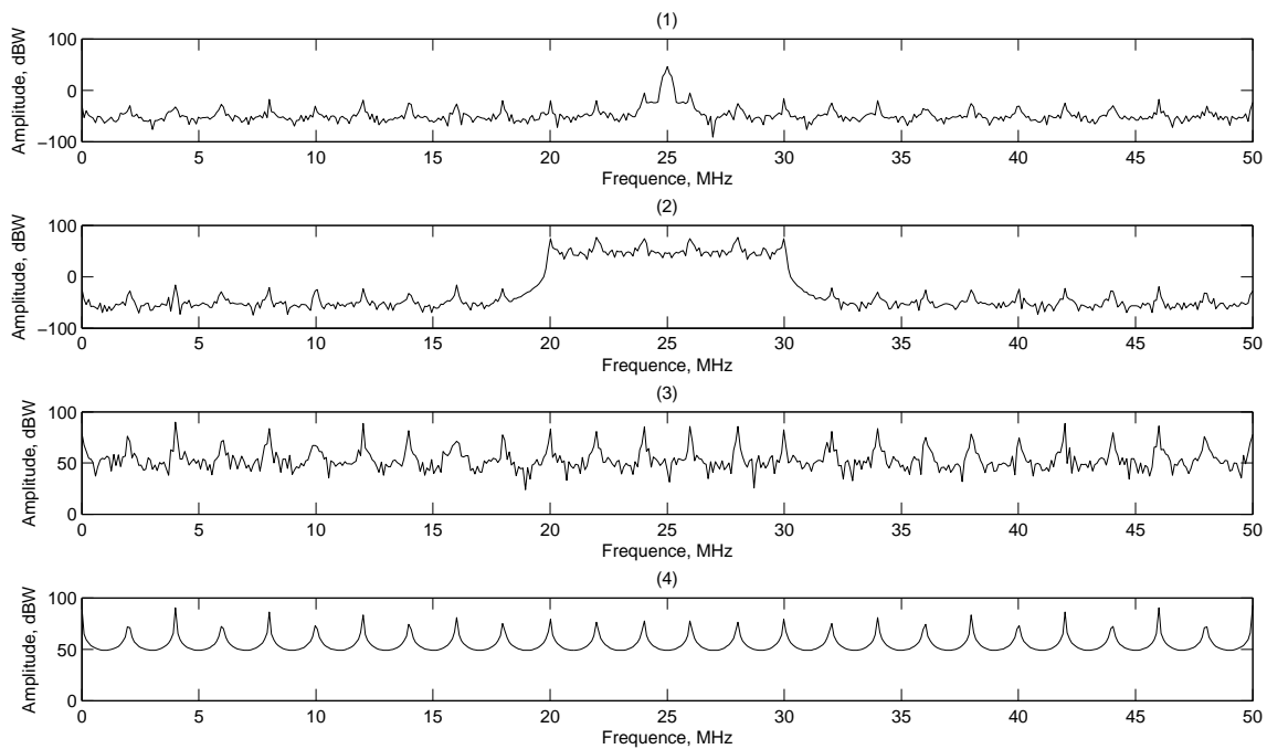
FIGURE 2.17 – Visualisation dans le domaine fréquentiel de l'impact d'un écho fort dans le cas d'un signal à bande étroite, large bande, bruit et tracking.
