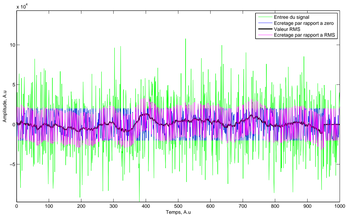
FIGURE 7.15 – Comparaison de l'écrêtage par rapport à zéro à l'écrêtage par rapport à la RMS.
