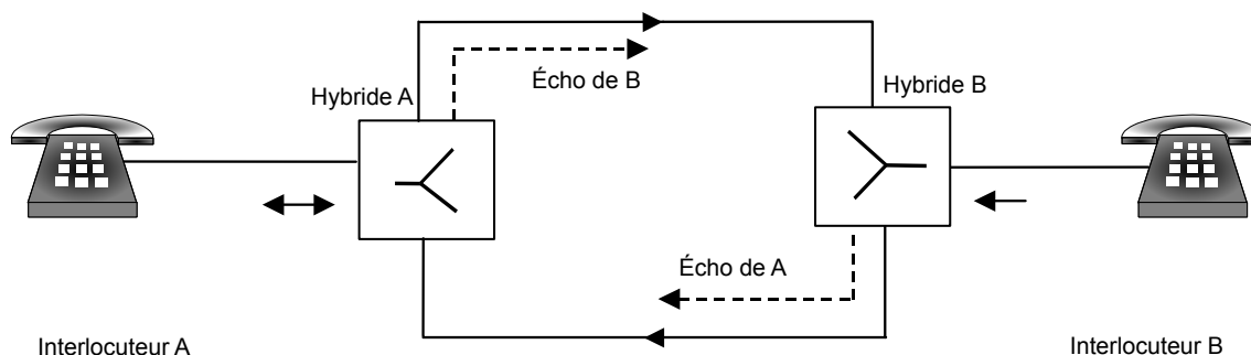
FIGURE 1.9 – Écho de ligne.
