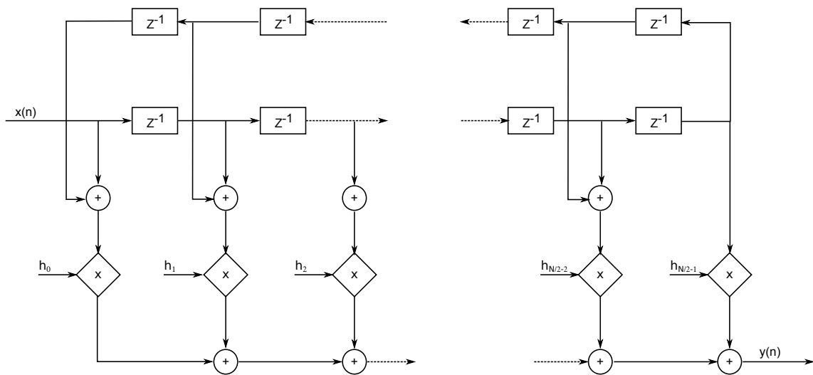
FIGURE C.12 – Structure symétrique d'une filtre FIR de d'ordre N_{\text{FIR}} .
