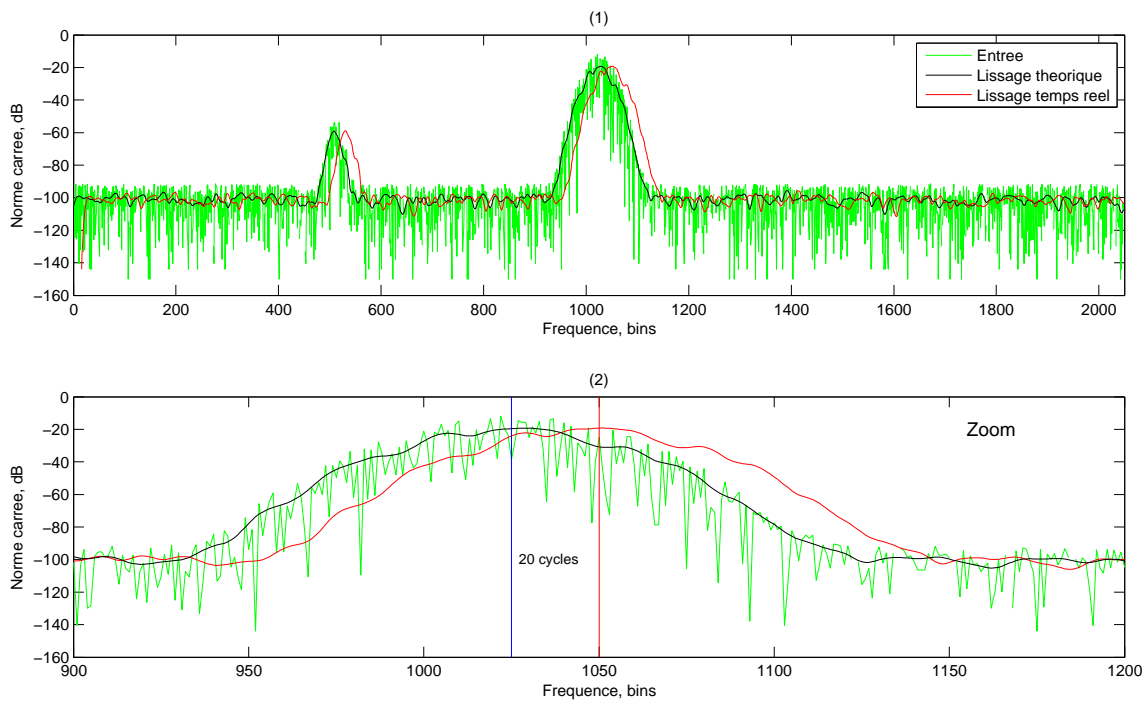
FIGURE 4.22 – Exemple de lissage en temps-réel, cascade de 5 filtres avec N_{MAV} = 5 .
