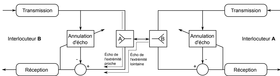
FIGURE 1.12 – Suppression des échos de ligne.
