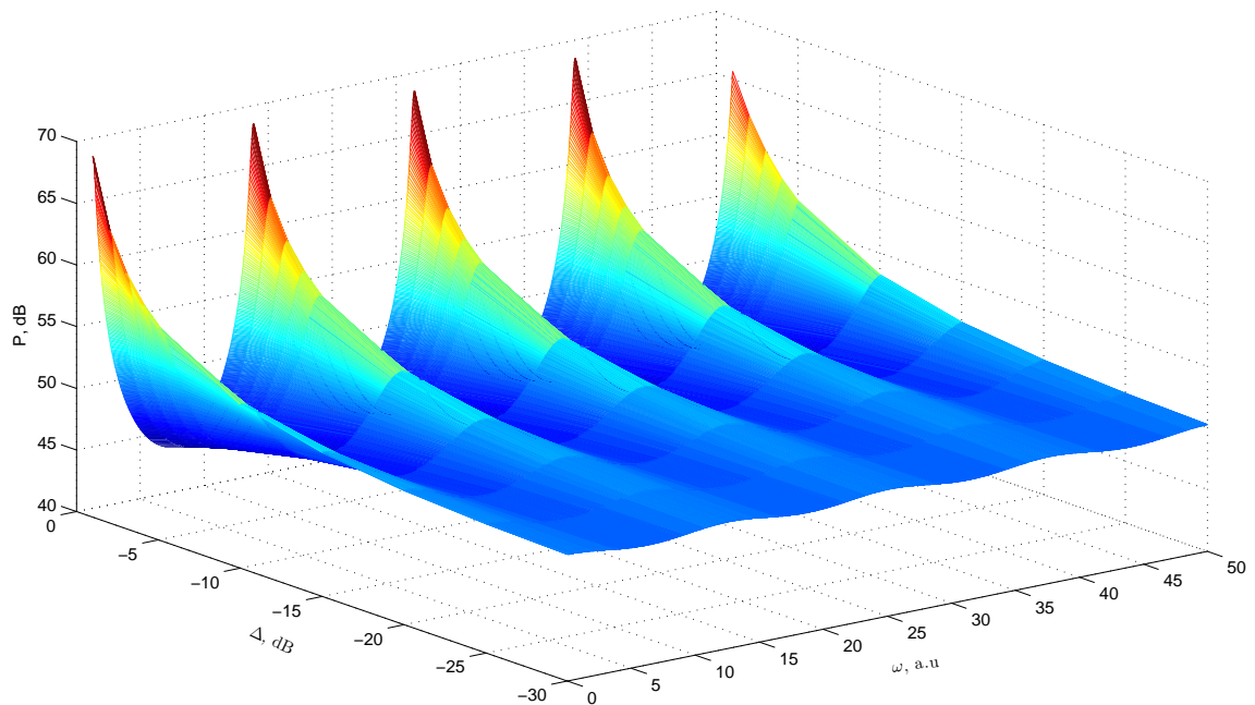
FIGURE 2.4 – Variations du gain de puissance dans le système en boucle-fermée dans le cas d'un écho direct.
