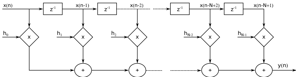
FIGURE C.11 – Structure directe d'une filtre FIR de d'ordre N_{FIR} .
