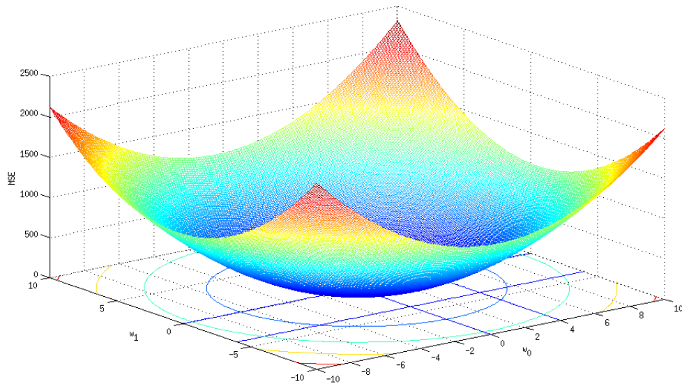
FIGURE 3.4 – Critère de performance MSE dans le cas d'un filtre FIR de deux coefficients.
