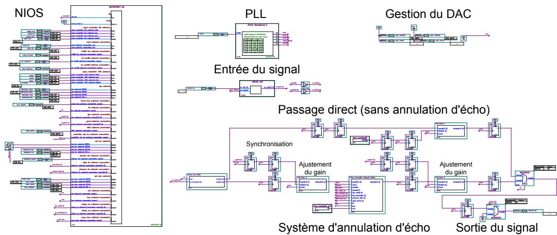
FIGURE C.21 – Schématique (top view) du système d'annulation d'écho.
