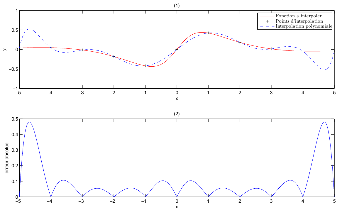
FIGURE A.2 – Exemple d'interpolation polynomiale (LAGRANGE) de la fonction f(x) = \frac{1}{1+x^2} \sin(x) , restreinte aux entiers de l'intervalle [-5, 5]
