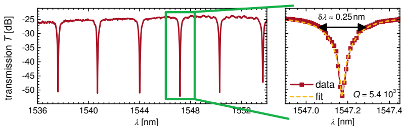
Fig. A.5 Spectre de transmission TM d'un résonateur circulaire à base de guides d'ondes composés comprenant du BaTiO 3 , étant couplé au point critique. Le facteur de qualite extrait de la resonance agrandie a droite est Q = 5.4 \times 10^3 . La largeur de la resonance a mi-transmission \delta\lambda (-3 dB) est indiquée dans la figure de droite.
