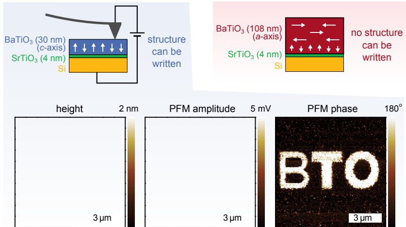
Fig. A.2 Haut : schémas de la structure des échantillons mesurés par PFM. Bas : topographie, amplitude et phase du signal PFM mesuré sur film mince de \text{BaTiO}_3 orienté selon l'axe c après écriture des lettres "BTO". Aucun contraste du signal PFM n'est observable sur le film plus épais orienté selon l'axe a .
