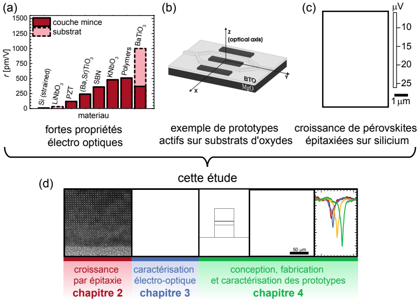
Fig. A.1 (a) Comparaison des coefficients de Pockels de différents matériaux (d'après les [26–28]), le BaTiO 3 épais présente la plus forte valeur. (b) Exemple de modulateur optique à base de BaTiO 3 déposé sur substrat de MgO [29] (schéma reporté avec la permission d'AIP Publishing LLC). (c) Croissance épitaxiée de SrTiO 3 ferroélectrique sur silicium [30] (schéma reporté avec la permission de l'association américaine pour l'avancée de la science). (d) Sujet et plan de la thèse.
