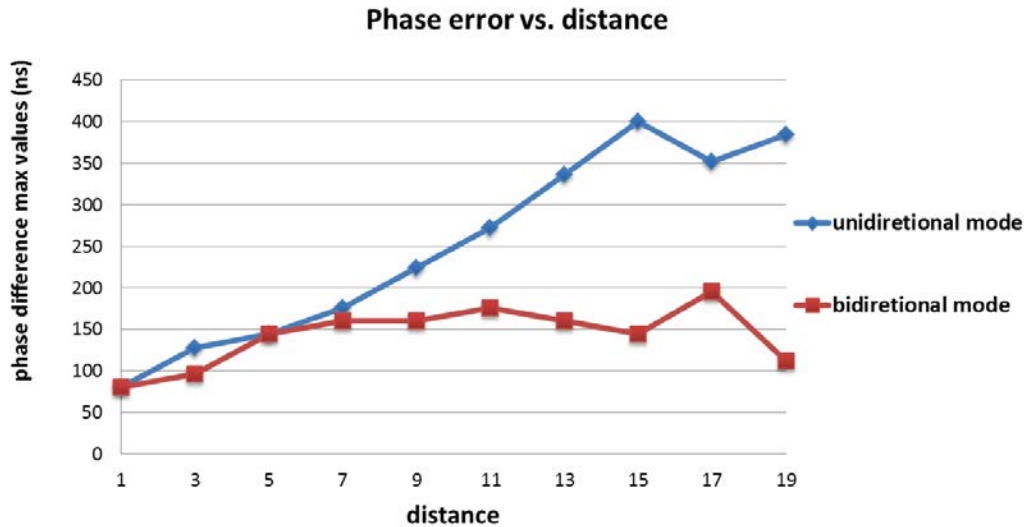
Figure 9: La valeur maximale de l'erreur de phase en fonction de la distance par rapport à l'horloge de référence
