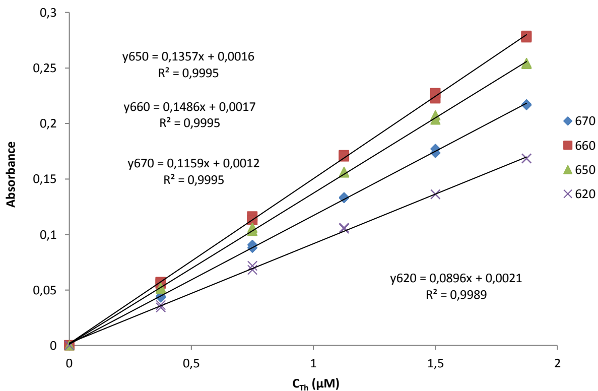
Figure 9 : Courbes d'étalonnage pour différentes longueurs d'onde (de 620 nm à 670 nm), avec deux mesures sur chaque point
