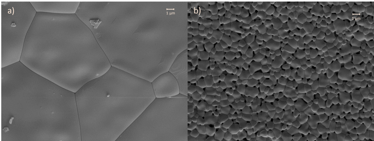
Figure I-5: Images MEB (microscopie à double faisceau SEM/FIB du CSNSM à Orsay) de deux pastilles réalisées dans des conditions différentes, même grossissement x4000, tension de 5 kV en électrons secondaires a) Pastille chauffée à 1700°C, frittage important, pas de porosité ouverte b) Pastille chauffée à 1400°C, frittage faible, porosité ouverte importante (27%)
