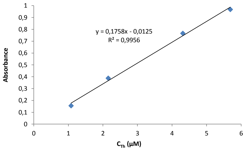
Figure 8 : Courbe d'étalonnage obtenue avec une solution d'arsenazo à 0,0075% dans \text{HClO}_4 2 M
