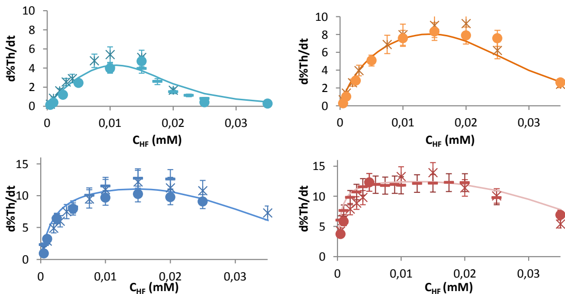
Comparaison entre les taux initiaux de dissolution obtenus par la modélisation (traits plein) et lors de trois sets de résultats expérimentaux (● expérience a, X expérience b, — expérience c) à quatre concentrations en acide nitrique (turquoise 1 M, orange 2,5 M, bleu 5 M et rouge 10 M)
