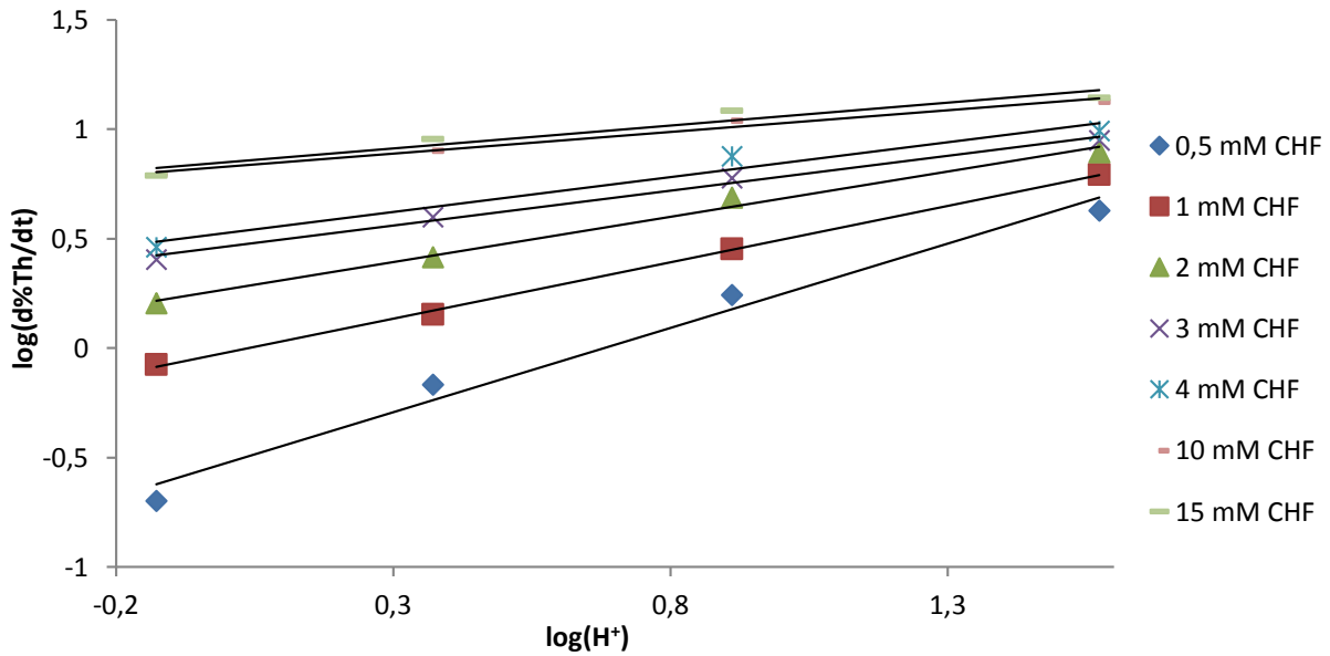
Figure II-9 : Détermination de l'ordre de réaction relatif à l'acidité en traçant \log\left(\frac{d\%Th}{dt}\right) en fonction de \log(H^+)
