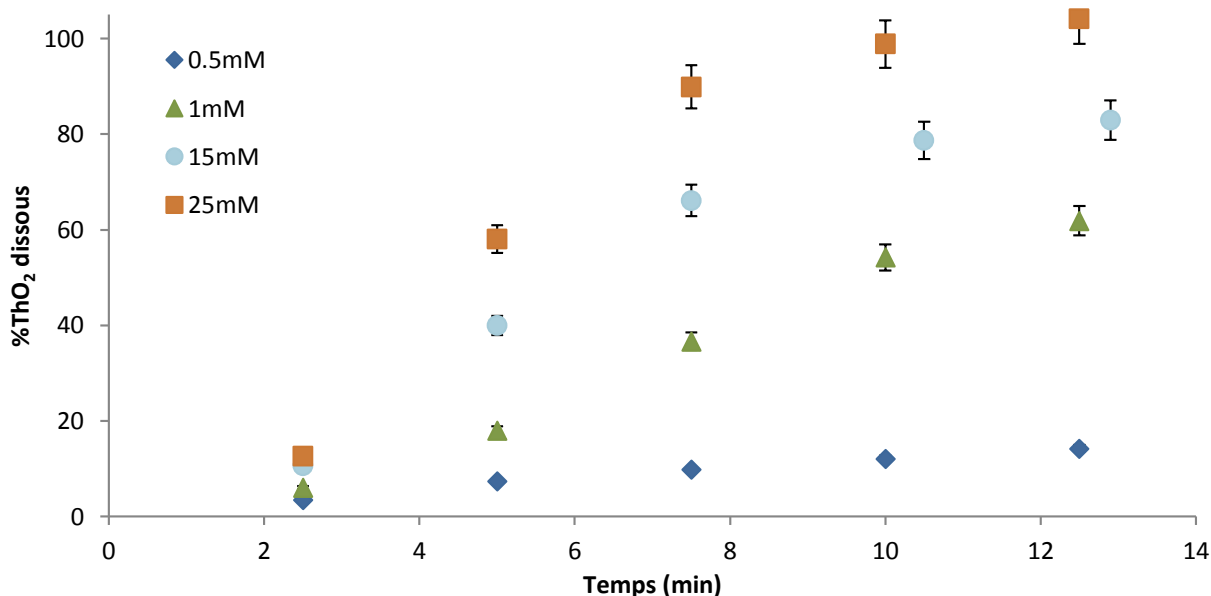
Figure I-25 : Pourcentage de masse de ThO 2 dissoute en fonction du temps dans le milieu HNO 3 5 M, surface spécifique de 1,5 m 2 /g, 130 mg dans 20 mL, 70°C
