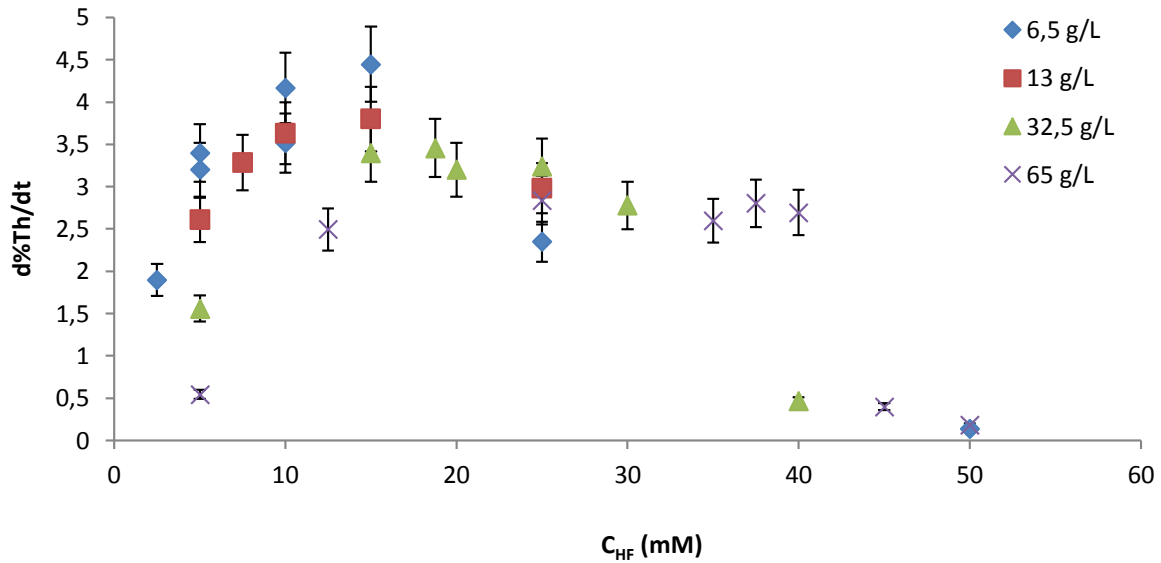
Figure II-14 : Variation du taux de dissolution en fonction de la concentration à différents rapports masse/volume à 5 M \text{HNO}_3 , 5 mM HF, 50°C, 1 \text{m}^2/\text{g}
