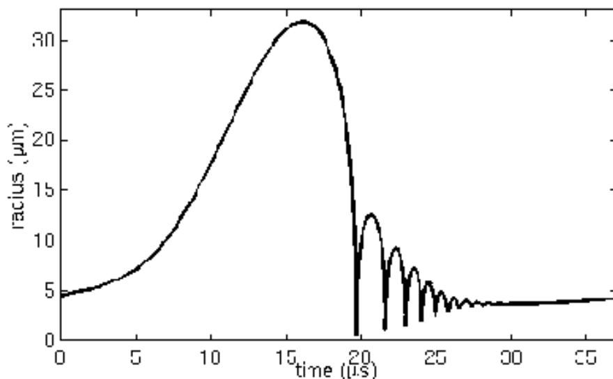
Figure I-13 : Evolution du rayon moyen (en µm) d'une bulle de cavitation au cours du temps, http://faculty.olin.edu/bstorey/sonochem/
