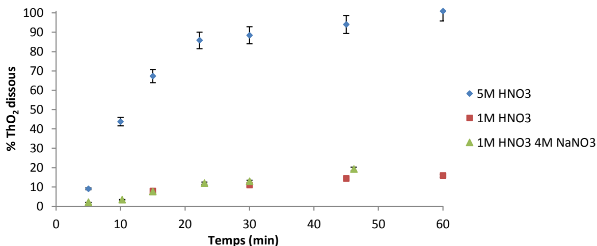
Figure II-4 : Comparaison de l'effet des nitrates et des protons sur la dissolution, C_{\text{HF}} 5 mM, température ambiante, 6,8 \text{ m}^2/\text{g} , 130 mg dans 20 mL
