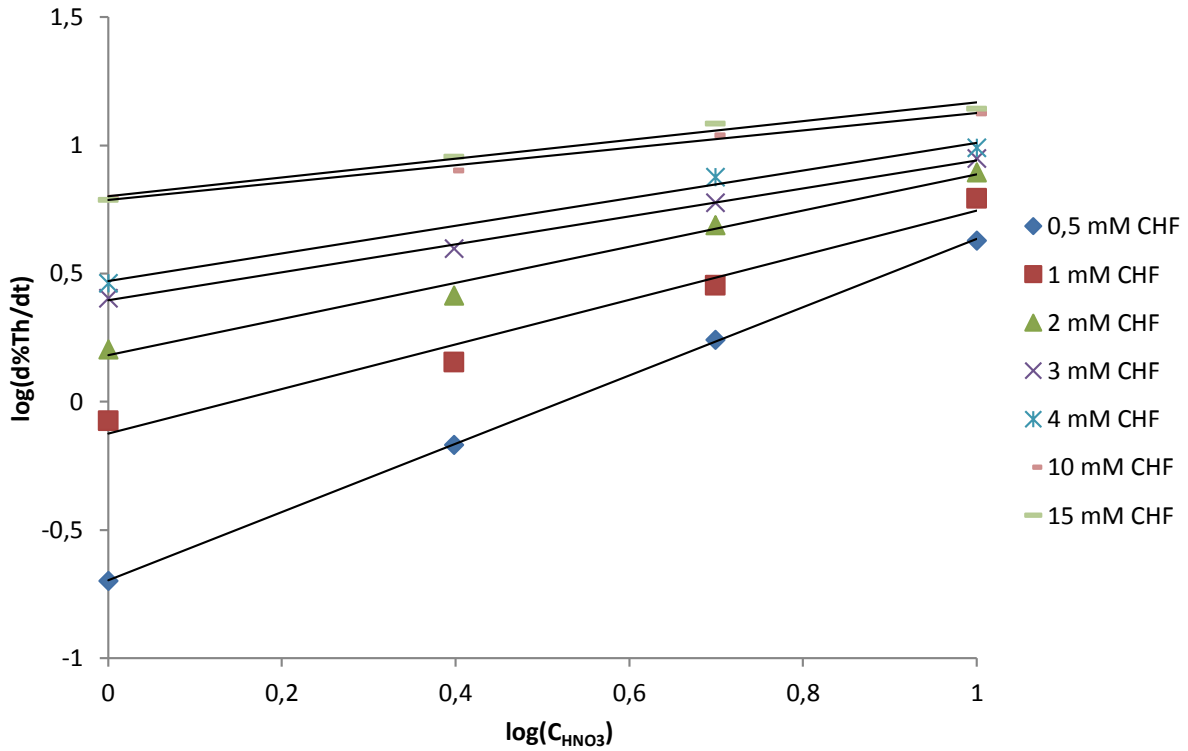
Figure II-8 : Détermination de l'ordre de réaction relatif à la concentration en acide nitrique en traçant \log\left(\frac{d\%Th}{dt}\right) (0) en fonction de \log(C_{HNO_3}) à différentes concentrations en acide fluorhydrique
