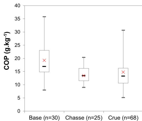
Figure 8-7 : Teneurs en COP dans les MES durant les différents régimes hydrologiques sur l'Isère à la station campus (les données de régime de base, chasses et crues correspondent au suivi 2011-2012)
