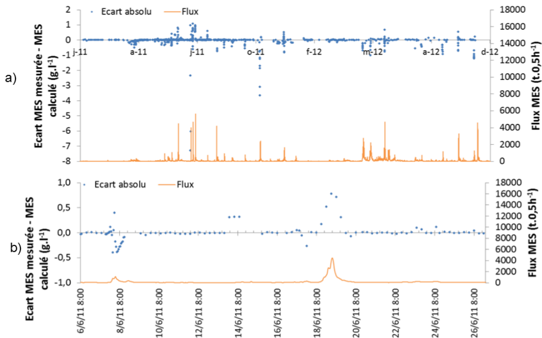
Figure 5-2 : Écart absolu entre la concentration en MES mesurée et la concentration en MES calculée par la relation MES-turbidité et flux de MES calculés a) en 2011-2012, b) zoom sur 20 jours
