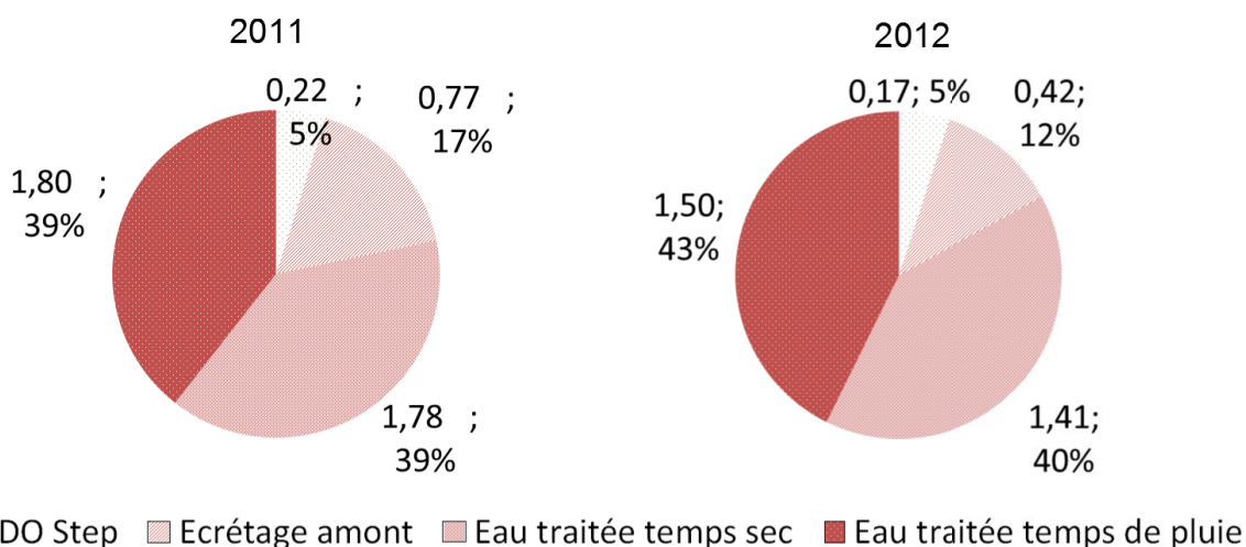
Figure 9-20 : Estimation des flux moyens de HgTP (kg.an -1 ) déversés par la Step, et contributions au rejet total de chaque type de rejet
