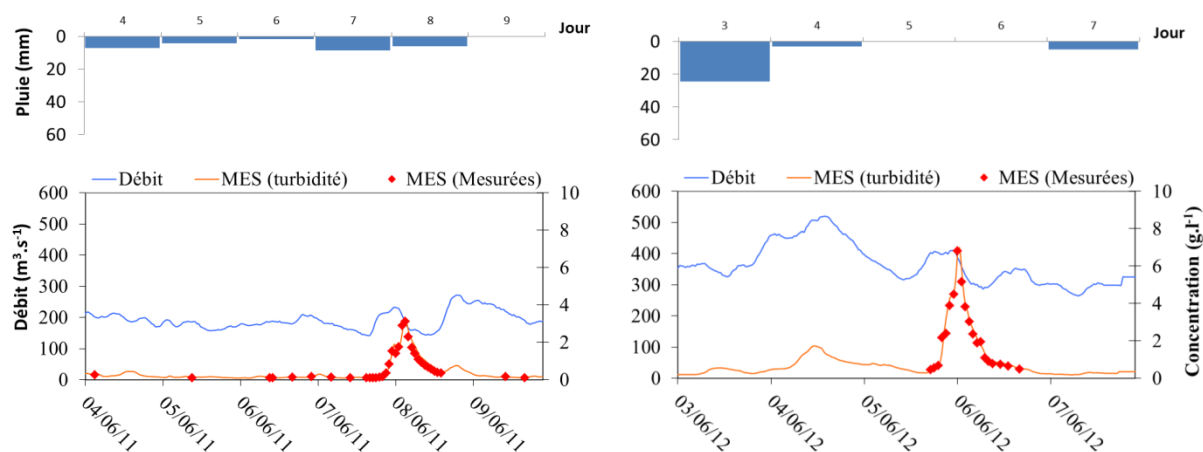
Figure 6-16 : Chroniques de débits et de MES à la station campus lors des chasses hydrauliques de l'Arc 2011 et 2012 (Précipitation moyenne sur l'agglomération)
