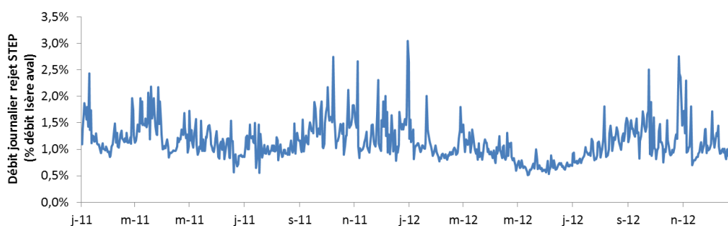
Figure 6-39 : Débits journaliers des rejets Step exprimés en pourcentage du débit journalier moyen de l'Isère à Saint-Gervais en 2011 et 2012
