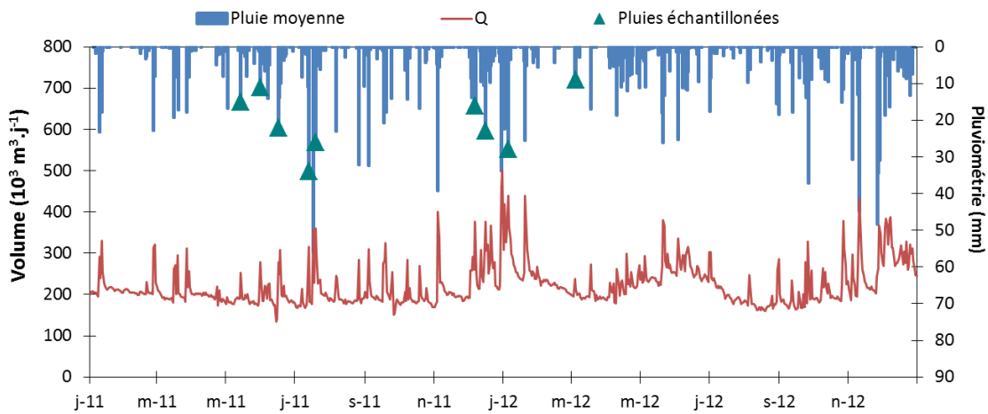
Figure 6-38 : Volumes journaliers moyens déversés en sortie de la station d'épuration Aquapole en 2011 et 2012
