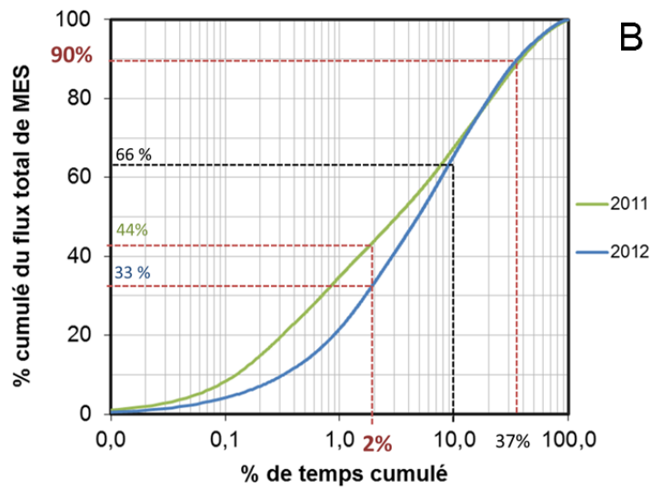
Figure 6-26 : Flux cumulé de MES en fonction du pourcentage de temps par année à la station Isère campus A) entre 2006 et 2012, B) en 2011 et 2012
