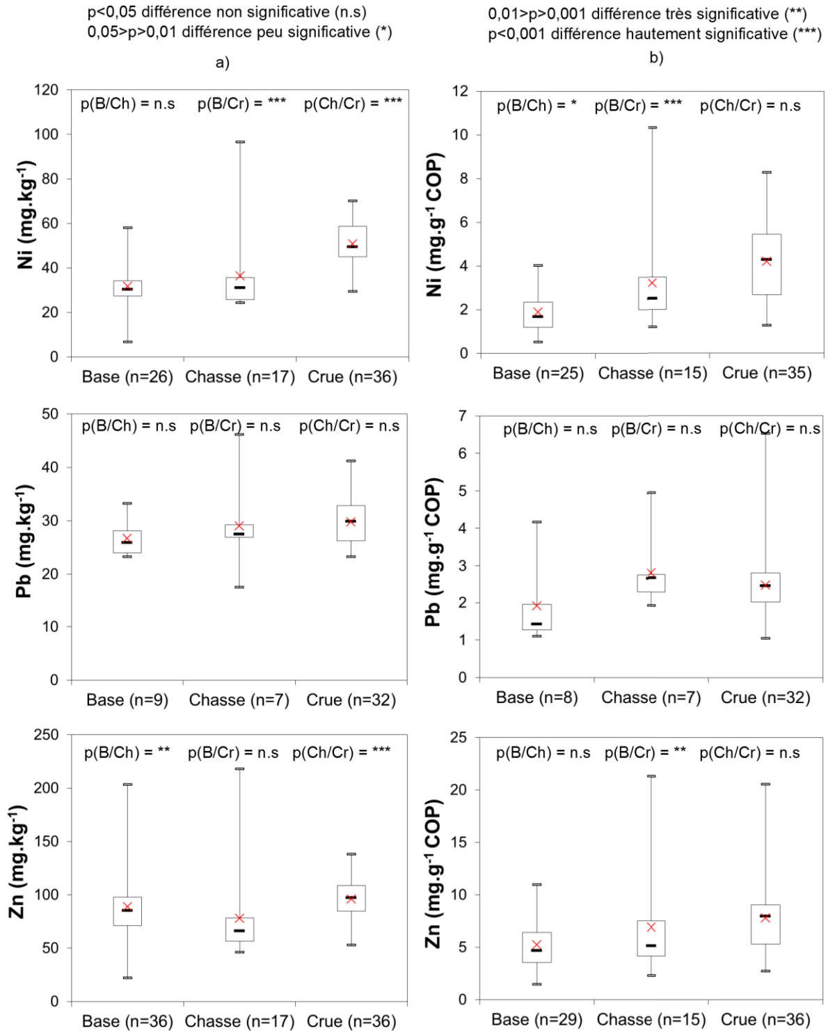
Figure 8-9 : Teneurs en, Ni, Pb et Zn, a) non normalisées et b) normalisées par la concentration en COP, à la station Isère campus en régime de base (B), lors des chasses de l'Arc (Ch), lors des crues 2011-2012 (Cr) (p(X/Y) indique le degré de significativité de l'écart entre les séries X et Y)
