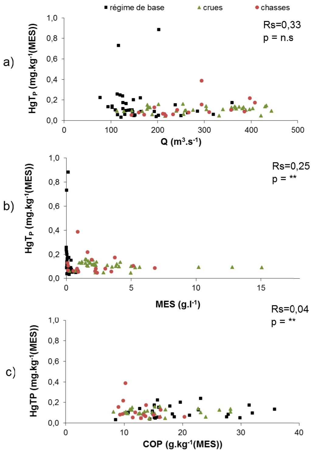
Figure 9-14 : Teneurs en mercure total dans les MES à la station campus en fonction a) du débit, b) de la concentration en MES et c) du COP sur la période 2011-2012 ( R_s : coefficient de Spearman, p le niveau de significativité du coefficient)
