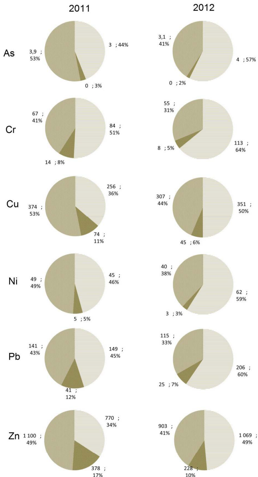
Figure 8-11 : Flux d'ETM particulières (kg) déversés par l'ensemble des DO, par le DO Step et l'écrêtage et par les eaux traitées de la Step (en temps sec et en temps de pluie) en 2011 et 2012 et proportion du déversement total du système d'assainissement
