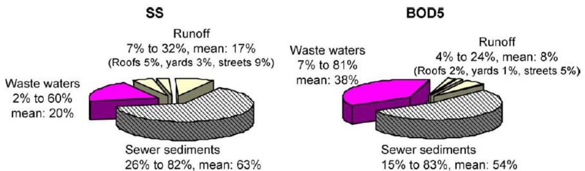
Figure 1-20 : Contribution du ruissellement, des eaux usées et des sédiments déposés aux flux de MES et DBO 5 dans les RUTP (contributions minimum, maximum et moyennes sur 31 événement pluvieux) [Chebbo and Gromaire, 2004]
