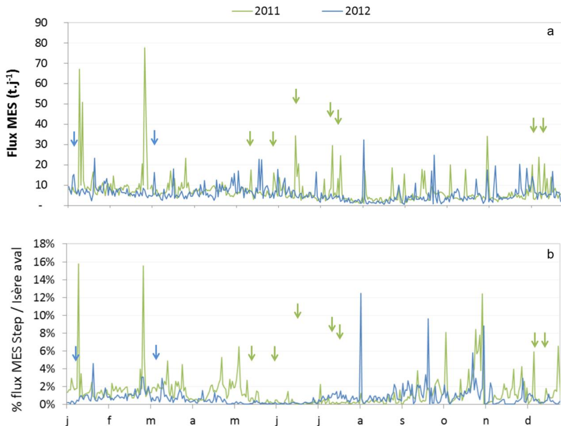
Figure 6-52 : a) Flux journaliers de MES en sortie de la station d'épuration Aquapole en 2011 et 2012 b) proportion des flux de MES journaliers rejetés par la Step par rapport au flux transité dans le milieu récepteur à l'aval de la Step (les flèches indiquent les pluies échantillonnées)
