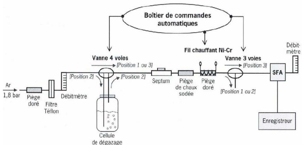
Figure 4-1 : Schéma de montage du dosage analytique du mercure total dissous [Cossa et al., 2003]
