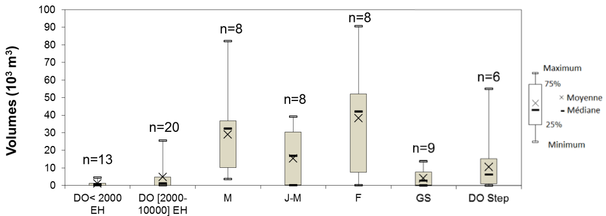
Figure 6-43 : Variabilité spatiale des volumes déversés par les différentes tailles des DO lors des événements pluvieux échantillonnés
