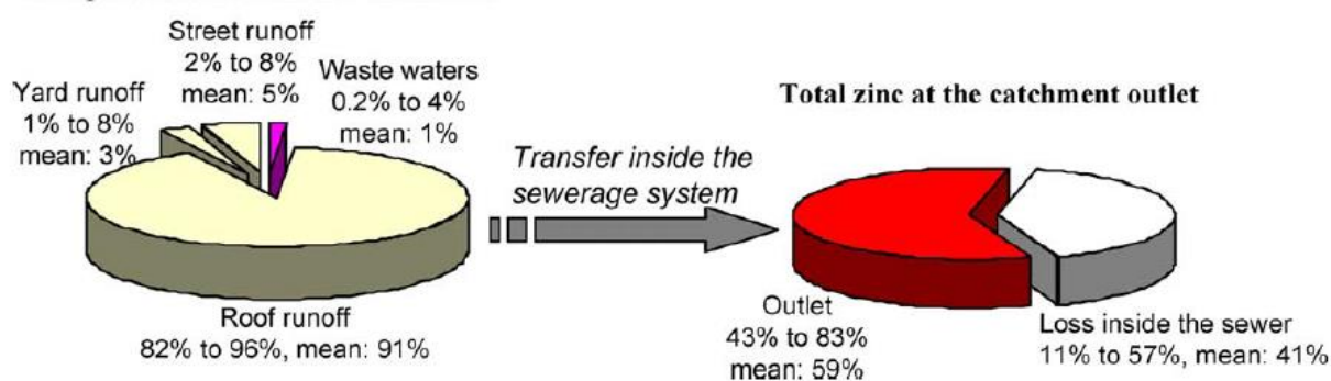
Figure 1-21 : Contributions des différentes sources de production de zinc total et leur évolution lors du transport dans le réseau (contributions minimum, maximum et moyennes sur 11 événements pluvieux) [Chebbo and Gromaire, 2004]
