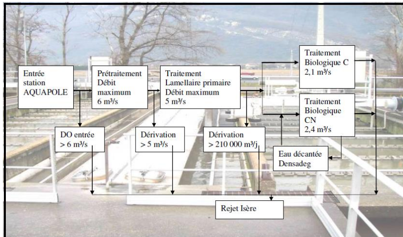
Figure 2-14 : Schéma de fonctionnement de la station d'épuration Aquapôle [Société Dauphinoise d'Assainissement, 2010]
