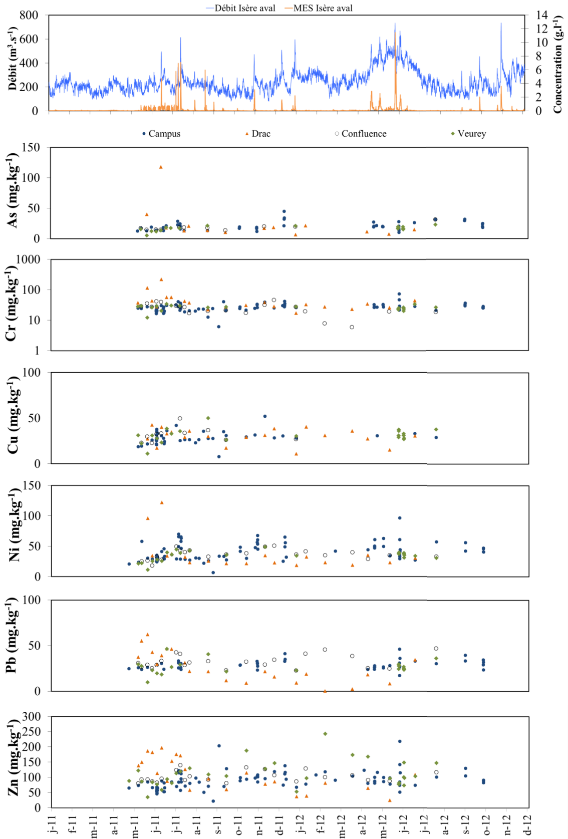
Figure 8-3 : Variation temporelles des concentrations en ETM particulaires aux stations de suivi amont et aval agglomération
