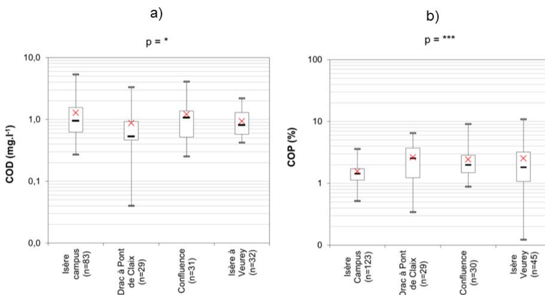
Figure 7-5 : Concentrations en a) COD (mg.L -1 ) et b) COP (exprimées en pourcentage de la concentration en MES) aux stations de suivi amont et aval agglomération issues des mesures LTHE
