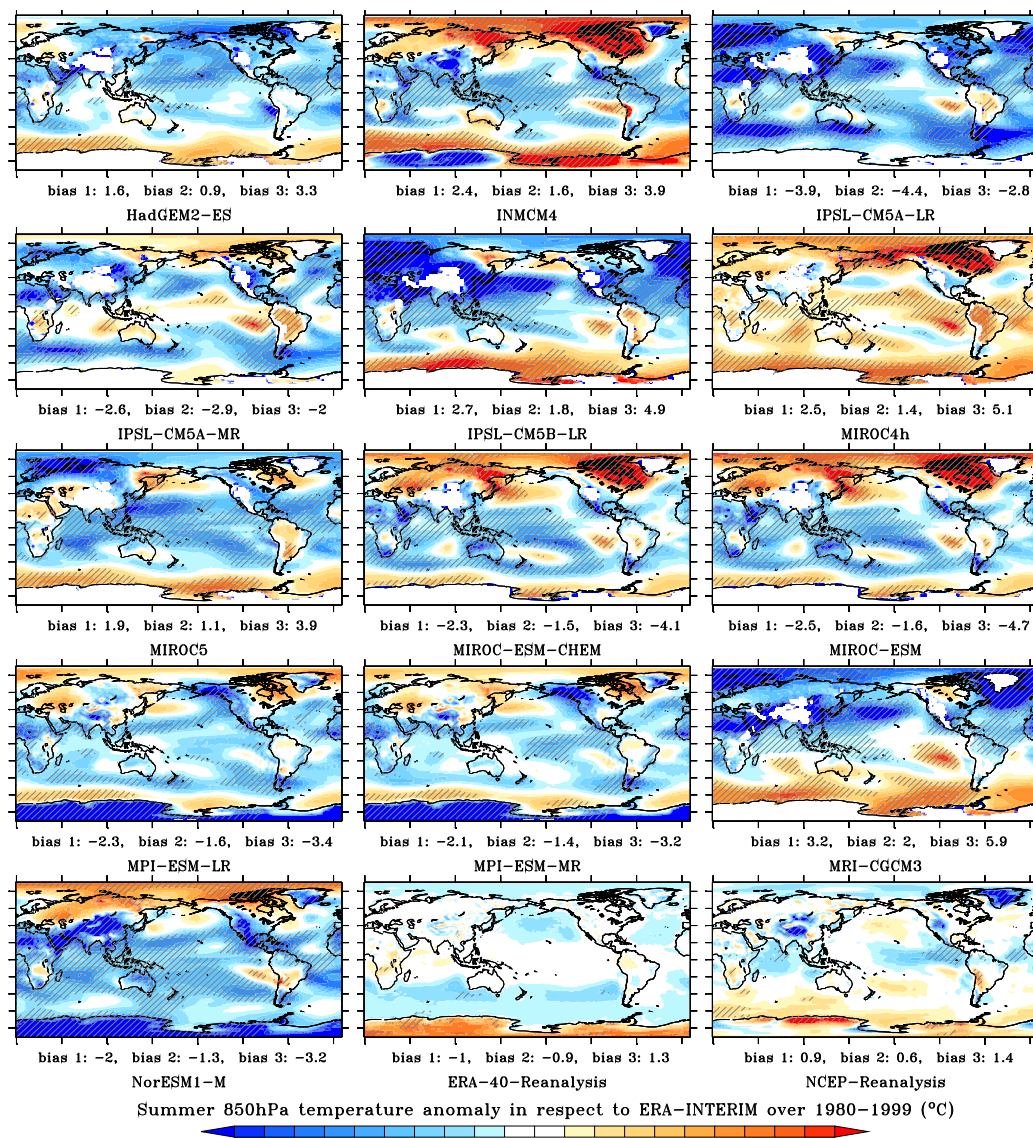
FIGURE G.1 – Anomalie moyenne ( \overline{T}_{CMIP5} - \overline{T}_{ERA-Int} ) de température estivale (DJF) à 850hPa par rapport à ERA-Interim sur la période 1980-1999, tracée sur la grille d'ERA-Interim. Les biais indiqués sont calculés de la manière suivante : (\overline{T}_{CMIP5} - \overline{T}_{ERA-Int}) / \sigma(T_{ERA-Int}) , où \sigma représente l'écart-type. Le biais 1 est calculé sur l'ensemble de la zone 40° S - 90° S, le biais 2 sur la zone 40° S - 60° S et le biais 3 sur la zone 60° S - 90° S. Les zones hâchurées représentent les endroits où l'anomalie de température est plus de deux fois supérieure à l'écart-type de la température dans le modèle CMIP5.
