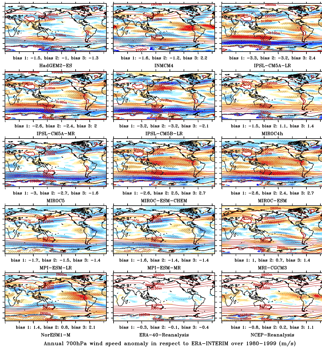
FIGURE G.2 – Anomalie moyenne ( \overline{WS}_{CMIP5} - \overline{WS}_{ERA-Int} ) de vitesse du vent annuelle à 700hPa par rapport à ERA-Interim sur la période 1980-1999, tracée sur la grille d'ERA-Interim. Les biais indiqués sont calculés de la manière suivante : (\overline{WS}_{CMIP5} - \overline{WS}_{ERA-Int})/\sigma(WS_{ERA-Int}) , où \sigma représente l'écart-type. Le biais 1 est calculé sur l'ensemble de la zone 40° S - 90° S, le biais 2 sur la zone 40° S - 60° S et le biais 3 sur la zone 60° S - 90° S. Les contours correspondent à la hauteur du géopotential 700 hPa. Les zones hachurées représentent les endroits où l'anomalie de vitesse du vent est plus de deux fois supérieure à l'écart-type de la vitesse du vent dans le modèle CMIP5.
