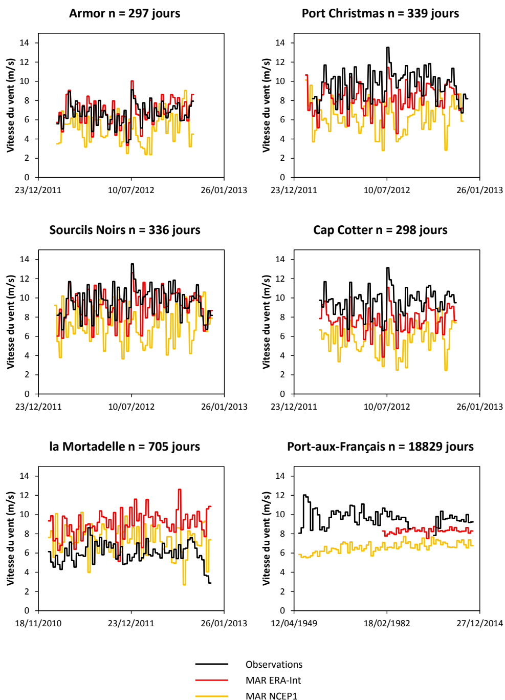
FIGURE H.2 – Séries temporelles de la vitesse du vent journalière en surface simulée par le MAR forcé par ERA-Interim et par NCEP1 en chaque point de grille contenant une station météorologique et de la vitesse du vent journalière en surface mesurée à cette station. Par souci de lisibilité, les mesures du réseau Kcrumble sont moyennées sur 5 jours, celles de la Mortadelle sur 10 jours et celles de PAF sur 300 jours.
