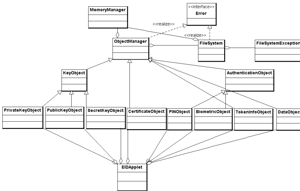
FIGURE 4.7 – Diagramme de classes de l'applet PKCS15
