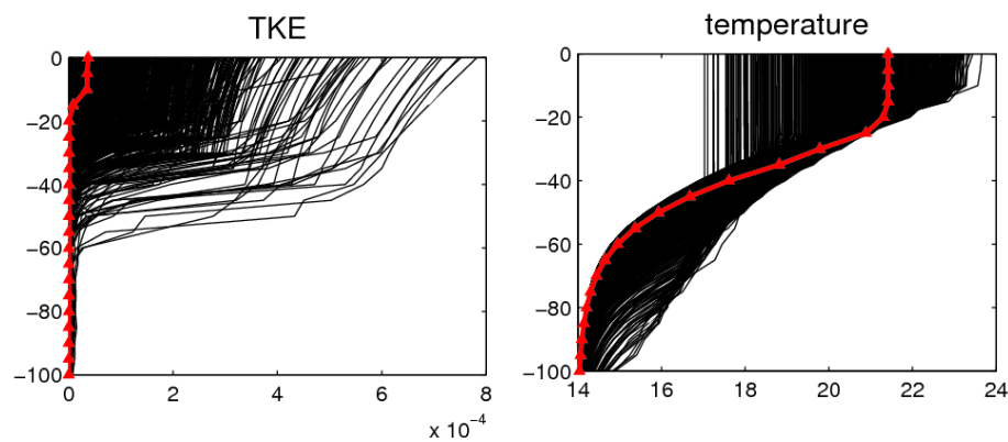
FIGURE 2.9 – Prévision d'ensemble (1000 membres) d'un profil d'énergie cinétique turbulente (en m^2/s^2 ) et de température potentielle (en ^{\circ}C ), en réponse à une incertitude sur le forçage atmosphérique (d'après Lauvernet et al., 2009). La ligne rouge représente la prévision déterministe, réalisée avec l'espérance mathématique du forçage.
