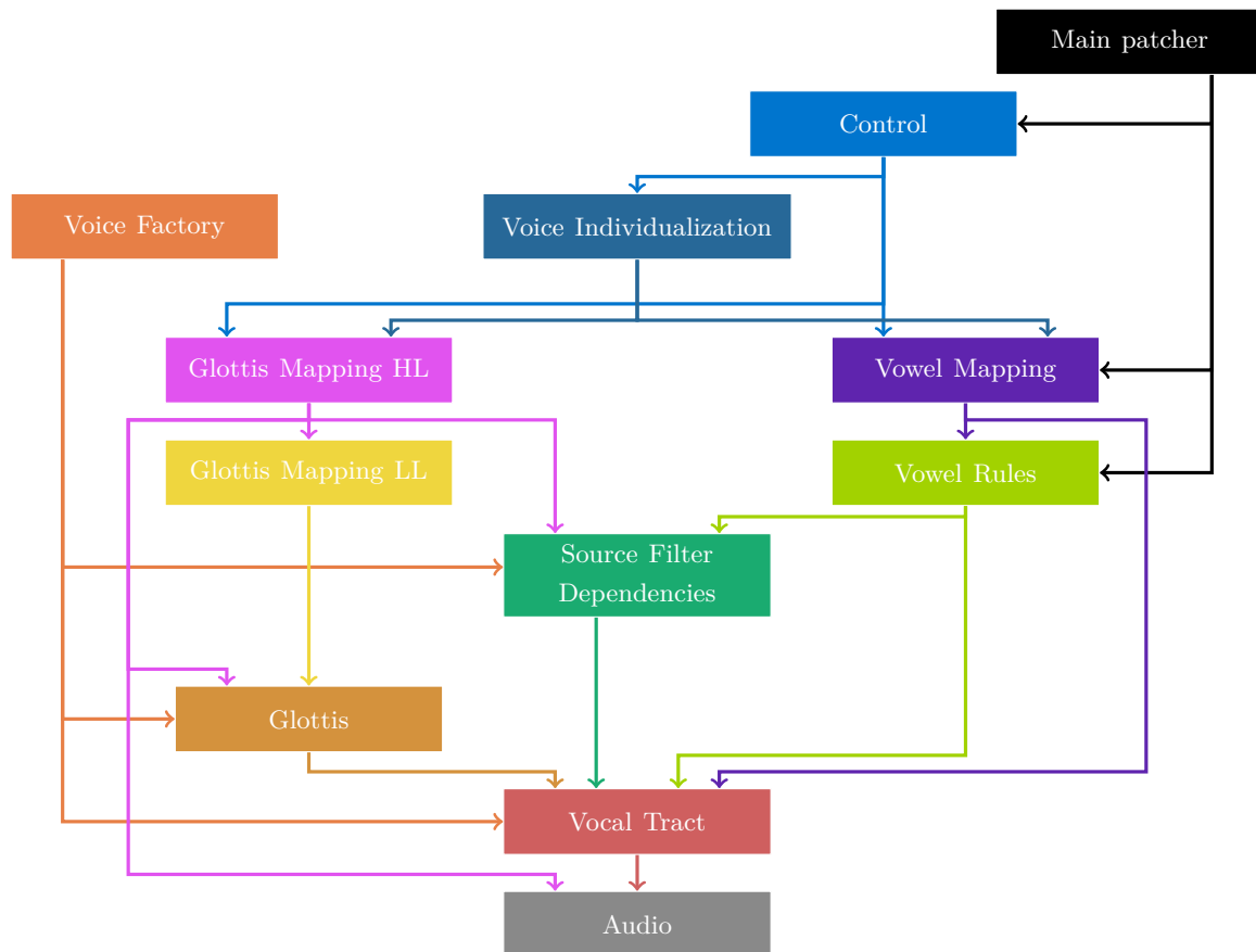
FIGURE 2.11 – Schéma de la hiérarchie du code.
