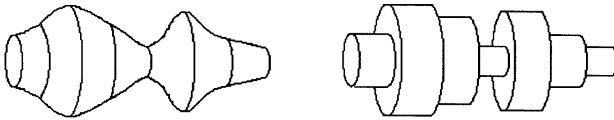
FIGURE 1.2 – Schéma du tube acoustique représentant le conduit vocal à gauche, et sa version discrétisée à droite, d’après [Coo90].
