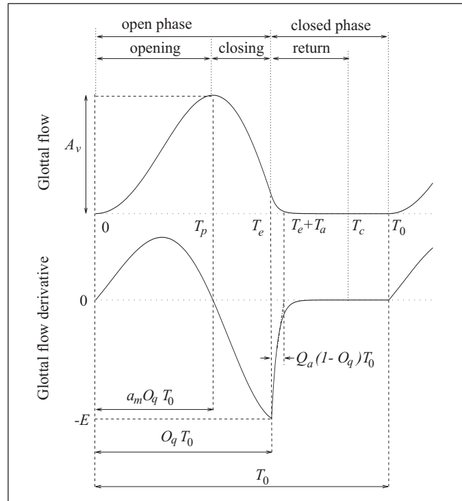
FIGURE 2.1 – Paramètres décrivant l'ODG (haut) et sa dérivée (bas), d'après [DdH06].
