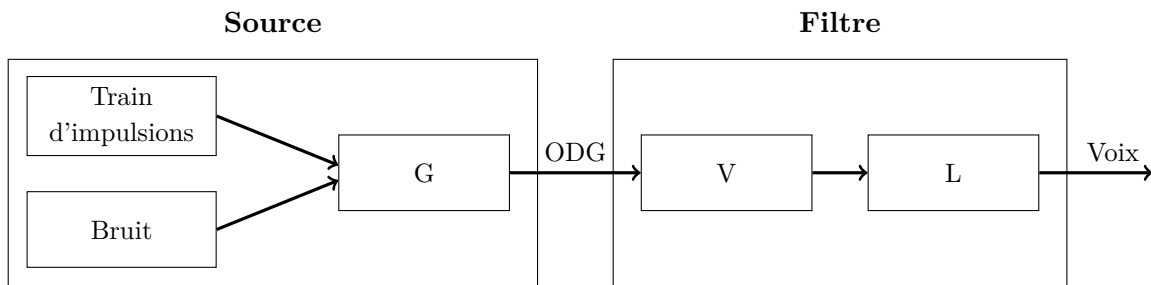
FIGURE 1.4 – Modèle source-filtre.
