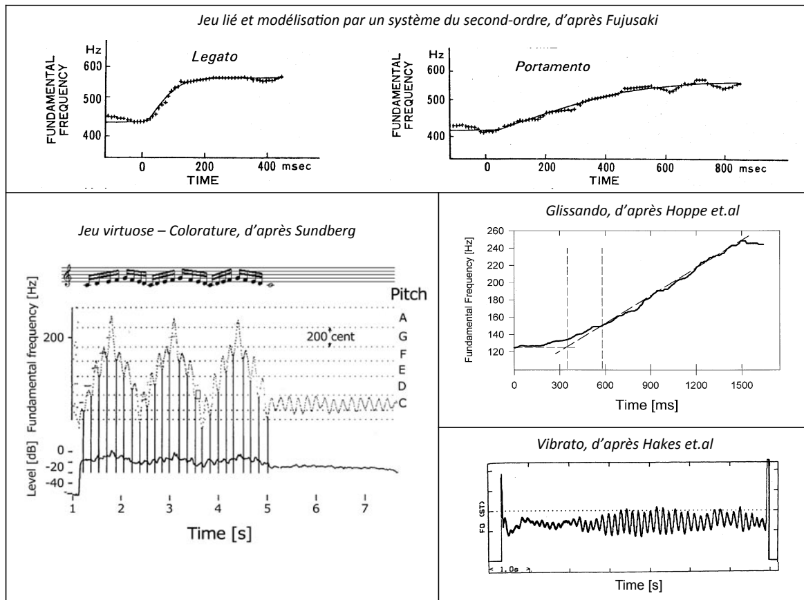
FIGURE 6.7 – Exemples d'effets musicaux : jeu lié legato et portamento d'après [Fuj81], jeu virtuose d'après [Sun06], jeu glissando d'après [HRD + 03] et jeu vibrato d'après [HSD87].
