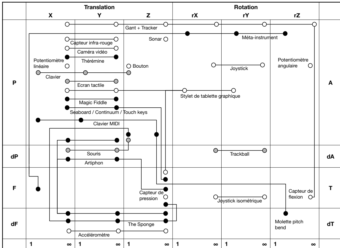
FIGURE 1.8 – Capteurs classés selon leur mode d'acquisition [VUK96], [OSW01], d'après la représentation de [CMR91]. Les colonnes sont les différents degrés de liberté, les lignes les grandeurs mesurées, et la résolution des capteurs dépend de leurs positions horizontales dans chaque case. En blanc, les voies gestuelles des capteurs individuels ; en gris, les voies gestuelles d'interfaces pour l'ordinateur ; en noir, les voies gestuelles d'instruments de musique numériques. Les voies appartenant aux mêmes canaux gestuels sont reliées par des segments.
