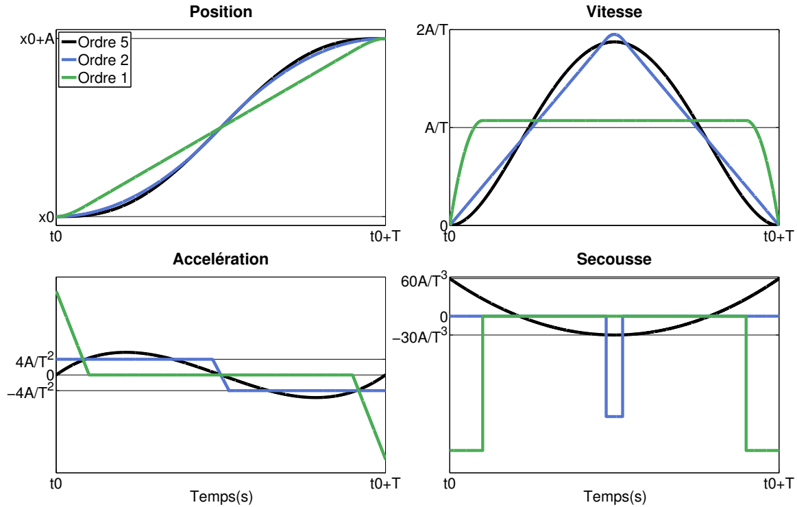
FIGURE 6.6 – Trajectoires théoriques d'une dimension minimisant les coûts de secousse (ordre 5), de force (ordre 2) et d'impulsion (ordre 1) et leurs profils de vitesse, d'accélération et de secousse respectifs.
