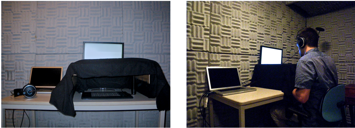
FIGURE 5.1 – Disposition de l'expérience. Gauche : la tablette est placée sous un support opaque et un écran derrière le support affiche le retour visuel. Droite : Position adoptée par un sujet pour l'expérience.
