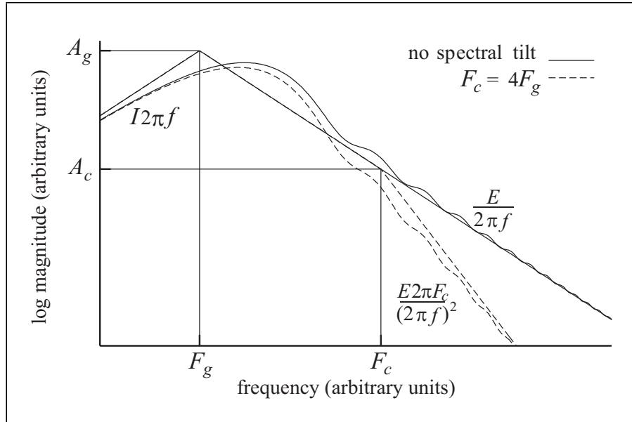
FIGURE 2.2 – Représentation spectrale de la source glottique, d'après [DdH06].
