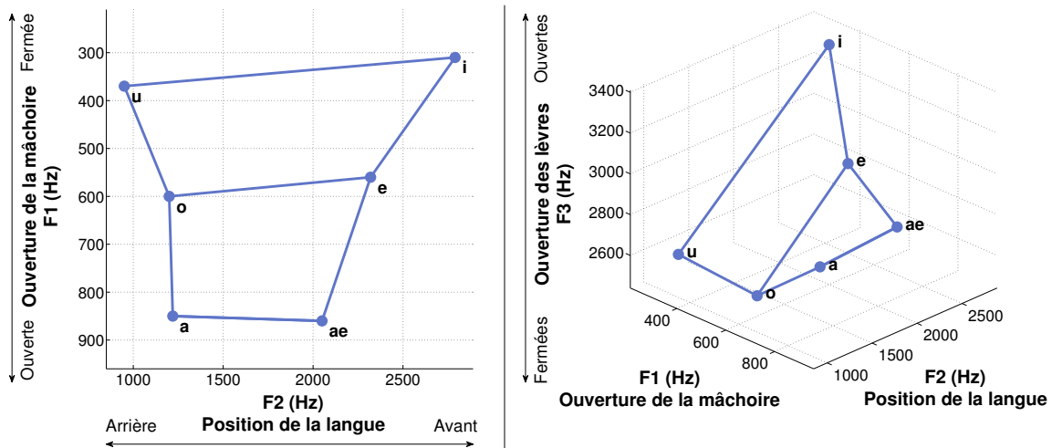
FIGURE 1.3 – Représentation des voyelles extrêmes du français dans le plan des deux premiers formants (gauche) et dans l'espace des trois premiers formants (droite).
