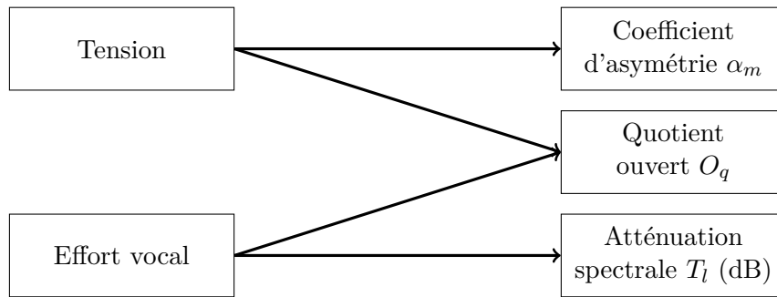
FIGURE 2.3 – Relation entre paramètres de qualité de voix et paramètres de source, d’après [dWF + 07].
