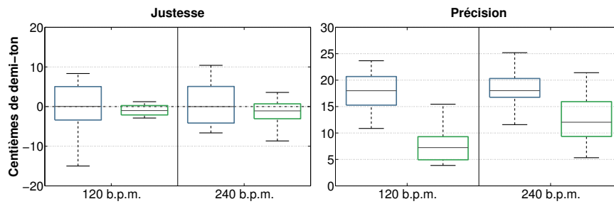
FIGURE 4.10 – Justesse (gauche) et précision (droite) des sujets en fonction du tempo. Pour chaque condition la boîte de gauche en bleu (resp. droite en vert) contient les valeurs d’entrée (resp. sortie) de chaque réalisation.
