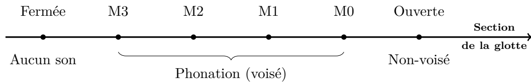
FIGURE 1.6 – Evolution des mécanismes et des modes de production de parole correspondants en fonction de la section de la glotte.
