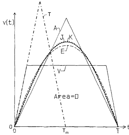
FIGURE 6.5 – Profils de vitesse minimisant le coût de : T - Temps ; A - Accélération ; V - Vitesse ; E - Energie ; J - Jerk ; K - Profil de vitesse d'un système masse-ressort, d'après [Nel83].
