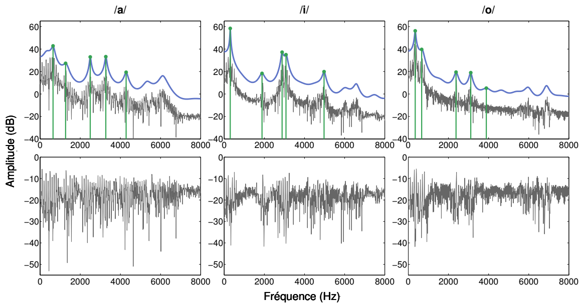
FIGURE 1.5 – Décomposition source-filtre par analyse LPC d'ordre 64. Le signal de parole est représenté en haut. L'enveloppe spectrale induite par le conduit vocal et extraite par LPC est indiquée en bleue. Les 5 premiers maxima correspondant aux premiers formants sont relevés en vert. Le signal de source obtenu par déconvolution du signal de parole est affiché en bas. De gauche à droite, les voyelles /a/, /i/ et /o/.
