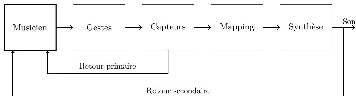
FIGURE 1 – Schéma d'un instrument de musique numérique, d'après [WD04].
