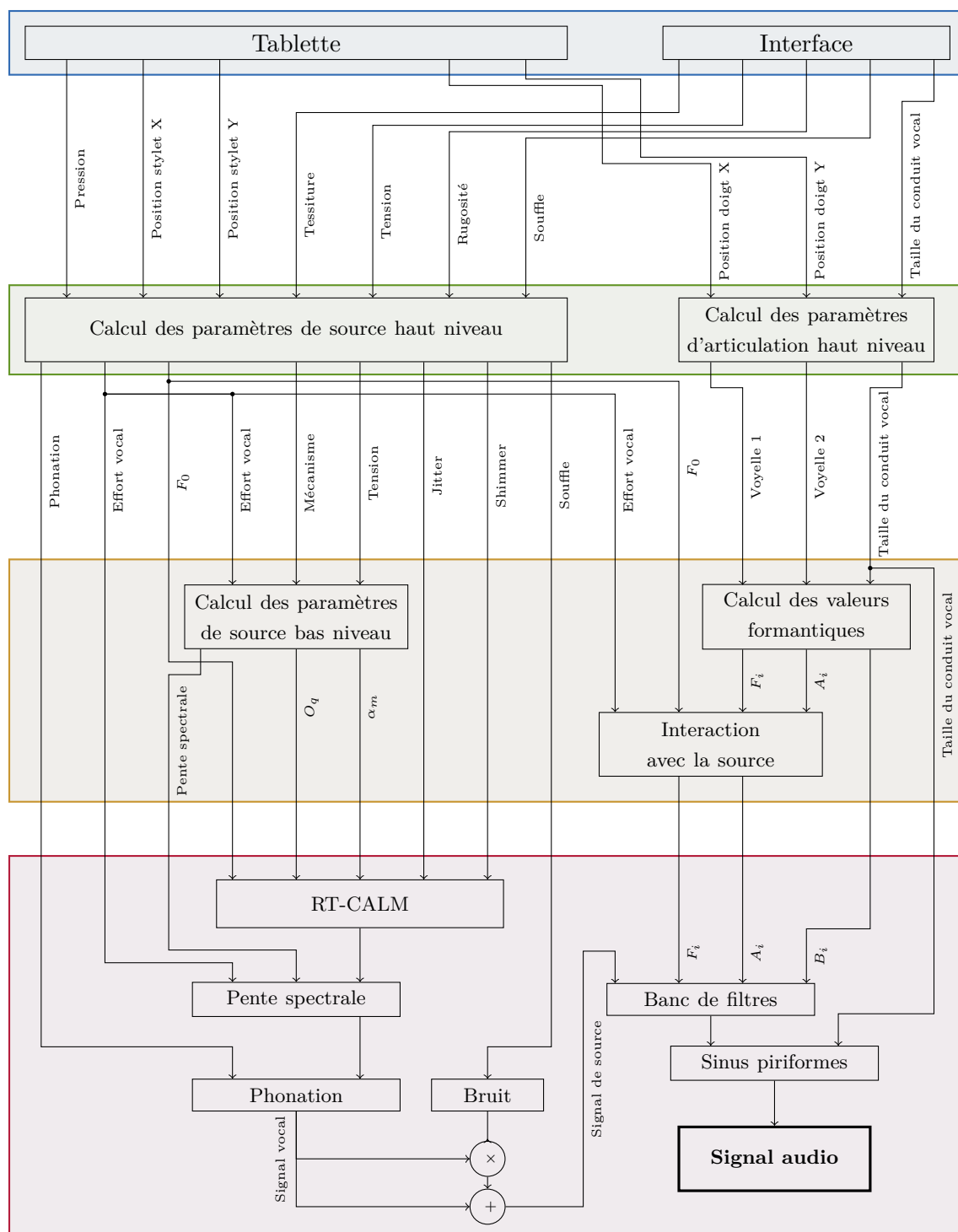
FIGURE 2.6 – Schéma d'évolution des paramètres du Cantor Digitalis.
