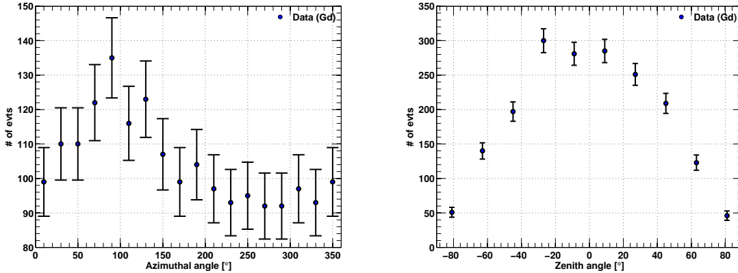
Figure C.20: Distribution des angles azimutaux (gauche) et zénithaux (droite) pour chaque évènement du jeu de données n-Gd du détecteur proche.
