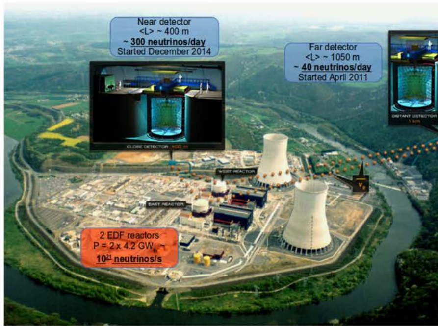
Figure C.26: Site expérimental de l'expérience Double Chooz.
