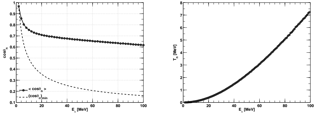
Figure C.10: Gauche: Valeurs moyennes (cercles) et maximales (ligne segmentée) du cosinus de l'angle d'émission du neutron \cos \theta_n en fonction de l'énergie du neutrino. Droite: Énergie cinétique moyenne T_n du neutron en fonction de l'énergie du neutrino.
