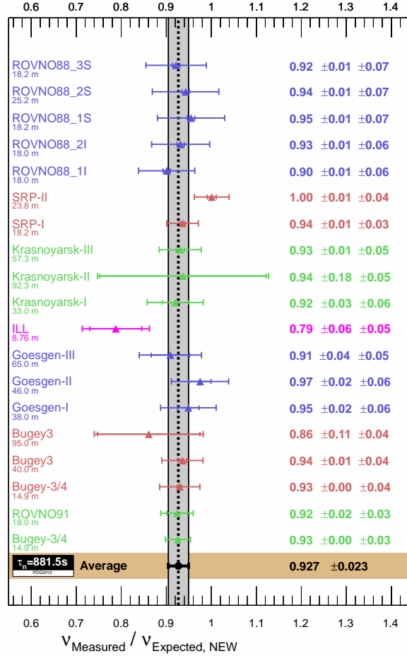
Figure C.4: Ratio du taux d'événements observé/attendu en fonction de la ligne de vol pour les expériences de réacteurs à courtes distances. La bande grise correspond à l'ajustement moyen avec son incertitude associée [96].
