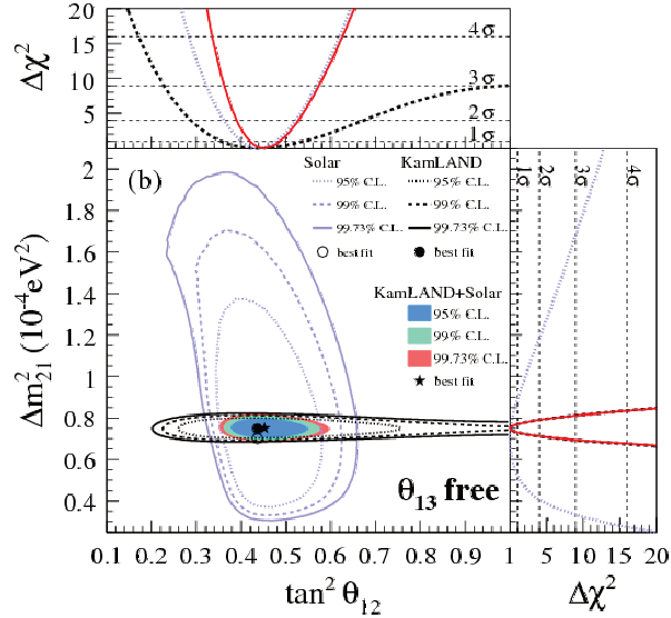
Figure C.2: Régions permises dans le plan (\tan^2 \theta_{12}, \Delta m_{21}^2) pour les données des expériences solaires et de KamLAND dans le cadre des oscillations à 3 neutrinos. L'angle de mélange \theta_{13} est ici considéré comme un paramètre libre [61].
