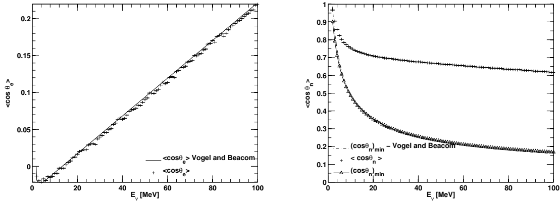
Figure C.12: Gauche: Cosinus moyen des angles entre la direction du positron (gauche) et du neutron (droite) et du neutrino. Les calculs analytiques effectuées par Vogel-Beacom sont incluses pour illustrer la fidélité de SuperNustradamus [158].
