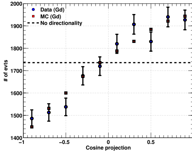
Figure C.16: Distribution \cos \alpha pour chaque événement dans le jeu de données n-Gd (cercles bleus) et du MC normalisé (carrés rouges).
