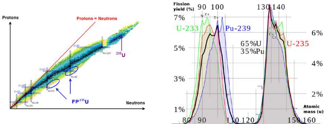
Figure C.5: Gauche: Localisation des fragments de fission de l' ^{235}\text{U} sur le tableau des noyaux [121]. Droite: Distribution des fragments de fission créés par les fission de l' ^{235}\text{U} , du ^{239}\text{Pu} , de l' ^{233}\text{U} et d'un combustible hybride (65% U, 35% Pu) [122].
