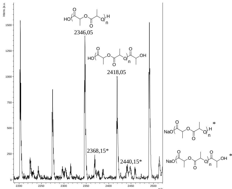
Figure IV-5 : Spectre de masse MALDI-TOF du mélange réactionnel issu de la ROP du L -LA, en utilisant le squelette PBu 85 comme macroamorceur et le TBD comme catalyseur, avec un rapport initial [\text{L-LA}]_0/[\text{OH}]_0 = 35 ; matrice : trans -2-[3-(4- tert -butylphényl)-2-méthyl-2-propénylidène]malononitrile + trifluoroacétate de sodium (DCTB + NaTFA).
