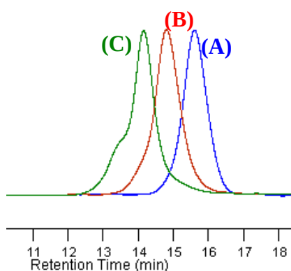
Figure II-7 : Chromatogrammes SEC de (A) 1-PCL 16 (Tableau II-2, Entrée 1), (B) 1-PCL 38 (Tableau II-2, Entrée 3), (C) 1-PCL 84 (Tableau II-2, Entrée 4).
