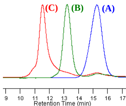
Figure II-20 : Chromatogrammes SEC du (A) 2-PCL 19 précipité (Tableau II-2, Entrée 5), du (B) PBu 10 -g-1-PCL 19 brut après 3 h de réaction (Tableau II-3, Entrée 8) et du (C) PBu 50 -g-1-PCL 19 brut après 3 h de réaction (Tableau II-2, Entrée 9).
