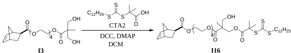
Schéma I-50 : Schéma de synthèse de l'inimer I16 , possédant des extrémités OH et trithiocarbonate.
