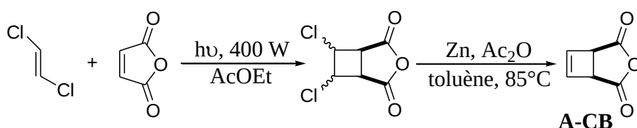
Schéma II-1 : Synthèse de l'anhydride cis-cyclobut-3-ène-1,2-dicarboxylate anhydride A-CB.
