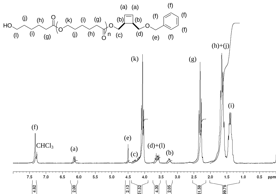
Figure II-9 : Spectre RMN ^1\text{H} (200 MHz, \text{CDCl}_3 , 25 °C) du 1-PCL 16 précipité obtenu par ROP de l' \epsilon -CL dans le THF à 25°C en utilisant l'inimer 1 comme amorceur et le TBD comme catalyseur pour un rapport [\epsilon\text{-CL}]_0/[\text{OH}]_0 = 18 (Tableau II-2, Entrée 1).
