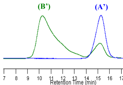
Figure II-15 : Chromatogrammes SEC du (A') 1-PCL 16 précipité (Tableau II-2, Entrée 1) et du (B') PBu 100 - g -1-PCL 16 brut après 3 h de réaction (Tableau II-3, Entrée 5).
