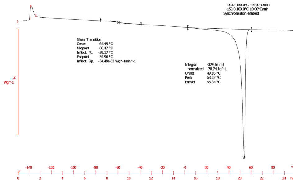
Figure S1 : Thermogramme obtenu en DSC pour le copolymère greffé PBu 200 -g-PCL 48 (Tableau IV-5, Entrée 10) avec une vitesse de chauffe et de refroidissement de 10 °C.min -1 .
