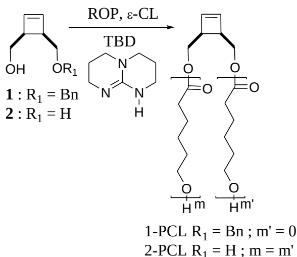
Schéma II-5 : Synthèse des macromonomères 1-PCL et 2-PCL.
