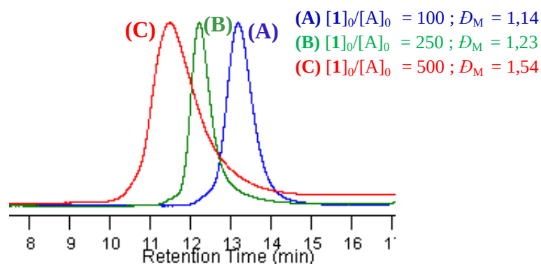
Figure IV-1 : Chromatogrammes SEC des PBus précipités obtenus à l'issue des ROMPs de 1 à 50°C dans le C 2 H 4 Cl 2 en présence de G2 pour des rapports [1]_0/[A]_0 = (A) 100, (B) 250 et (C) 500 (Tableau IV-1, Entrées 1, 3 et 5).
