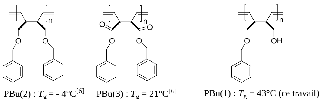
Schéma IV-2 : Structures et températures de transition vitreuse ( T_g ) des poly(1,4-butadiène)s PBu(2), PBu(3) et PBu(1) obtenus par ROMP de dérivés CB 3,4-disubstitués.
