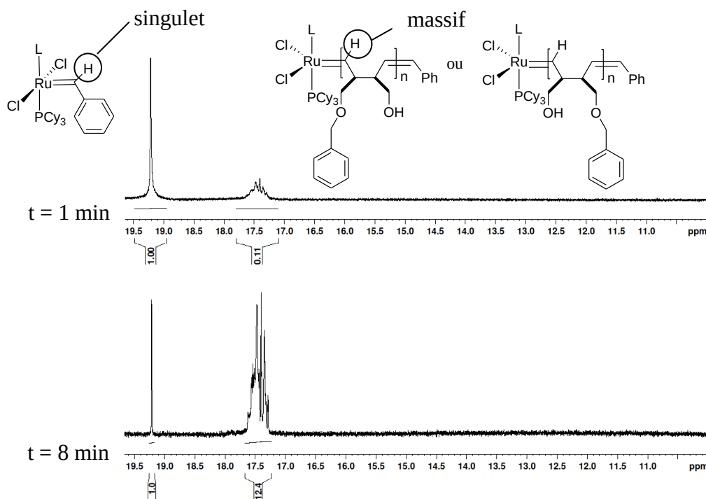
Figure III-8 : Superposition des spectres RMN ^1\text{H} entre \delta = 10 \text{ ppm} et \delta = 19,5 \text{ ppm} des mélanges réactionnels obtenus lors de la ROMP de 1 dans le THF- \text{d}_8 à 50^\circ\text{C} et en utilisant un rapport [\mathbf{1}]_0/[A]_0 de 5 à t = 1 \text{ min} et t = 8 \text{ min} .
