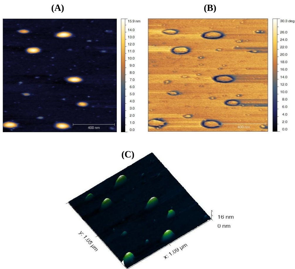
Figure IV-17 : Clichés obtenus par AFM en mode tapping du PBu 85 -g-PLLA 16 (A) mode topographie, (B) mode phase et (C) visualisation 3D.
