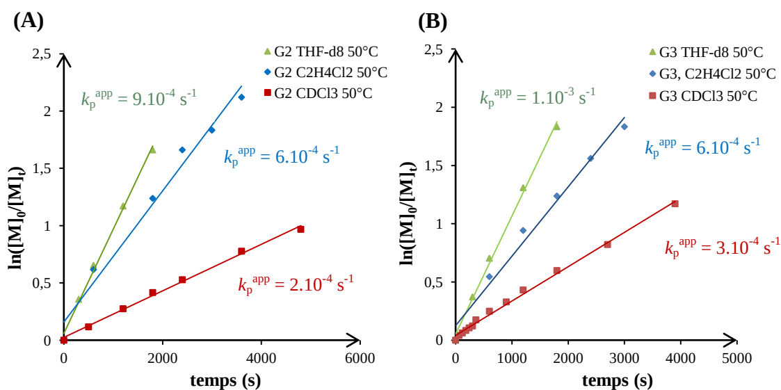
Figure III-7 : Evolutions de \ln([M]_0/[M]_t) en fonction du temps obtenues lors des ROMPs de 1 à 50°C en présence des amorceurs : (A) G2 et (B) G3 en utilisant le THF-d 8 , le \text{C}_2\text{H}_4\text{Cl}_2 et le \text{CDCl}_3 comme solvants et un rapport initial [1]_0/[A]_0 de 100.
