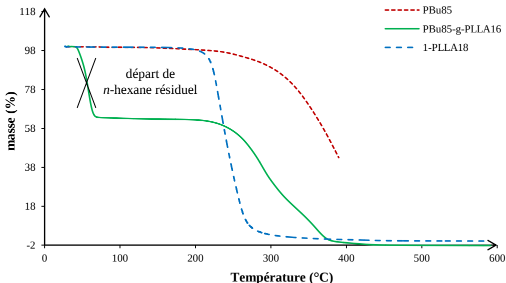
Figure IV-14 : Thermogrammes obtenus en ATG pour le PBu 85 (Tableau IV-1, Entrée 1), le PBu 85 -g-PLLA 16 (Tableau IV-4, Entrée 5) et le PLLA 18 (Tableau IV-4, Entrée 1) avec une vitesse de chauffe de 10°C. min -1 .
