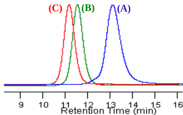
Figure IV-6 : Chromatogrammes SEC du (A) PBu 85 (Tableau IV-1, Entrée 1) et des copolymères greffés (B) PBu 85 -g-P L LA 9 (Tableau IV-2, Entrée 1) et (C) PBu 85 -g-P L LA 16 (Tableau IV-2, Entrée 2) après purification.
