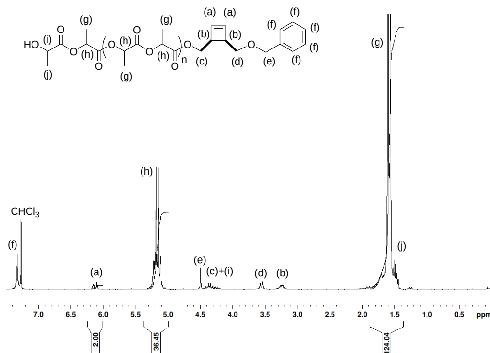
Figure II-3: Spectre RMN ^1\text{H} (200 MHz, \text{CDCl}_3 , 25 °C) du 1-PLLA 18 précipité obtenu par ROP du L-LA dans le DCM à 35°C en utilisant l'inimer 1 comme amorceur et la DMAP comme catalyseur pour un rapport [\text{L-LA}]_0/[\text{OH}]_0 = 14 (Tableau II-1, Entrée 3).
