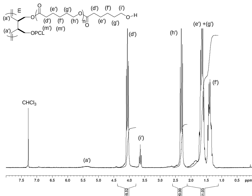
Figure S-4 : Spectre RMN ^1\text{H} (200 MHz, \text{CDCl}_3 , 25 °C) du PBu 10 -g-2-PCL 19 obtenu par ROMP du 2-PCL 19 dans le toluène à 70°C, en utilisant le G2 comme amorceur avec un rapport [2\text{-PCL}_{19}]_0/[G2]_0 = 10 pour un temps de réaction de 3 h (Tableau II-3, Entrée 8).
