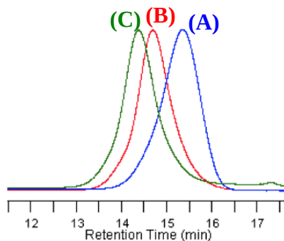
Figure II-4 : Chromatogrammes SEC de (A) 1-P L LA 18 (Tableau II-1, Entrée 3), (B) 1-P L LA 41 (Tableau II-1, Entrée 5), (C) 1-P L LA 76 (Tableau II-1, Entrée 6).
