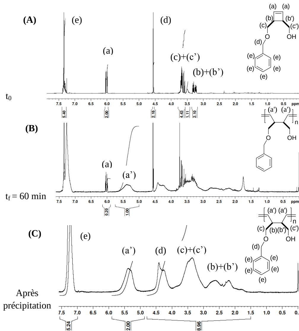
Figure III-1 : Spectre RMN ^1\text{H} (200 MHz, \text{CDCl}_3 , 25 °C) : (A) de l'inimer 1 , (B) du mélange réactionnel obtenu par ROMP de l'inimer 1 dans \text{C}_2\text{H}_4\text{Cl}_2 à 50°C, en utilisant G2 comme amorceur avec un rapport [\text{inimer}]_0/[\text{G2}]_0 = 100 pour un temps de réaction de 60 min et (C) du poly(1,4-butadiène) obtenu après précipitation (Tableau III-1, Entrée 5).
