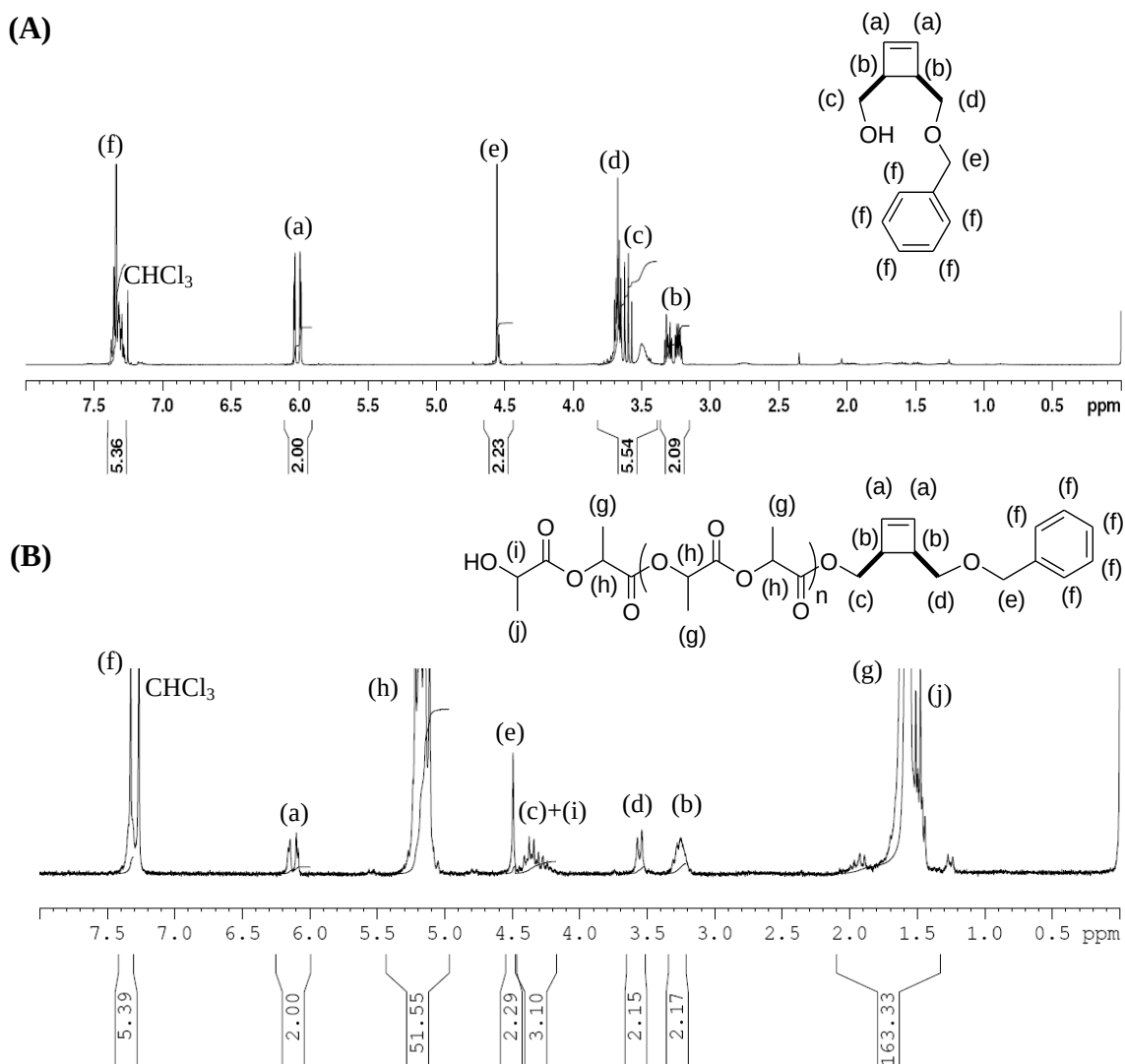
Figure II-1: Spectres RMN ^1\text{H} (200 MHz, \text{CDCl}_3 , 25 °C) de (A) 1 et (B) du mélange réactionnel issu de la ROP du L-LA dans le DCM à 35 °C en utilisant le composé 1 comme amorceur et le TBD comme catalyseur pour un temps de réaction de 1h (Tableau II-1, Entrée 1).
