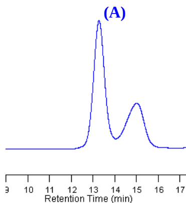
Figure II-11 : Chromatogrammes SEC du (A) PBu 10 -g-1-PCL 16 brut obtenu après 3 h de réaction en utilisant G3 comme amorceur (Tableau II-3, Entrée 1).
