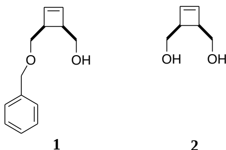
Schéma III-4 : Structures des inimers cis -4-benzyloxyméthyl-3-hydroxyméthylcyclobut-1-ène 1 et cis -3,4-bis(hydroxyméthyl)cyclobutène 2 .
