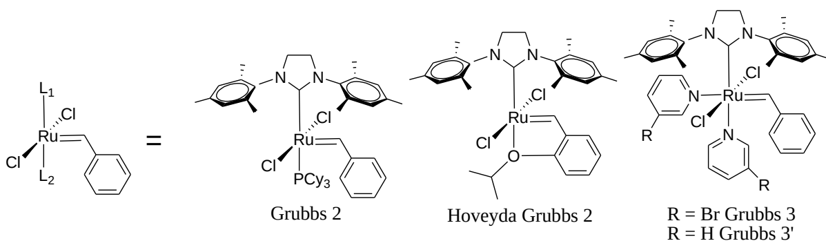
Schéma III-9 : Structures des amorceurs de Grubbs 2, d'Hoveyda Grubbs 2, de Grubbs 3 et de Grubbs 3'.
