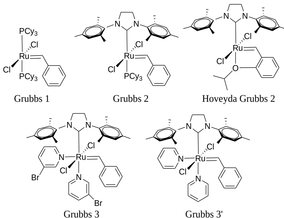
Schéma I-12 : Structures des amorces de Grubbs et Hoveyda Grubbs utilisés en ROMP.
