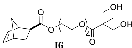
Schéma I-58 : Structure de l' inimer I6 possédant deux extrémités OH.
