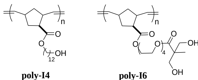
Schéma I-33 : Structures des polymères obtenus par ROMP des inimers I4 et I6 en présence d'amorceur G1.
