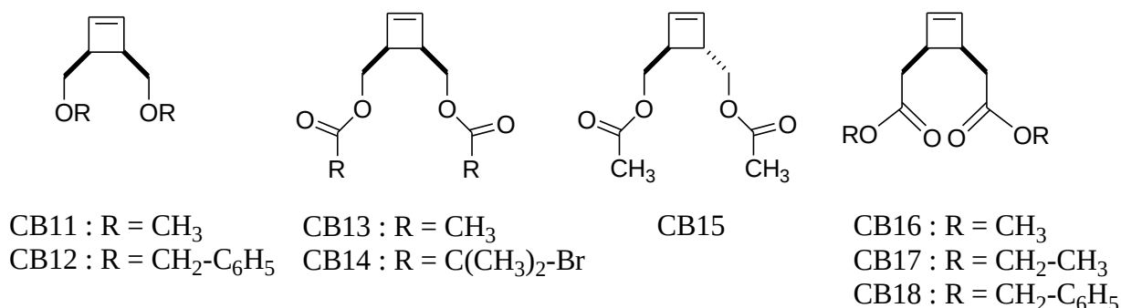
Schéma III-3 : Structures de monomères CB 3,4-disubstitués polymérisés par ROMP.
