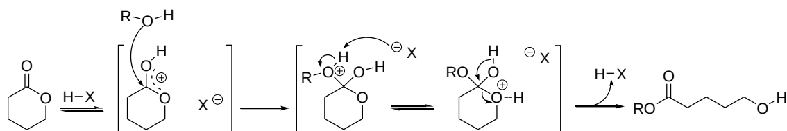
Schéma I-24 : Mécanisme proposé pour la ROP catalysée par des espèces acides.
