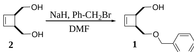
Schéma II-3 : Synthèse du cis -4-benzyloxyméthyl-3-hydroxyméthylcyclobut-1-ène 1 .
