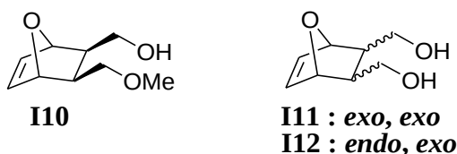
Schéma I-41 : Structures des inimers utilisés pour la synthèse de macromonomères oxaNB-P DLLA .
