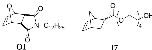
Schéma I-34 : Structures du monomère O1 et de l'inimer I7 , copolymérisés par ROMP de manière séquentielle pour obtenir les squelettes PO1- b -PI7.
