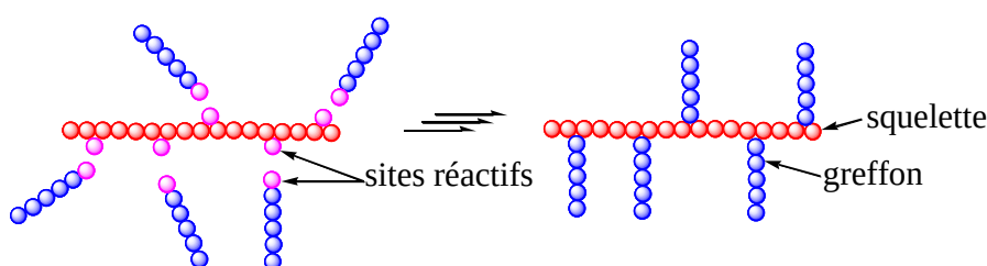
Schéma I-1 : Représentation schématique de la synthèse d'un copolymère greffé par la méthode grafting onto .
