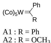
Schéma I-8 : Structures des premiers amorceurs bien définis à base de tungstène A1 et A2, utilisés en ROMP.
