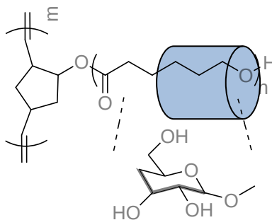
PNB-g-PCL 1 -CDIs
