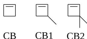
Schéma III-1 : Structures des monomères CB, CB1 et CB2 polymérisés par ROMP.
