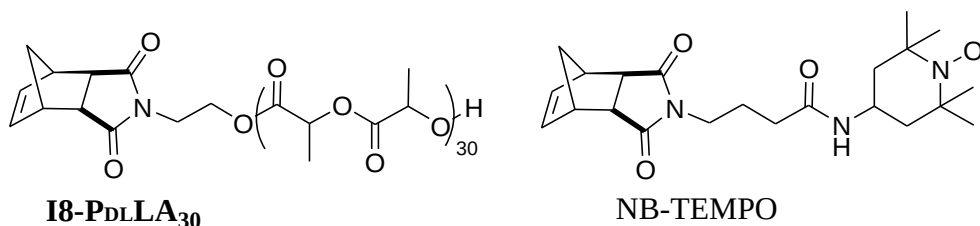
Schéma I-37 : Structures des macromonomères 18-PdLLA 30 et du monomère NB-TEMPO copolymérisés de manière séquentielle par ROMP.
