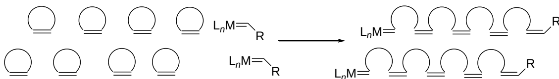
Schéma I-4 : Principe de formation de macromolécules par ROMP [13,14] .
