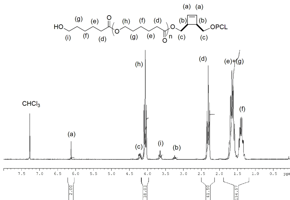
Figure S-2 : Spectre RMN ^1\text{H} (200 MHz, \text{CDCl}_3 , 25 °C) du 2-PCL 19 précipité obtenu par ROP de L ' \epsilon -CL dans le THF à 25°C en utilisant l'inimer 2 comme amorceur et du TBD comme catalyseur pour un rapport [\epsilon\text{-CL}]_0/[\text{OH}]_0 = 18 (Tableau II-2, Entrée 5).
