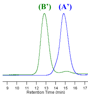
Figure II-12 : Chromatogrammes SEC du (A') 1-PCL 16 précipité (Tableau II-2, Entrée 1) et de (B') PBu 10 -g-1-PCL 16 brut après 3 h de réaction en utilisant G2 comme amorceur (Tableau II-3, Entrée 2).
