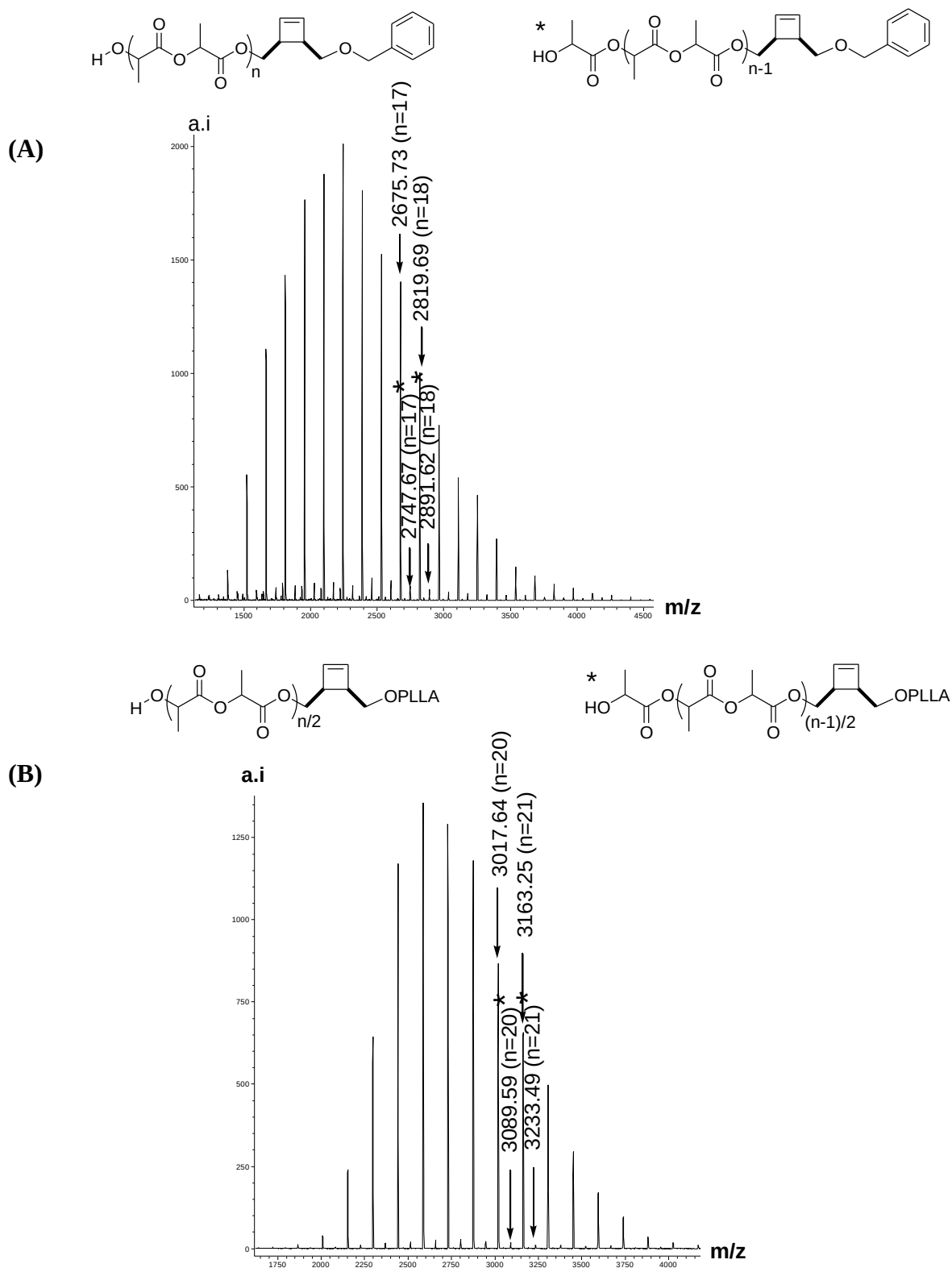
Figure II-6 : Spectres de masse MALDI-TOF (matrice : trans -2-[3-(4- tert -butylphényl)-2-méthyl-2-propénylidène]malononitrile + trifluoroacétate de sodium (DCTB + NaTFA) des macromonomères (A) 1- Pt LA 18 et (B) 2- Pt LA 20 .
