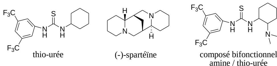
Schéma I-20 : Structures de composés utilisés en tant que (co)catalyseurs pour la ROP.
