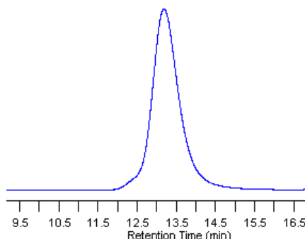
Figure III-3 : Chromatogramme SEC du poly(1,4-butadiène) brut obtenu par ROMP de l'inimer 1 dans C_2H_4Cl_2 à 50^\circ C , en utilisant G2 comme amorceur avec un rapport [1]_0/[G2]_0 = 100 pour un temps de réaction de 1 h.
