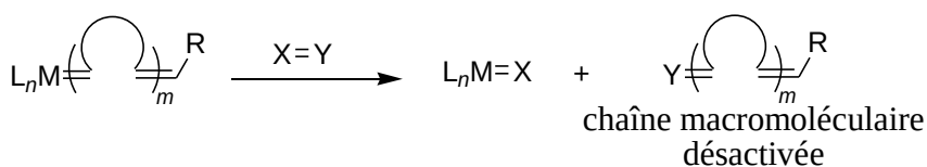
Schéma I-6 : Mécanisme de la ROMP.
