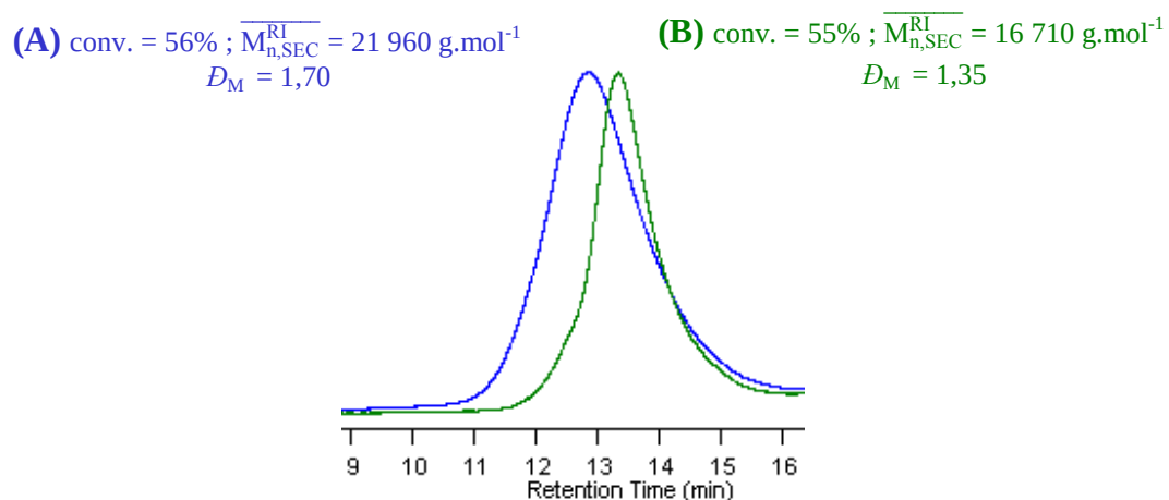
Figure III-10 : Chromatogrammes SEC de poly(1,4-butadiène)s bruts obtenus lors des ROMPs de 1 à 25°C en présence de G2 pour des rapports [inimer]_0/[A]_0=100 en utilisant le (A) CDCl_3 et le (B) THF-d_8 comme solvant.
