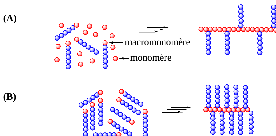
Schéma I-3 : Représentation schématique de (A) la copolymérisation d'un macromonomère avec un comonomère conventionnel conduisant à un copolymère greffé, (B) l'homopolymérisation de macromonomères conduisant à un polymacromonomère.
