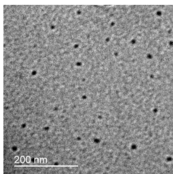
Figure IV-19 : Cliché obtenu par TEM d'un film PBu 200 -g-PCL 48 .
