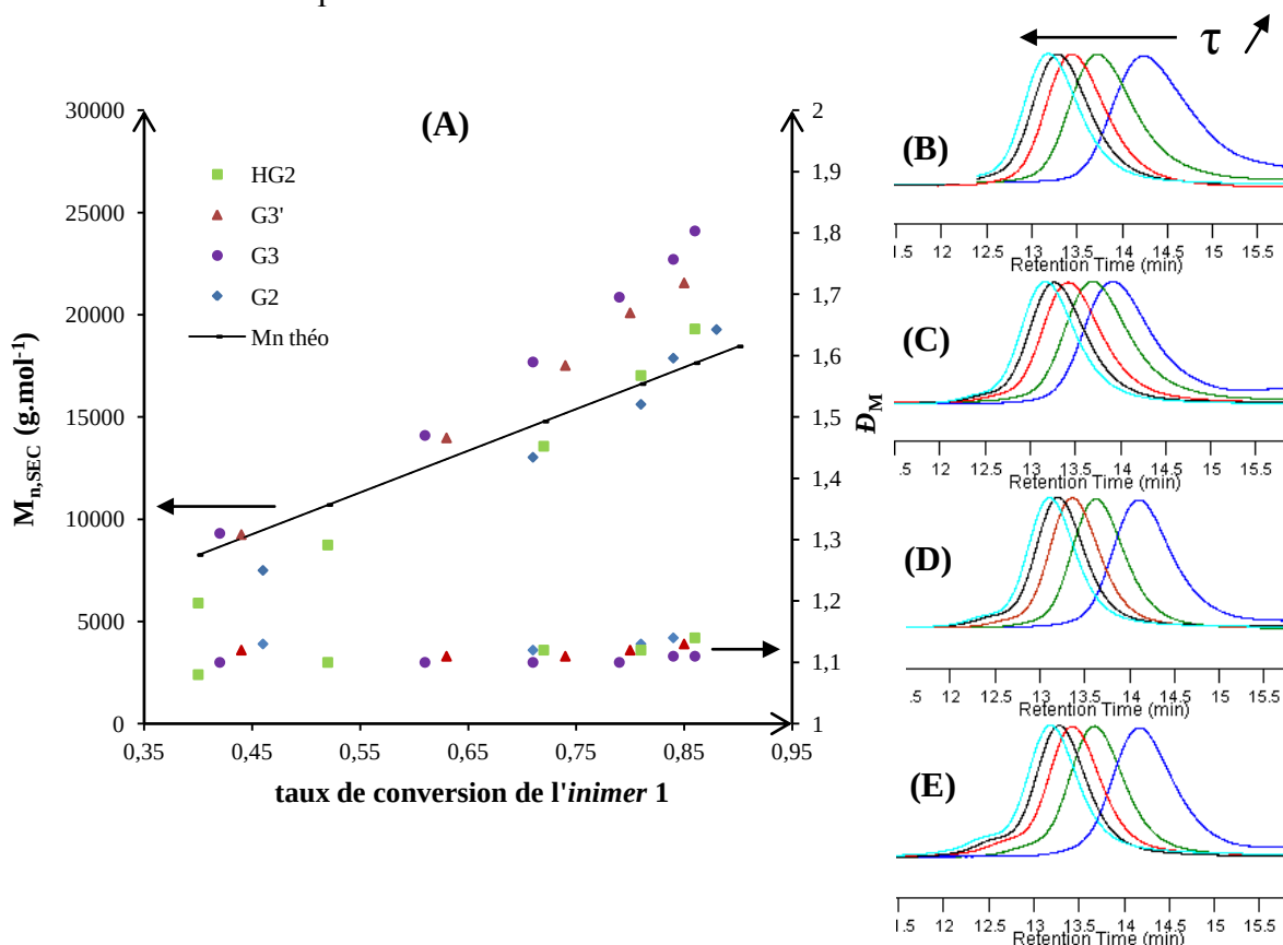
Figure III-5 : (A) Evolution des \overline{M}_{n,SEC}^{RI} en fonction de la conversion de 1 et chromatogrammes SEC pour les poly(1,4-butadiène)s bruts obtenus à différents taux de conversion, en utilisant l'amorceur (B) G2 (C) G3 (D) G3' et (E) HG2 pour les ROMPs de 1 à 50°C dans le C_2H_4Cl_2 avec un rapport [1]_0/[A]_0 de 100.
