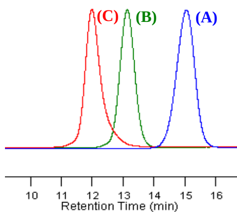
Figure II-23 : Chromatogrammes SEC du (A) 2-PLLA 20 précipité (Tableau II-1, Entrée 7), du (B) PBu 10 -g-2-PLLA 20 (Tableau II-3, Entrée 18) et du (C) PBu 50 -g-2-PLLA 20 (Tableau II-3, Entrée 19) après purification.
