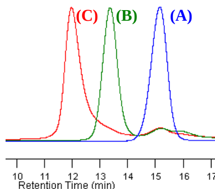
Figure II-21 : Chromatogrammes SEC du (A) 2-P L LA 20 précipité (Tableau II-1, Entrée 7), du (B) PBu 10 -g-2-P L LA 20 brut après 3 h de réaction (Tableau II-3, Entrée 18) et du (C) PBu 50 -g-2-P L LA 20 brut après 3 h de réaction (Tableau II-3, Entrée 19).
