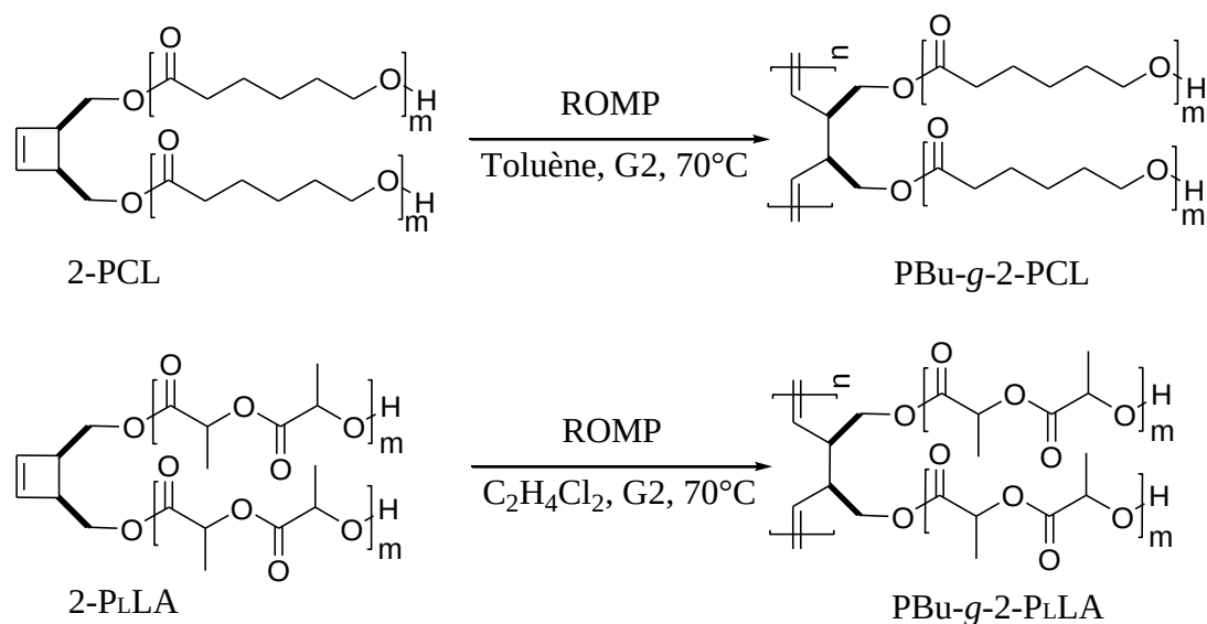
Schéma II-7: ROMP des macromonomères 2-PCL et 2-PLLA en présence de l'amorceur de Grubbs 2.
