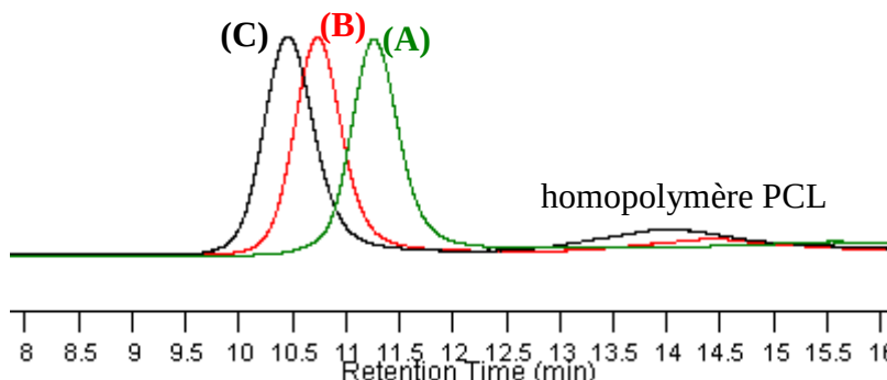
Figure IV-8 : Chromatogrammes SEC du (A) PBu 85 -g-PCL 18 brut (Tableau IV-3, Entrée 1), du (B) PBu 85 -g-PCL 35 brut (Tableau IV-3, Entrée 2) et du (C) PBu 85 -g-PCL 45 (Tableau IV-3, Entrée 3), obtenus par ROP de l' \epsilon -CL en utilisant le PBu 85 comme macroamorceur et le TBD comme catalyseur.
