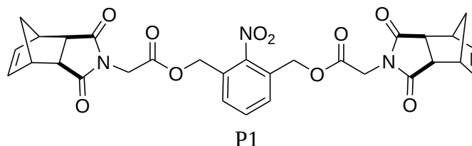
Schéma I-55 : Structure du composé P1, agent de réticulation photodégradable en ROMP.
