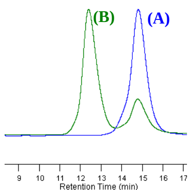
Figure II-18 : Chromatogrammes SEC du (A) 1-PCL 38 précipité (Tableau II-2, Entrée 3) et du (B) PBu 10-g-1-PCL 42 brut après 3 h de réaction (Tableau II-3, Entrée 6).
