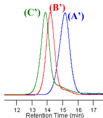
Figure II-5 : Chromatogrammes SEC de (A') 2-P L LA 20 (Tableau II-1, Entrée 7), (B') 2-P L LA 40 (Tableau II-1, Entrée 8), (C') 2-P L LA 77 (Tableau II-1, Entrée 9).
