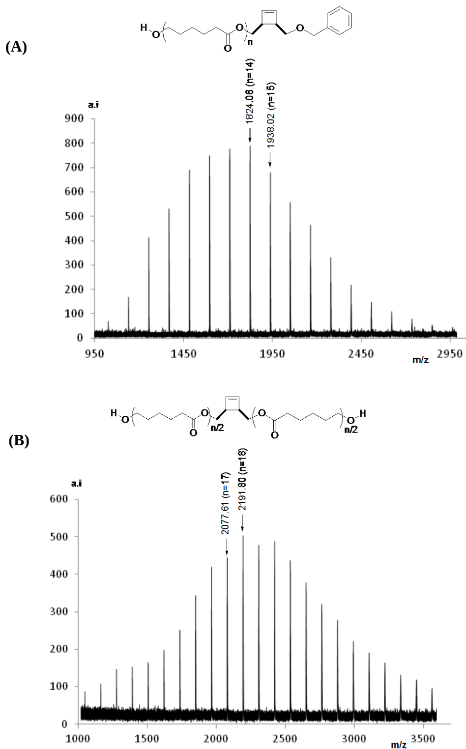
Figure II-10 : Spectres MALDI-TOF (matrice : DCTB + NaTFA) des macromonomères (A) 1-PCL 16 et (B) 2-PCL 19 .
