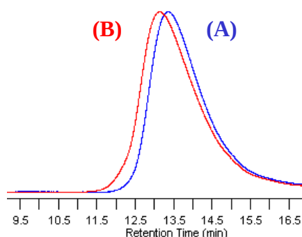
Figure III-2 : Chromatogrammes SEC des poly(1,4-butadiène)s bruts obtenus par ROMP de l'inimer 1 dans C 2 H 4 Cl 2 à 50 °C en utilisant l'amorceur Nolan avec un rapport [1]_0/[Nolan]_0 = 100 (A) après 1 h de réaction et, (B) après 4 h de réaction.
