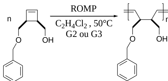
Schéma IV-1 : ROMP de l' inimer 1 en présence des amorceurs G2 ou G3.
