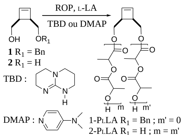
Schéma II-4 : Synthèse des macromonomères 1-P L LA et 2-P L LA.
