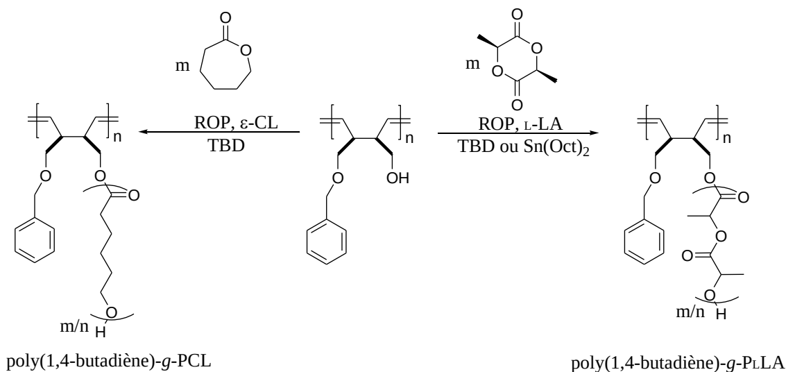
Schéma IV-3 : Synthèse des copolymères greffés PBu- g -PCL et PBu- g -PLLA à partir des squelettes PBu, utilisés en tant que macroamorceurs.
