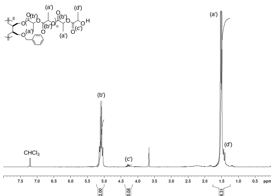
Figure S-3 : Spectre RMN ^1\text{H} (200 MHz, \text{CDCl}_3 , 25 °C) du PBu 10-g-1-PLLA 24 obtenu par ROMP du 1-PLLA 24 dans \text{C}_2\text{H}_4\text{Cl}_2 à 70°C, en utilisant G2 comme amorceur avec un rapport [1\text{-PLLA}_{24}]_0/[G2]_0 = 10 pour un temps de réaction de 3 h (Tableau II-3, Entrée 14).
