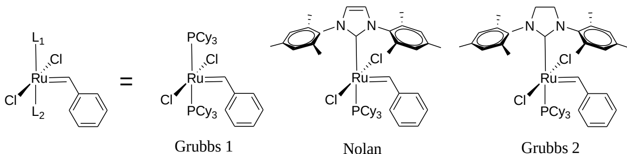
Schéma III-6 : Structures des amorceurs à base de ruthénium utilisés : Grubbs 1, Nolan et Grubbs 2.
