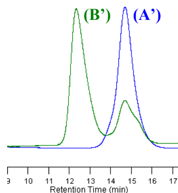
Figure II-19 : Chromatogrammes SEC du (A') 1-PtLA 41 précipité (Tableau II-1, Entrée 5) et du (B') PBu 10-g-1-PtLA 41 brut après 3 h de réaction (Tableau II-3, Entrée 16).
