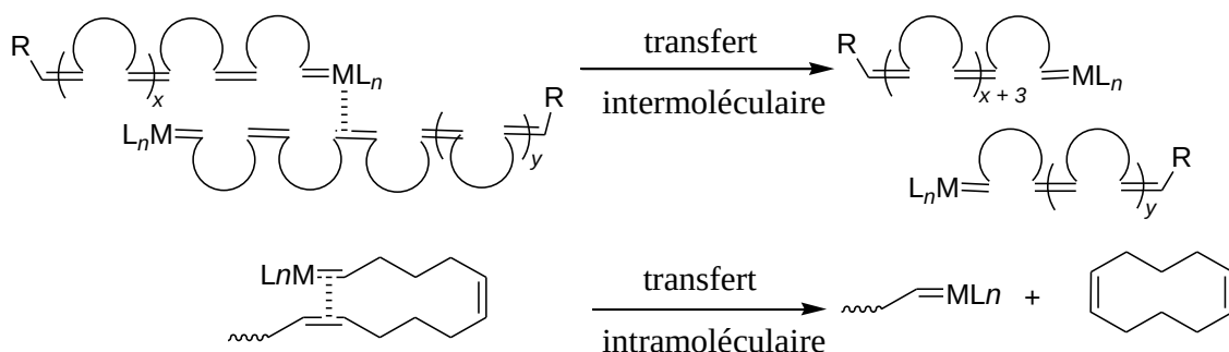
Schéma I-7 : Représentation des réactions de transferts intramoléculaire et intermoléculaire se produisant au cours des ROMP.
