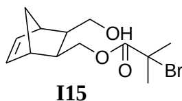
Schéma I-48 : Structure de l' inimer trifonctionnel I15 , susceptible d'amorcer une ROP et une ATRP et possédant une double liaison polymérisable en ROMP.
