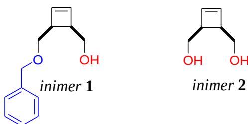
Schéma 1 : Structures des inimers 1 et 2 , précurseurs de macromonomères polymérisables en ROMP et de macroamorceurs poly(1,4-butadiène) en ROP.
