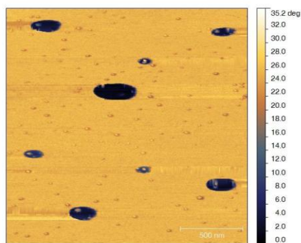
Figure IV-18 : Cliché obtenu par AFM en mode tapping du PBu 200 -g-PtLA 9 : mode phase.
