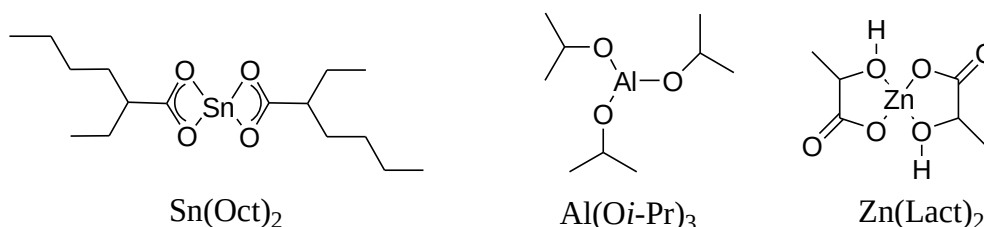
Schéma I-14 : Structures du bis(2-éthylhexanoate d'étain), de l'isopropoxyde d'aluminium et du lactate de zinc utilisés en ROP.
