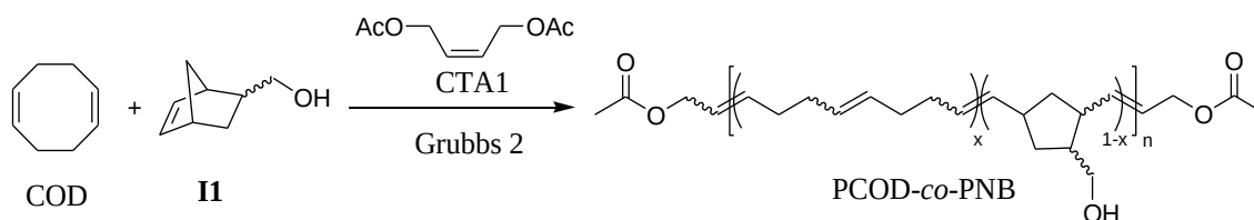
Schéma I-40 : Schéma de synthèse du squelette PCOD-co-PNB.
