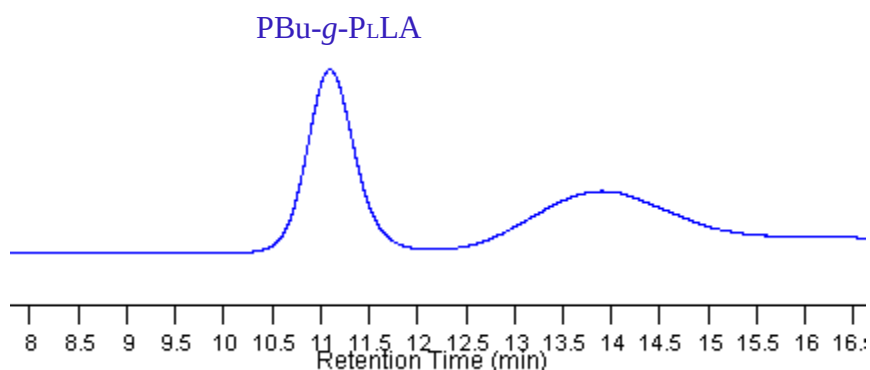
Figure IV-4 : Chromatogramme SEC du mélange réactionnel issu de la ROP du L-LA, en utilisant le squelette PBu 85 comme macroamorceur et le TBD comme catalyseur avec un rapport [L-LA]_0/[OH]_0 = 35 .
