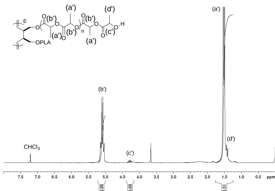
Figure II-22 : Spectre RMN ^1\text{H} (200 MHz, \text{CDCl}_3 , 25 °C) du PBu 10 -g-2-PLLA 20 , obtenu par ROMP du 2-PLLA 20 dans \text{C}_2\text{H}_4\text{Cl}_2 à 70°C, en utilisant G2 comme amorceur avec un rapport [\text{2-PLLA}_{20}]_0/[\text{G2}]_0 = 10 pour un temps de réaction de 3 h ( Tableau II-3, Entrée 18 ).
