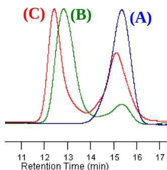
Figure II-17 : Chromatogrammes SEC du (A) 1-P L LA 24 précipité (Tableau II-1, Entrée 4), du (B) PBu 10 -g-1-P L LA 24 brut après 3 h de réaction (Tableau II-3, Entrée 14) et du (C) PBu 50 -g-1-P L LA 24 brut après 3 h de réaction (Tableau II-3, Entrée 15).
