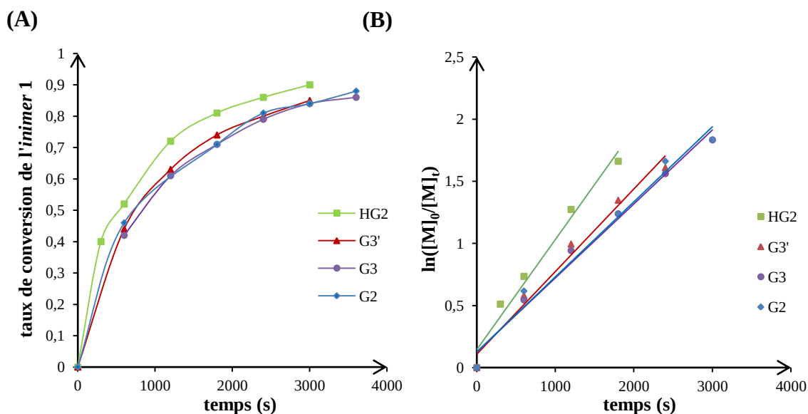
Figure III-4 : (A) Variation du taux de conversion de l'inimer 1 en fonction du temps et, (B) variation de \ln([M]_0/[M]_t) en fonction du temps pour les ROMPs de l'inimer 1 à 50°C dans C_2H_4Cl_2 en présence des amorceurs G2, HG2, G3 et G3' avec un rapport [1]_0/[A]_0 de 100.
