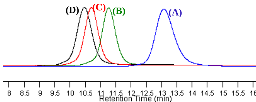
Figure IV-9 : Chromatogrammes SEC du (A) \text{PBU}_{85} (Tableau IV-1, Entrée 1), du (B) \text{PBU}_{85}\text{-g-PCL}_{18} (Tableau IV-3, Entrée 1), du (C) \text{PBU}_{85}\text{-g-PCL}_{35} (Tableau IV-3, Entrée 2) et du (D) \text{PBU}_{85}\text{-g-PCL}_{45} (Tableau IV-3, Entrée 3).
