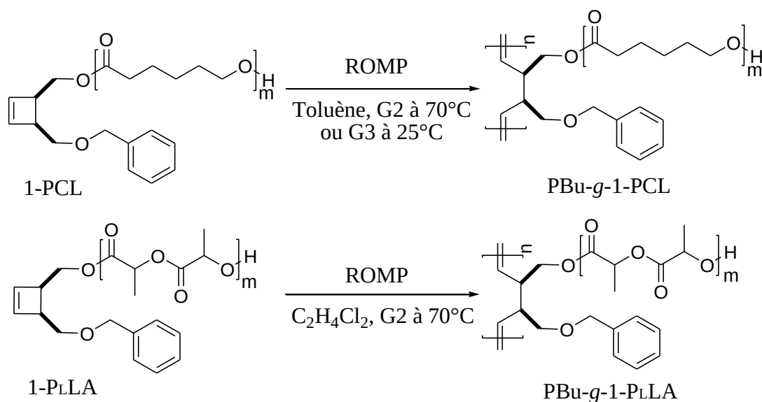
Schéma II-6 : ROMP des macromonomères 1-PLLA et 1-PCL en présence d'amorceurs de Grubbs 2 ou de Grubbs 3.
