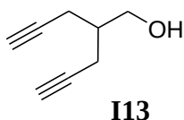
Schéma I-43 : Structure de l'inimer I13 utilisé comme amorceur pour la synthèse des macromonomères I13-P L LA 18 et I13-PCL 26 .
