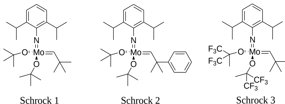
Schéma I-11 : Structures des amorceurs de Schrock 1, Schrock 2 et Schrock 3 utilisés en ROMP.
