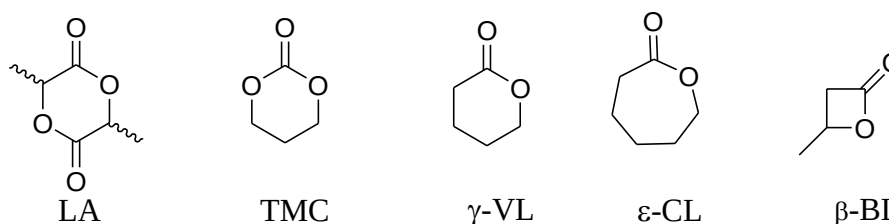
Schéma I-13 : Structures de composés cycliques polymérisables par ROP.
