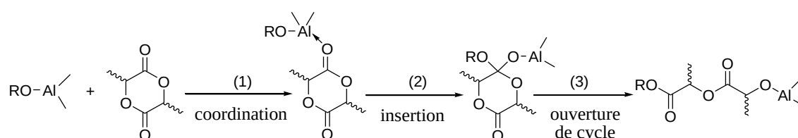
Schéma I-16 : Mécanisme de la ROP catalysée par des alcoxydes d'aluminium.
