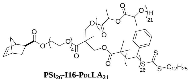
Schéma I-51 : Structure du macromonomère PSt 26 -I16-PDLA 21 synthétisé par combinaison one-pot RAFT/ROP.
