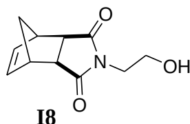
Schéma I-60 : Structure de l'inimer I8 , utilisé en tant qu'amorceur pour synthétiser les macromonomères I8-P DL LA .
