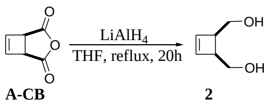
Schéma II-2 : Synthèse du cis -3,4-bis(hydroxyméthyl)cyclobutène 2 .
