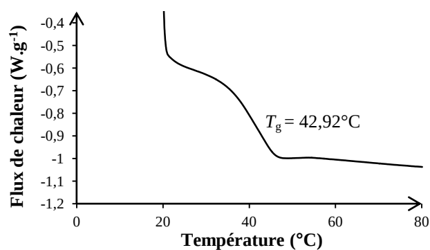
Figure IV-2 : Thermogramme obtenu en DSC pour le PBU 85 (Tableau IV-1, Entrée 1) avec une vitesse de chauffe et de refroidissement de 5 °C.min -1 .
