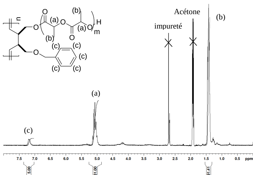
Figure IV-7 : Spectre RMN 1 H (200 MHz, Acétone-d 6 , 25 °C) du PBu 85 -g-P L LA 16 purifié obtenu par ROP du L-LA dans le DCM à 25 °C en utilisant le PBu 85 comme macroamorceur et le TBD comme catalyseur pour un temps de réaction de 1 h (Tableau IV-2, Entrée 2).
