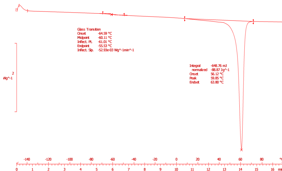
Figure S2 : Thermogramme obtenu en DSC pour le macromonomère 1-PCL 38 (Tableau IV-5, Entrée 2) avec une vitesse de chauffe et de refroidissement de 10 °C.min -1 .
