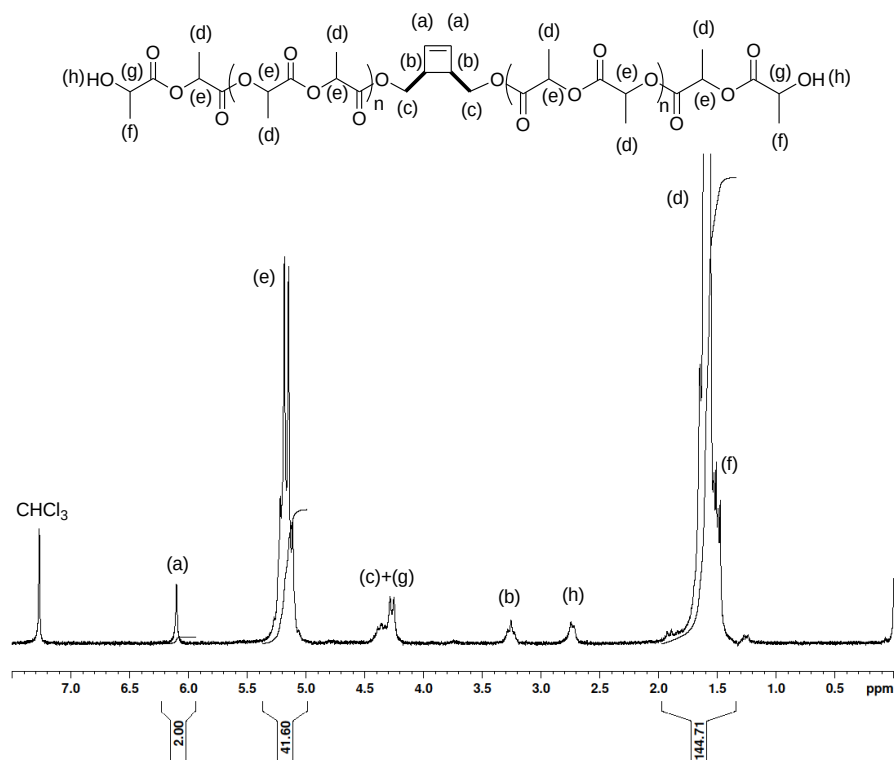
Figure S-1: Spectre RMN ^1\text{H} (200 MHz, \text{CDCl}_3 , 25 °C) du 2-PLA 20 précipité obtenu par ROP du L-LA dans le DCM à 35°C en utilisant l'inimer 2 comme amorceur et la DMAP comme catalyseur pour un rapport [\text{L-LA}]_0/[\text{OH}]_0 = 14 (Tableau II-1, Entrée 7).
