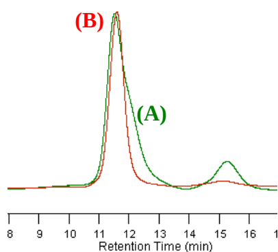
Figure II-14 : Chromatogrammes SEC du (A) PBu 50 - g -1-PCL 16 brut après 3 h de réaction (Tableau II-3, Entrée 3) et du (B) PBu 50 - g -1-PCL 16 brut après 3 h de réaction (Tableau II-3, Entrée 4).
