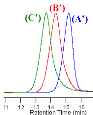
Figure II-8 : Chromatogrammes SEC de (A') 2-PCL 19 (Tableau II-2, Entrée 5), (B') 2-PCL 47 (Tableau II-2, Entrée 6), (C') 2-PCL 81 (Tableau II-2, Entrée 7).
