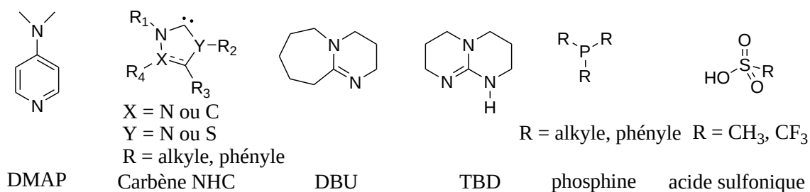
Schéma I-15 : Structures de catalyseurs organiques couramment utilisés pour la ROP organocatalysée.
