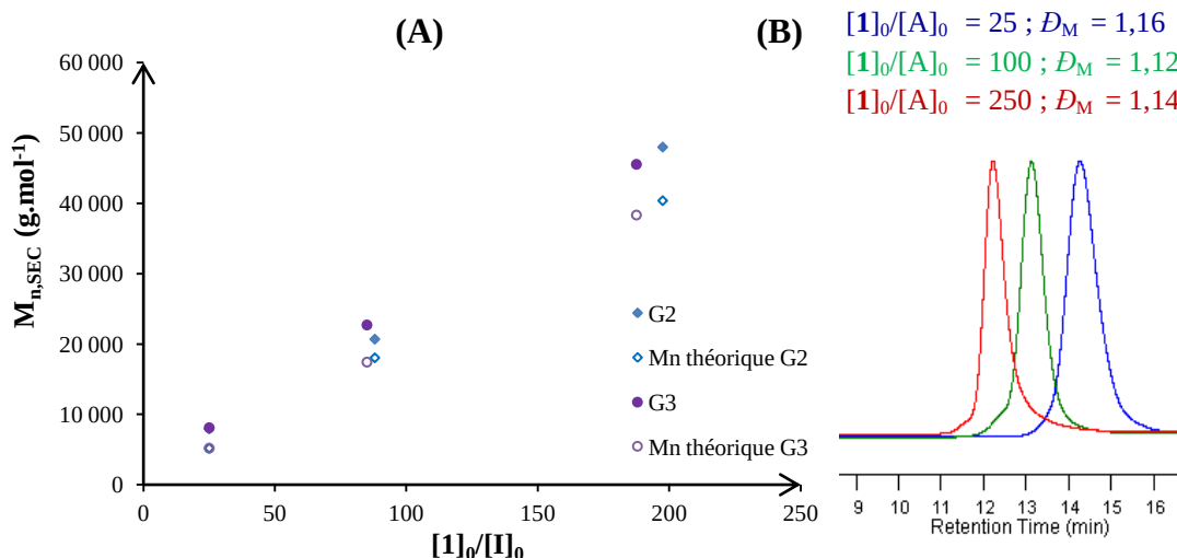
Figure III-6 : (A) Evolution des \overline{M}_{n,SEC}^{RI} en fonction du rapport [1]_0/[A]_0 pour les ROMPs de 1 à 50°C dans le C_2H_4Cl_2 en présence de G2 ou G3 et (B) chromatogrammes SEC des poly(1,4-butadiène)s précipités obtenus à l'issue des ROMPs de 1 à 50°C dans le C_2H_4Cl_2 en présence de G3 pour des rapports [inimer]_0/[A]_0 = 25, 100 et 250 (Tableau III-3, Entrées 4, 6 et 8).
