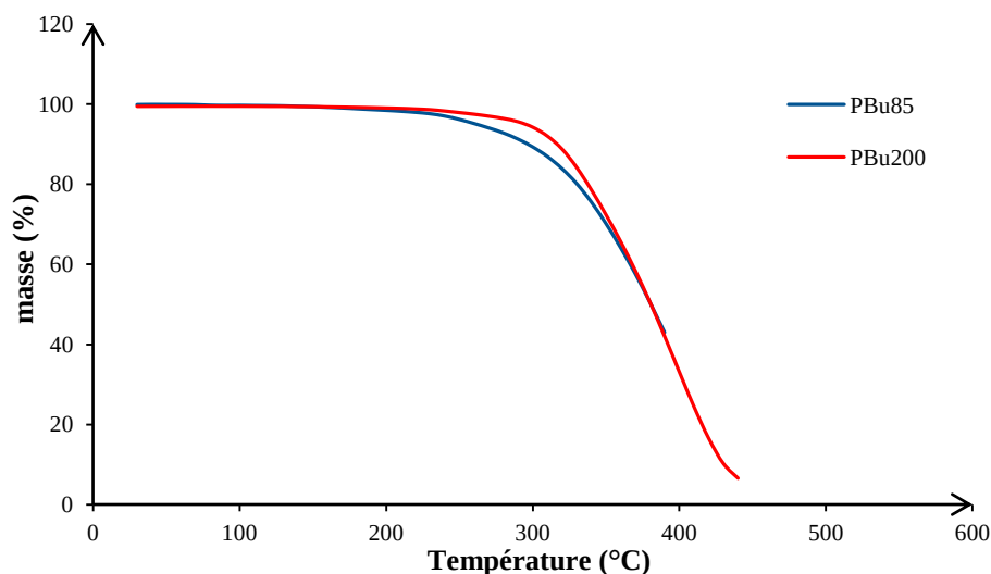
Figure IV-3 : Thermogrammes obtenus en ATG pour le PBu 85 et le PBu 200 (Tableau IV-1, Entrées 1 et 3), avec une vitesse de chauffe de 10°C. min -1 .
