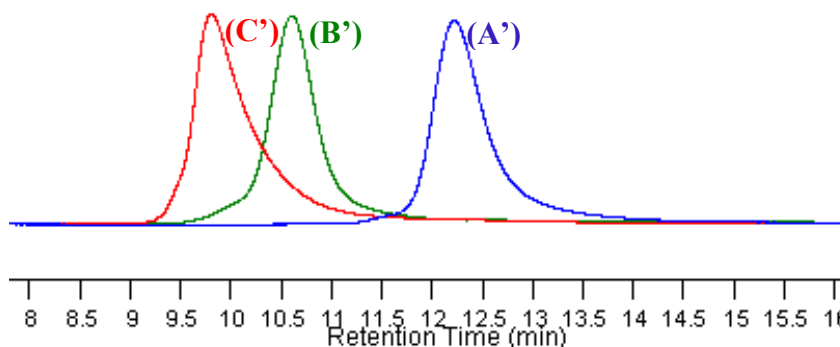
Figure IV-10 : Chromatogrammes SEC du (A') \text{PBU}_{200} (Tableau IV-1, Entrée 3), du (B') \text{PBU}_{200}\text{-g-PCL}_{18} (Tableau IV-3, Entrée 4) et (C') \text{PBU}_{200}\text{-g-PCL}_{48} (Tableau IV-3, Entrée 5).
