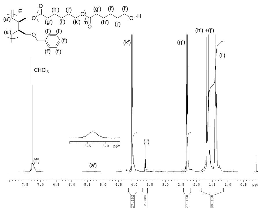
Figure II-13 : Spectre RMN ^1H (200 MHz, CDCl_3 , 25 °C) du PBu10-g-1-PCL 16 obtenu par ROMP du 1-PCL 16 dans le toluène à 70°C, en utilisant G2 comme amorceur avec un rapport [1-PCL_{16}]_0/[G2]_0 = 10 pour un temps de réaction de 3 h (Tableau II-3, Entrée 2).
