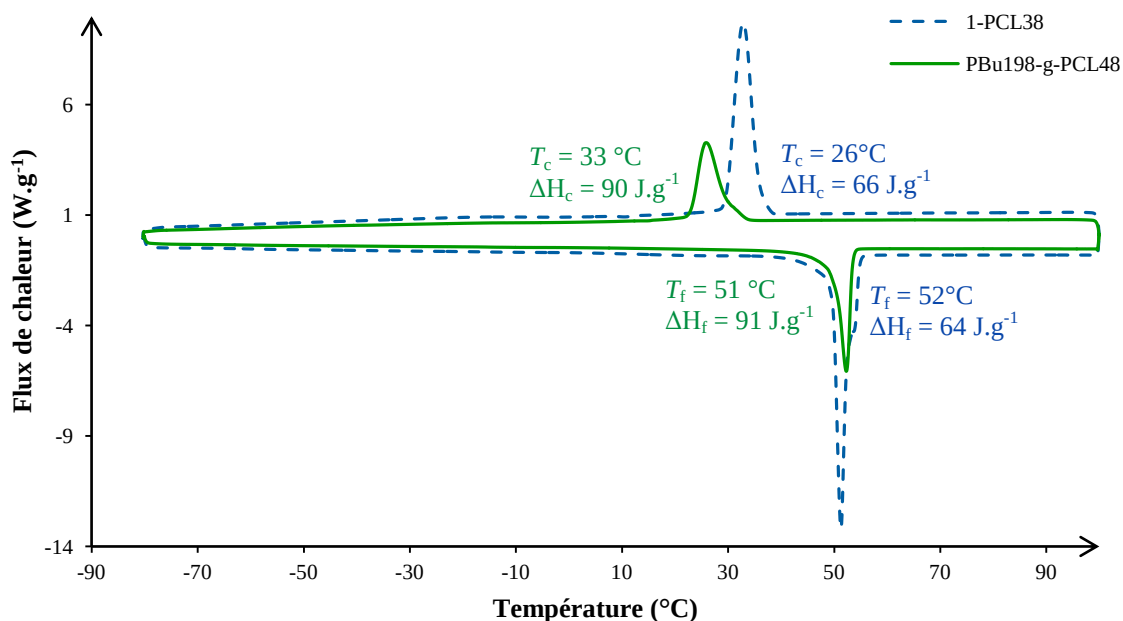
Figure IV-15 : Thermogrammes obtenus en DSC pour le copolymère greffé PBu 200 - g -PCL 48 (Tableau IV-5, Entrée 10) et pour le macromonomère 1-PCL 38 (Tableau IV-5, Entrée 2) avec une vitesse de chauffe et de refroidissement de 5 °C.min -1 .
