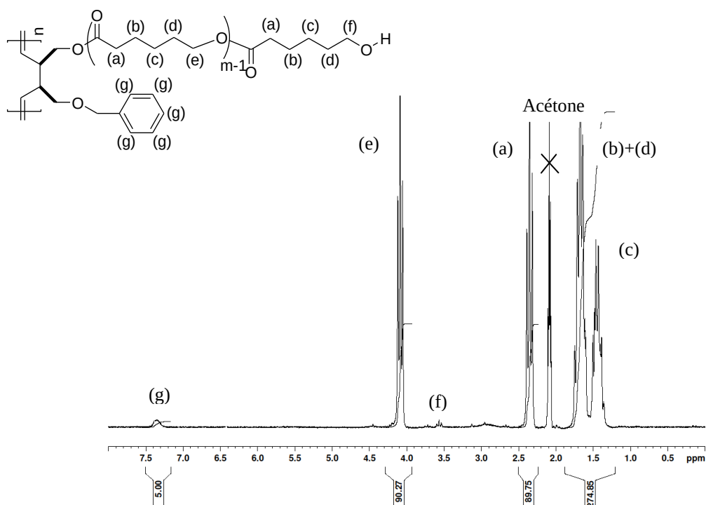
Figure IV-11 : Spectre RMN ^1\text{H} (200 MHz, Acétone- d_6 , 25 °C) du PBu 85 -g-PCL 45 purifié obtenu par ROP de l' \epsilon -CL dans le THF à 25 °C en utilisant le PBu 85 comme macroamorceur et le TBD comme catalyseur pour un temps de réaction de 16 h (Tableau IV-3, Entrée 3).
