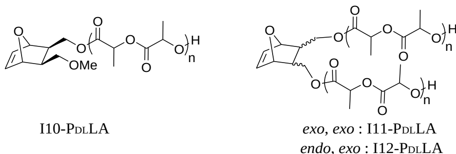
Schéma I-42 : Structures des macromonomères obtenus par ROP du DL-LA en présence de Sn(Oct)_2 à partir des inimers I10 , I11 et I12 .
