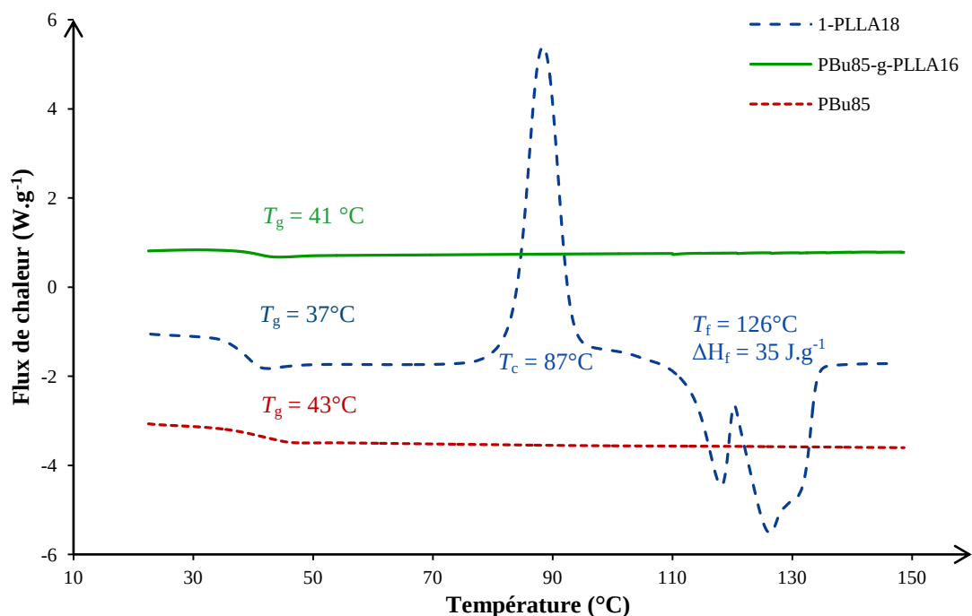
Figure IV-13 : Thermogrammes obtenus en DSC pour le squelette PBu 85 (Tableau IV-1, Entrée 1), pour le copolymère greffé PBu 85 - g -PLLA 16 (Tableau IV-4, Entrée 5) et pour le macromonomère 1-PLLA 18 (Tableau IV-4, Entrée 1) avec une vitesse de chauffe et de refroidissement de 5 °C.min -1 .
