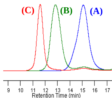
Figure II-16 : Chromatogrammes SEC du (A) 1-PCL 16 précipité (Tableau II-2, Entrée 1), (B) PBu 10 -g-1-PCL 16 brut après 3 h de réaction (Tableau II-3, Entrée 2) avec [1\text{-PCL}_{16}] = 0,01 \text{ mol.L}^{-1} et (C) PBu 50 -g-1-PCL 16 brut après 3 h de réaction (Tableau II-3, Entrée 4) avec [1\text{-PCL}_{16}] = 0,04 \text{ mol.L}^{-1} .
