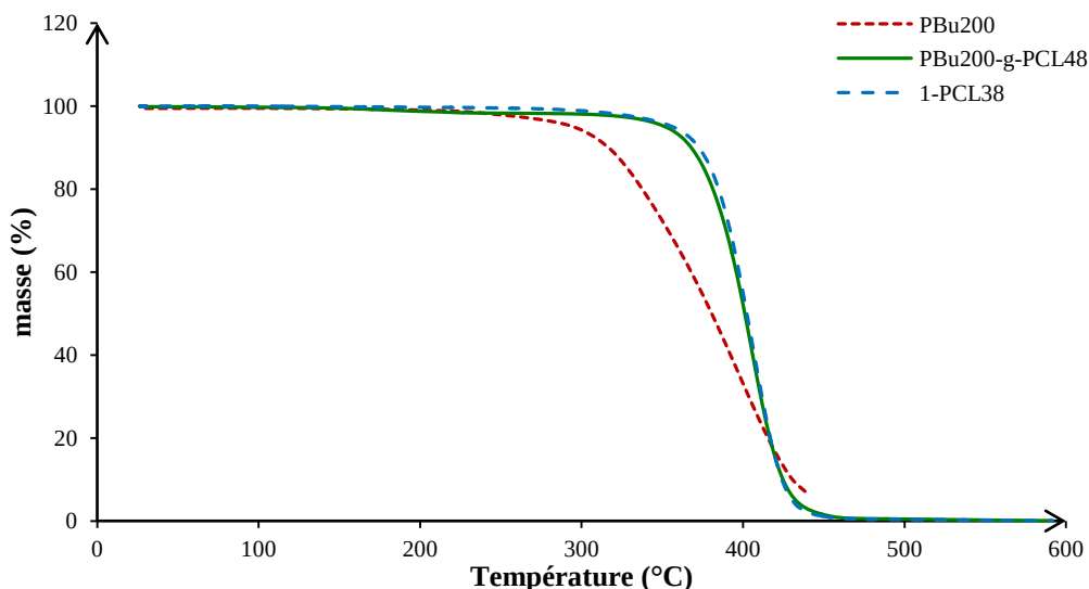
Figure IV-16 : Thermogrammes obtenus en ATG pour le PBu 200 (Tableau IV-1, Entrée 3), le PBu 200 -g-PCL 48 (Tableau IV-5, Entrée 10) et le PCL 38 (Tableau IV-5, Entrée 2) avec une vitesse de chauffe de 10°C. min -1 .
