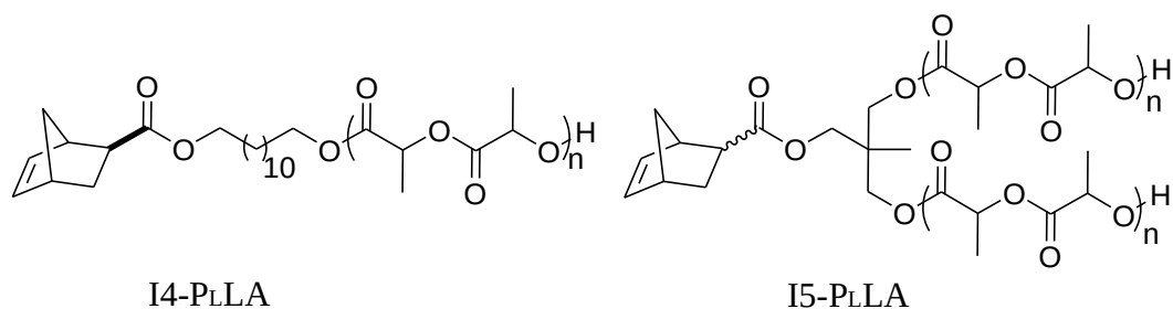
Schéma I-32 : Structures des macromonomères obtenus par ROP du L-lactide en présence du catalyseur \text{Sn}(\text{Oct})_2 à partir de I4 et I5 .
