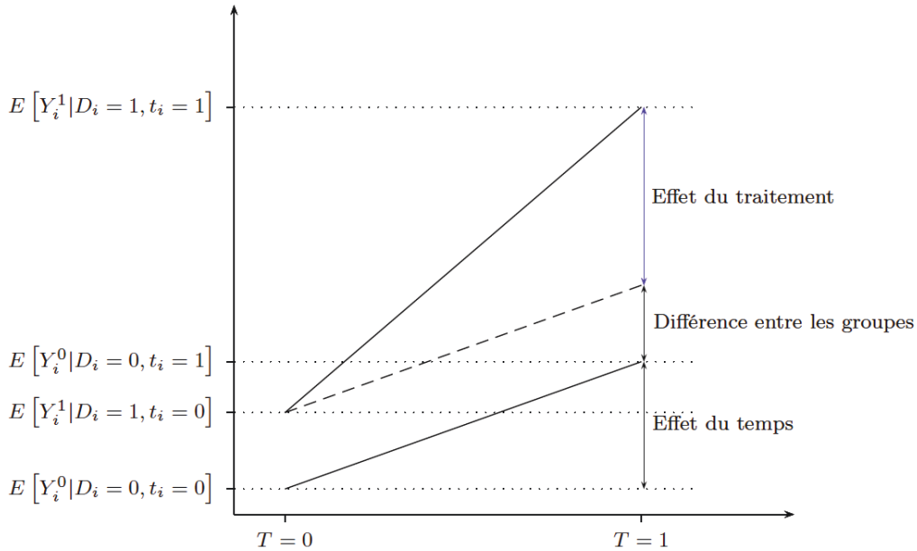
FIGURE 5.1 – Doubles différences
