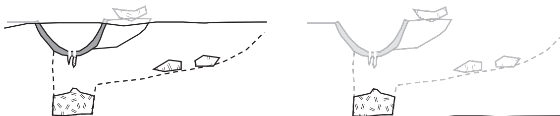
Figure III.48. Hypothèse de fonctionnement des bas fourneaux à scorie coulée par égouttage (SCe)
