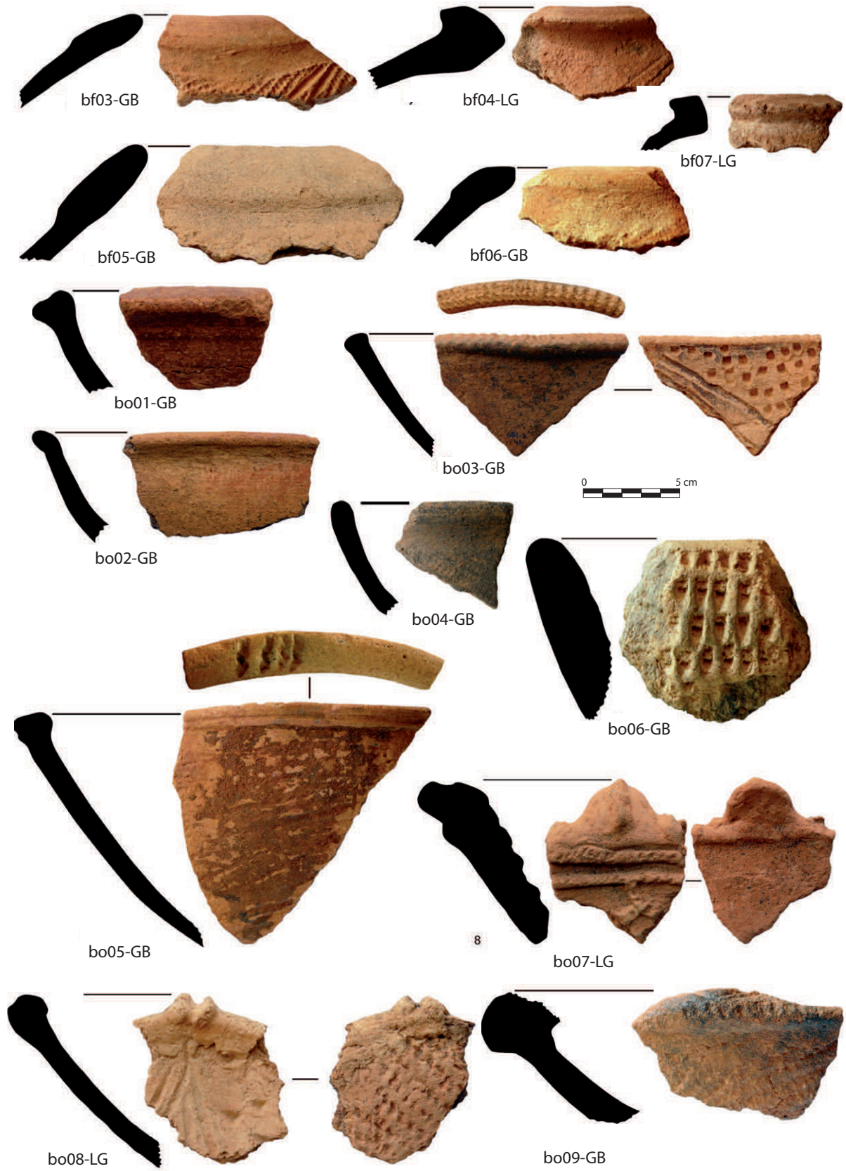
Figure III.5. Mobilier céramique : bords fermés (bf) et bords ouverts (bo)
