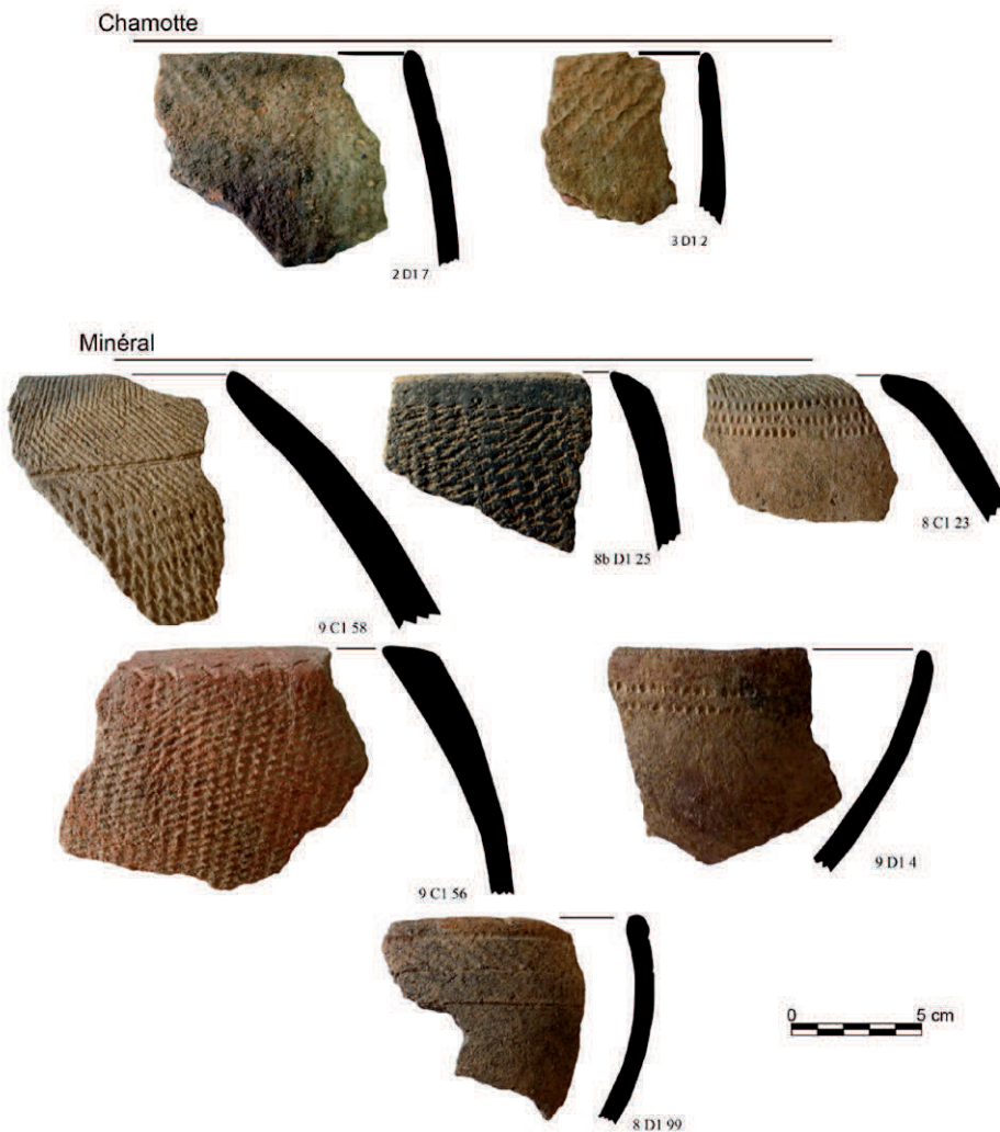
Figure II.5. Exemples de tessons (bords) à dégraissant à chamotte et minéral provenant du front de carrière de Kirkisoy
