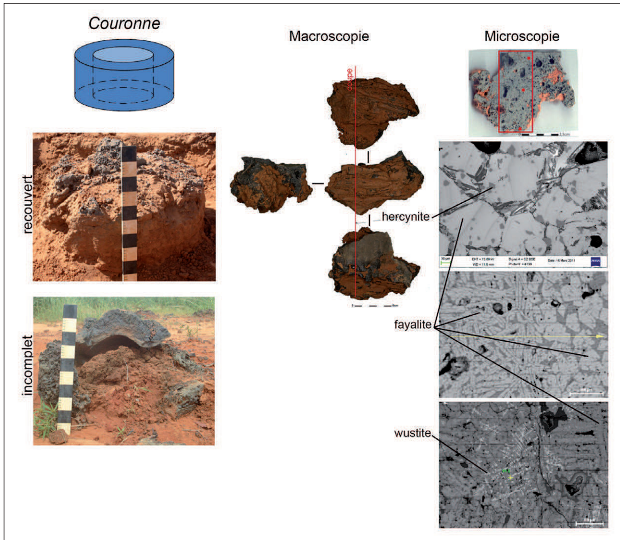
Figure III.25. Les scories en anneau
