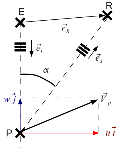
FIGURE 3.9 – Schéma de fonctionnement de la mesure de vitesse par les profilers acoustiques (policopié du cours Flow Measurement Science , D. Hurther). E représente la céramique émettrice, P une particule (ou rétro-diffuseur) voyageant à la vitesse \vec{V}_p et R un des récepteurs. \lambda = cf_0 représente la longueur d’onde du train d’onde pulsé.
