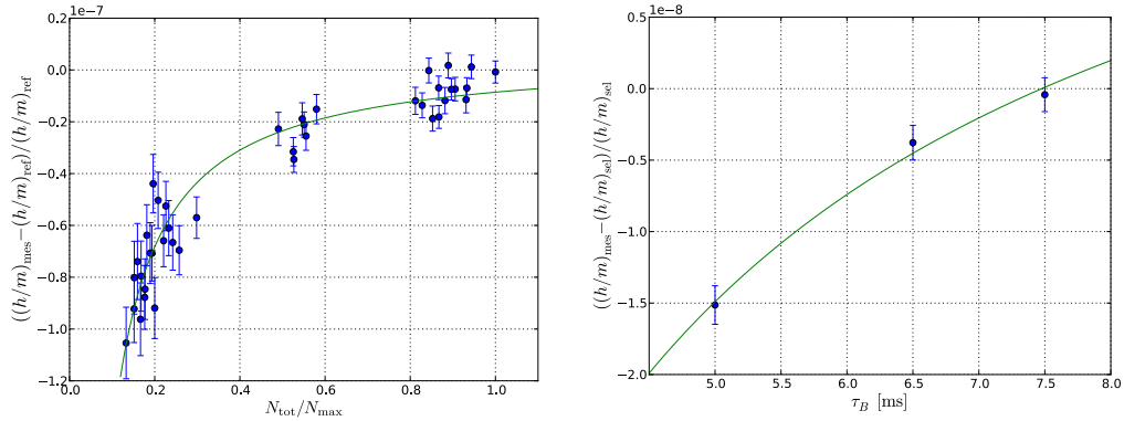
(a) Effet de l'intensité des faisceaux Bloch sur la valeur de h/m .
