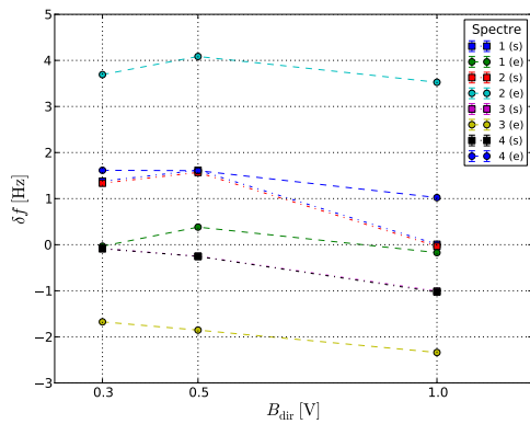
(a) Position du centre des franges \delta f pour les trois valeurs de champ magnétique directeur, valeurs simulées (s) et expérimentales (e).
