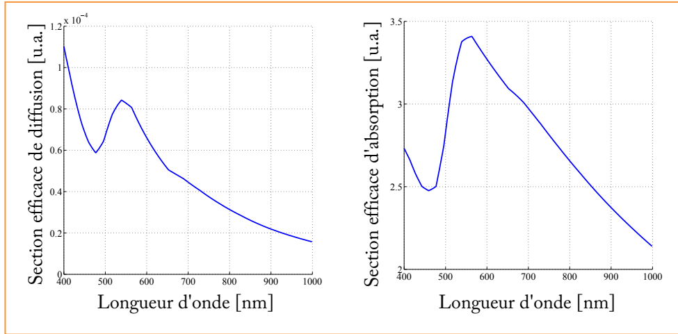
Figure 3.2 – Sections efficaces d'absorption et de diffusion calculées à l'aide de l'équation 3.3 pour une nanoparticule sphérique d'or de 5 nm de diamètre.
