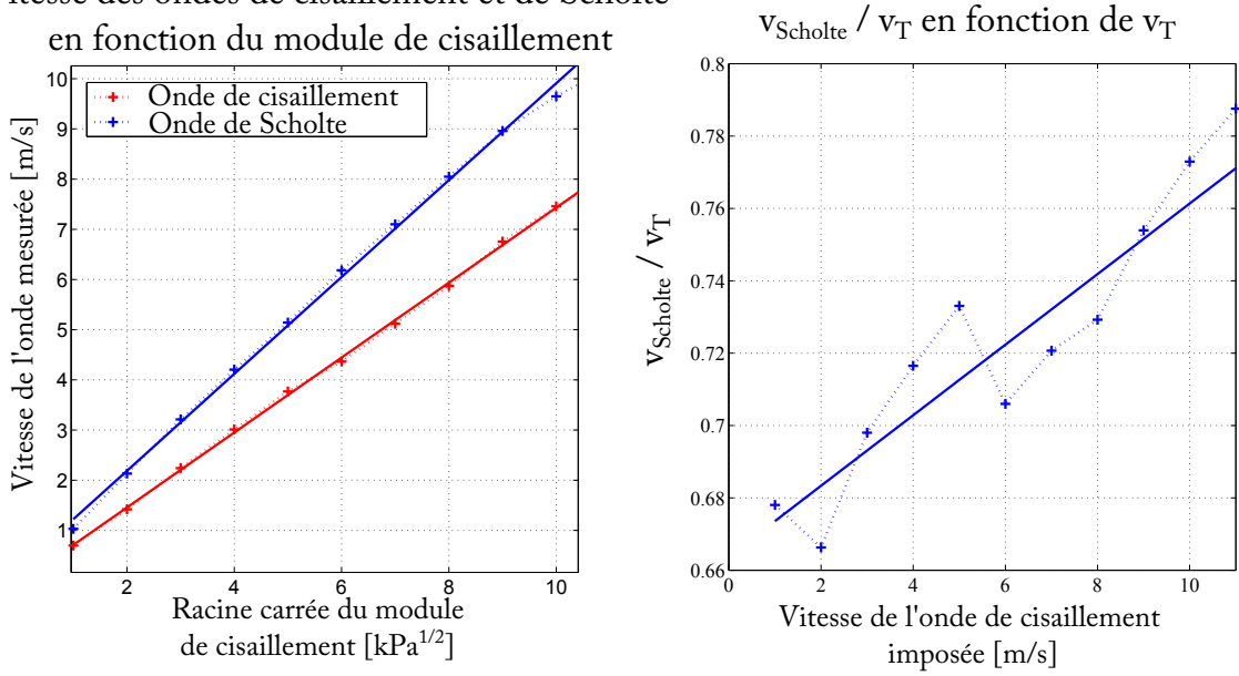
Figure 7.3 – Résultats de simulations pour des milieux isotropes, semi-infinis de rigidité différente. A gauche le graphique représente les vitesses de propagation des ondes de Scholte et des ondes volumiques de cisaillement en fonction de la racine carrée du module de cisaillement \sqrt{\mu} . A droite est représenté le quotient entre la vitesse de propagation des ondes de Scholte et des ondes volumiques de cisaillement en fonction de la racine carrée du module de cisaillement \sqrt{\mu} .
