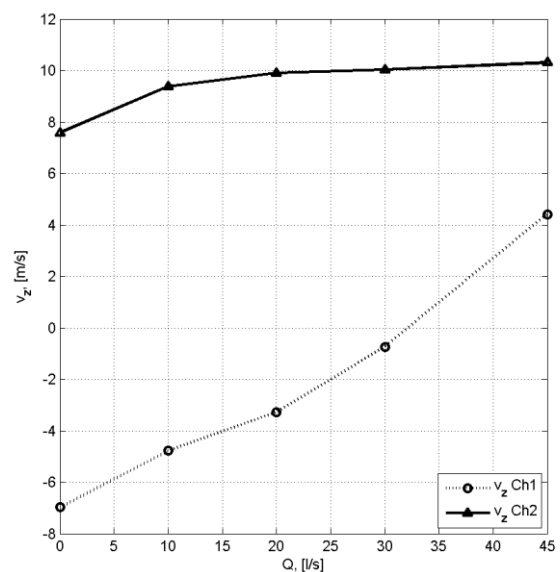
Fig. R 16. v_z [m/s] dans le milieu de la sous-canal en fonction du débit.
