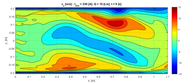
Fig. R 19. v_z [m/s]: Rm_S = 4.47 , t = 0 s.
