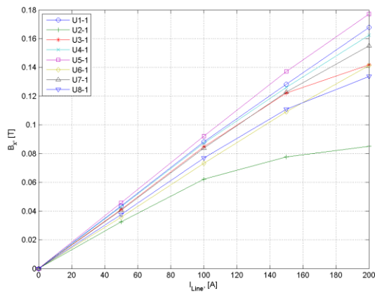
Fig. R 35. |B_x| en tant que fonction de I_{line} pour tous les échantillonneurs 1 st bobine.
