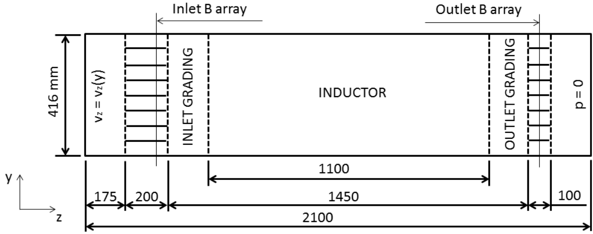
Fig. R 17. Géométrie et la configuration du modèle numérique sans sous-canaux.
