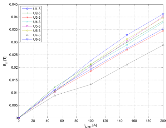
Fig. R 37. |B_x| en tant que fonction de I_{line} pour tous les échantillonneurs 3 rd bobine.
