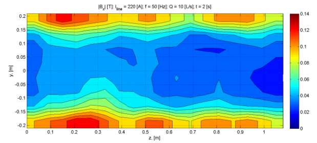
Fig. R 50. |B_x| [T]: Rm_S = 4.47 , t = 2 s.
