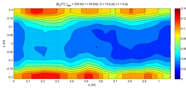
Fig. R 49. |B_x| [T]: Rm_S = 4.47 , t = 1.4 s.
