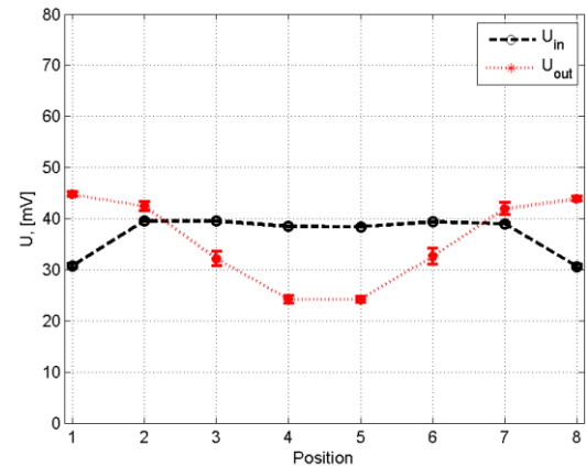
Fig. R 27. Différence de potentiel: Rm_s = 3.5 .
