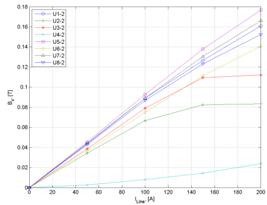
Fig. R 36. |B_x| en tant que fonction de I_{line} pour tous les échantillonneurs 2 nd bobine.
