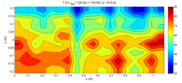
Fig. 250. T [C] , Rm_s = 3.43
