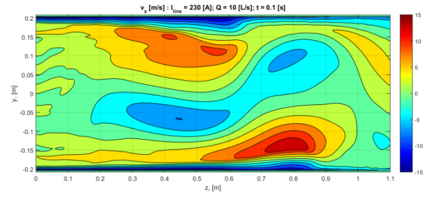
Fig. R 21. v_z [m/s]: Rm_S = 4.47 , t = 0.1 s.
