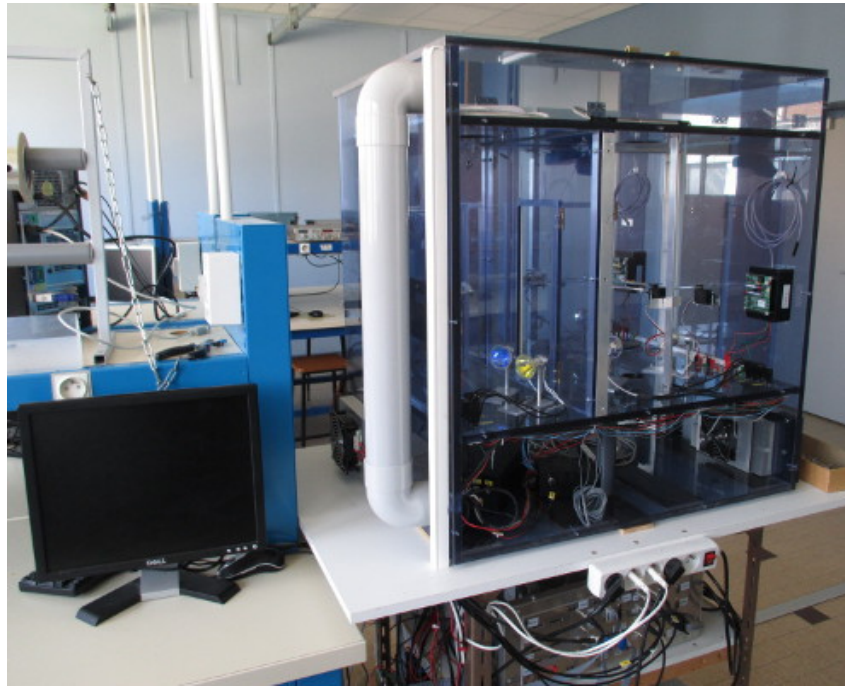
Figure 4 – Maquette d'un bâtiment intelligent de 4 pièces avec la solution UFAD.
