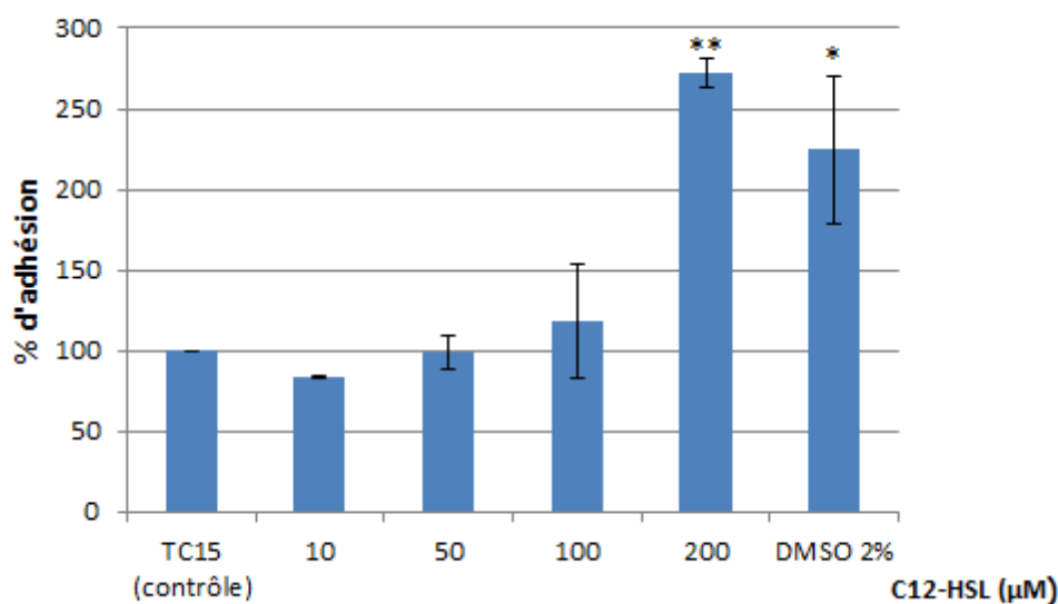
Figure 47 Effet de la C 12 -HSL exogène sur l'adhésion de TC15 en microplaque. Les résultats sont exprimés en % d'adhésion. Les essais marqués par des astérisques sont significativement différents par rapport au contrôle (culture de TC15 sans C 12 -HSL) (Tukey; **: p < 0,01; *: p < 0,05). L'expérience a été réalisée trois fois en triplicats.
