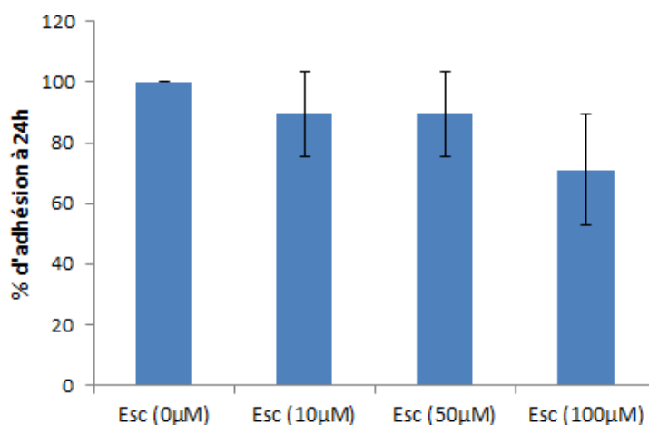
Figure 71 Effet de l'esculetine sur l'adhésion de TC14.
