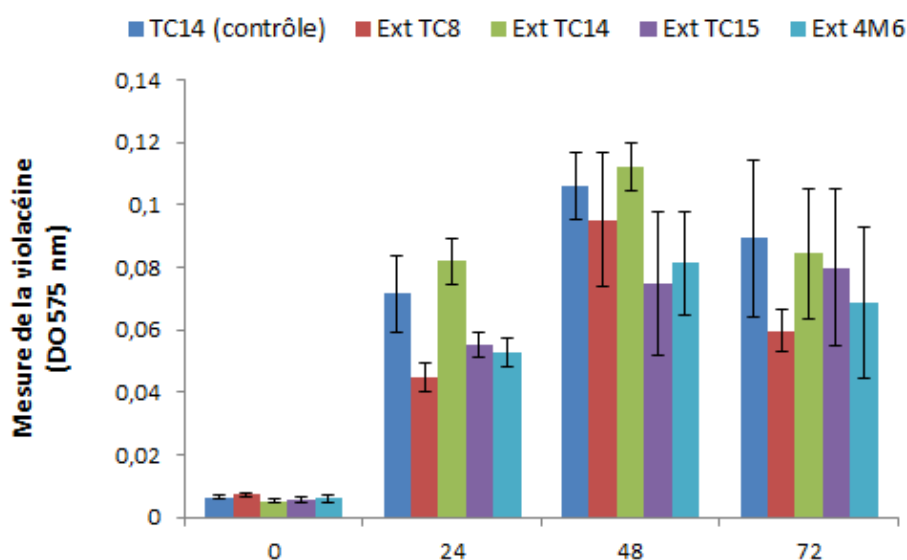
Figure 63 Effet des extraits de bactéries marines sur la production de violacéine par TC14. La violacéine a été mesurée à différents temps d'incubation (0,24, 48 et 72h) et les résultats ont été comparés au contrôle (culture de TC14 sans extraits). Chaque expérience a été réalisée trois fois en triplicat.
