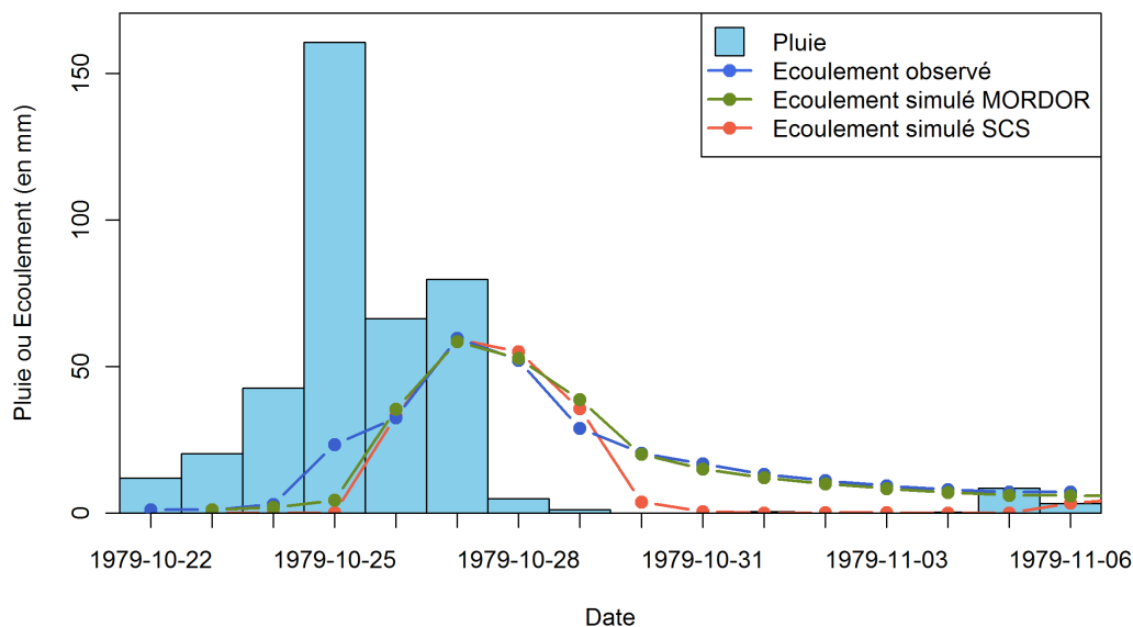
FIGURE V.4 – Un exemple d'événement simulé pour le bassin de l'Agout à Fraisse.
