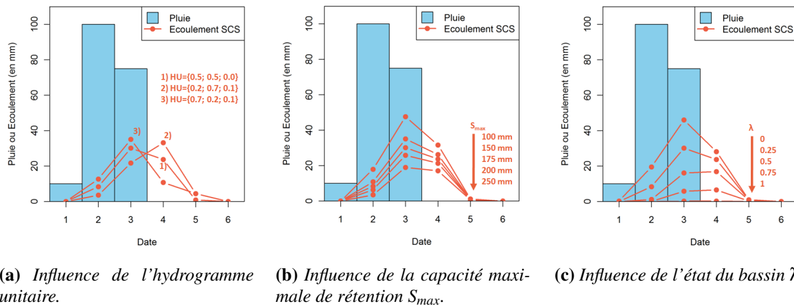
FIGURE V.5 – Influence des différents paramètres du modèle SCS sur la simulation d'un événement.
