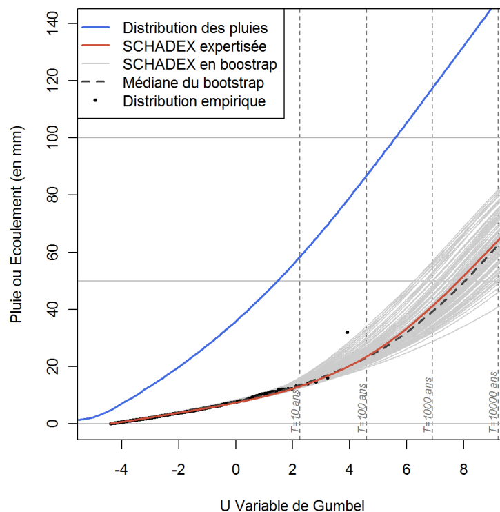
FIGURE V.24 – Les distributions de débits journaliers obtenues avec la méthode SCHADEX sur le bassin de la Creuse à Fresseline (1238 km 2 ).
