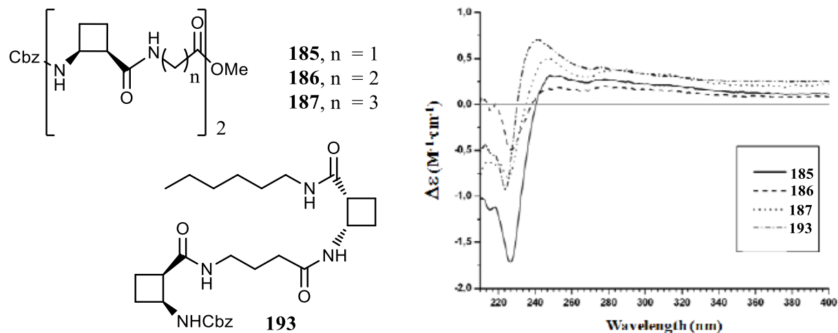
Figure 57 : \beta -peptides cyclobutaniques (gauche) ; spectre de CD à l'état solide (30 mM dans le KBr) des tétrapeptides 185 , 186 , 187 et 193 . 139
