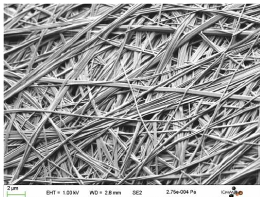
Figure 75 : L'image de MEB des fibrilles obtenues par le tripeptide 205 . 132
