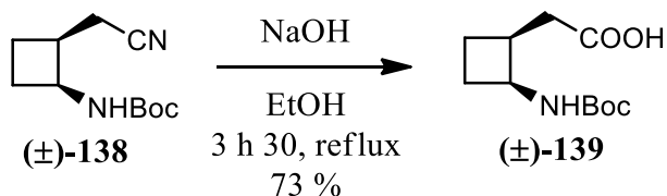
Schéma 54 : Hydrolyse basique et formation de l'acide N -Boc homologué.
