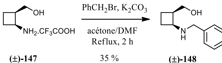
Schéma 56 : Protection de l'aminoalcool par le bromure de benzyle.
