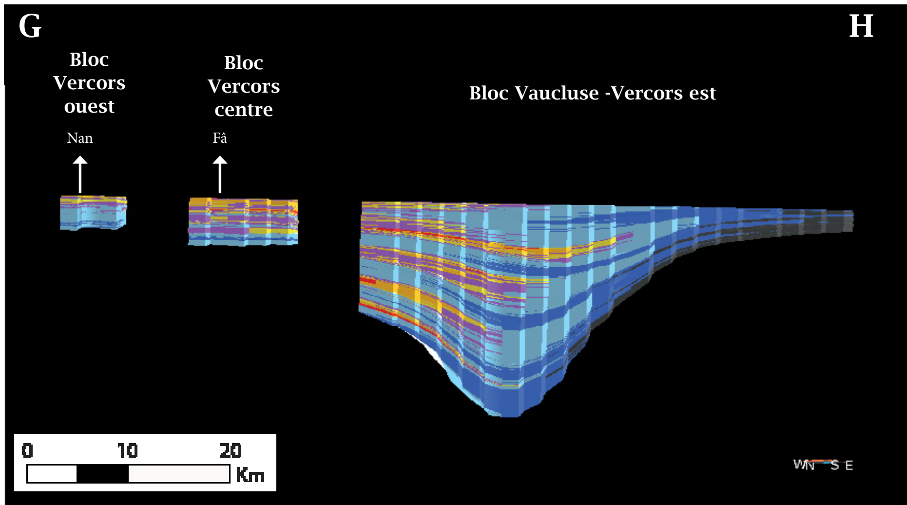
Figure 5-34 : Coupe est-ouest du modèle stratigraphique renseigné en environnements de dépôt à travers le bloc est du Vercors. L'exagération verticale est de facteur 15.
