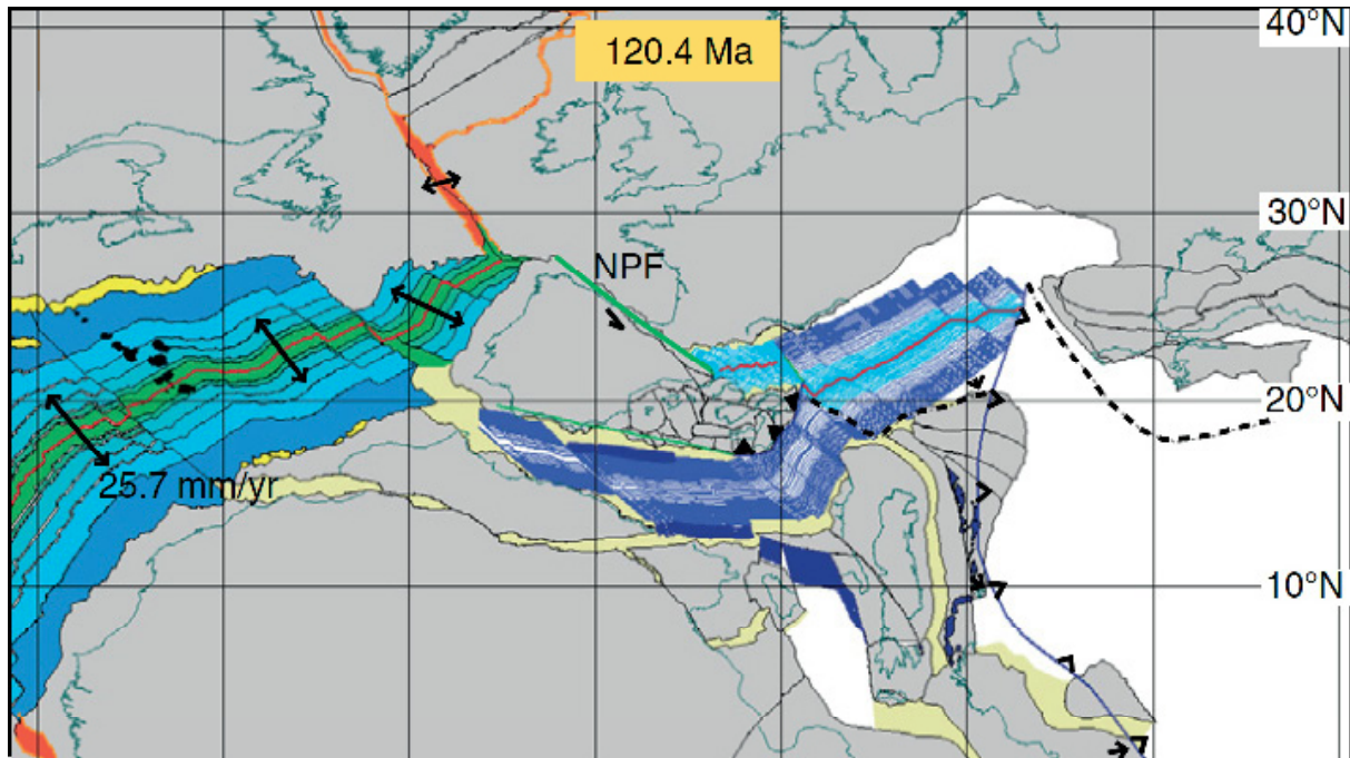
Figure 6-1 : Reconstruction paléogéographique au niveau de l'anomalie magnétique M0 (limite Barrémien-Aptien). NPF correspond à la faille Nord Pyrénéenne. (Schettino et al. , 2011)
