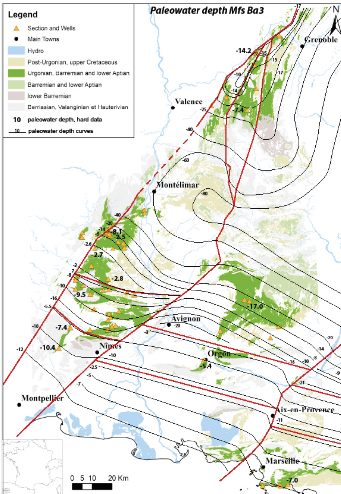
Annexe 79 : Carte de paléoprosfondeur d'eau au niveau la surface d'inondation maximum de la séquence
