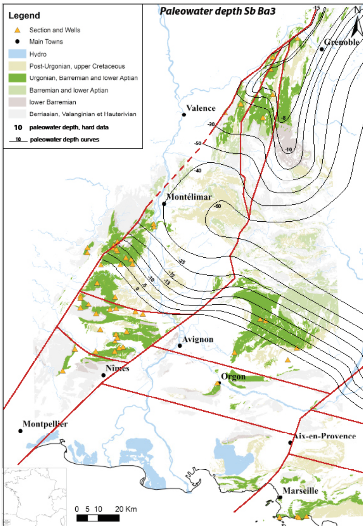
Annexe 77 : Carte de paléopronfondeur d'eau à la base de la séquence Ba3.
