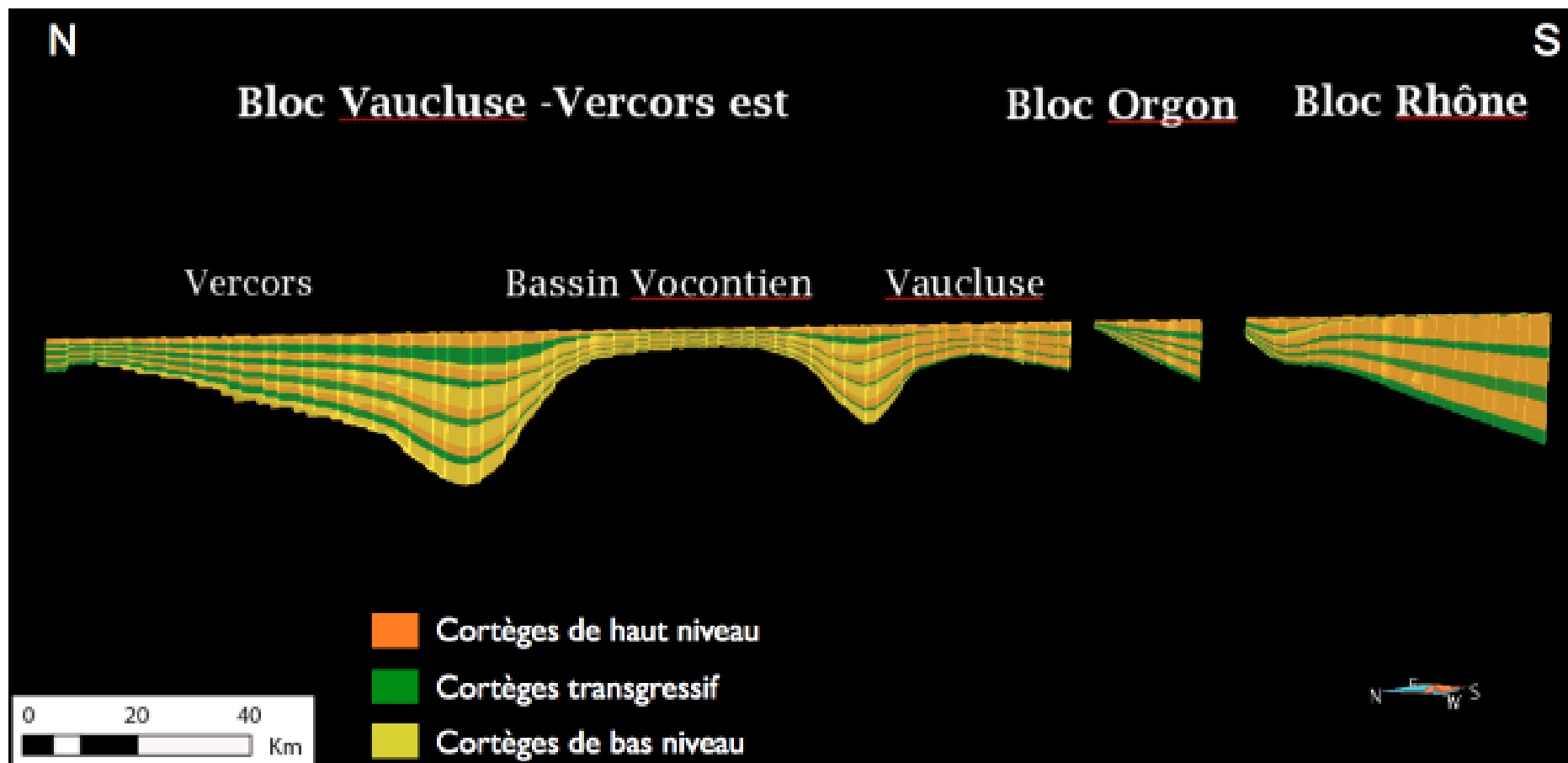
Figure 7-1 : Coupe nord sud à travers l'ensemble du modèle renseignés en cortège sédimentaires.
