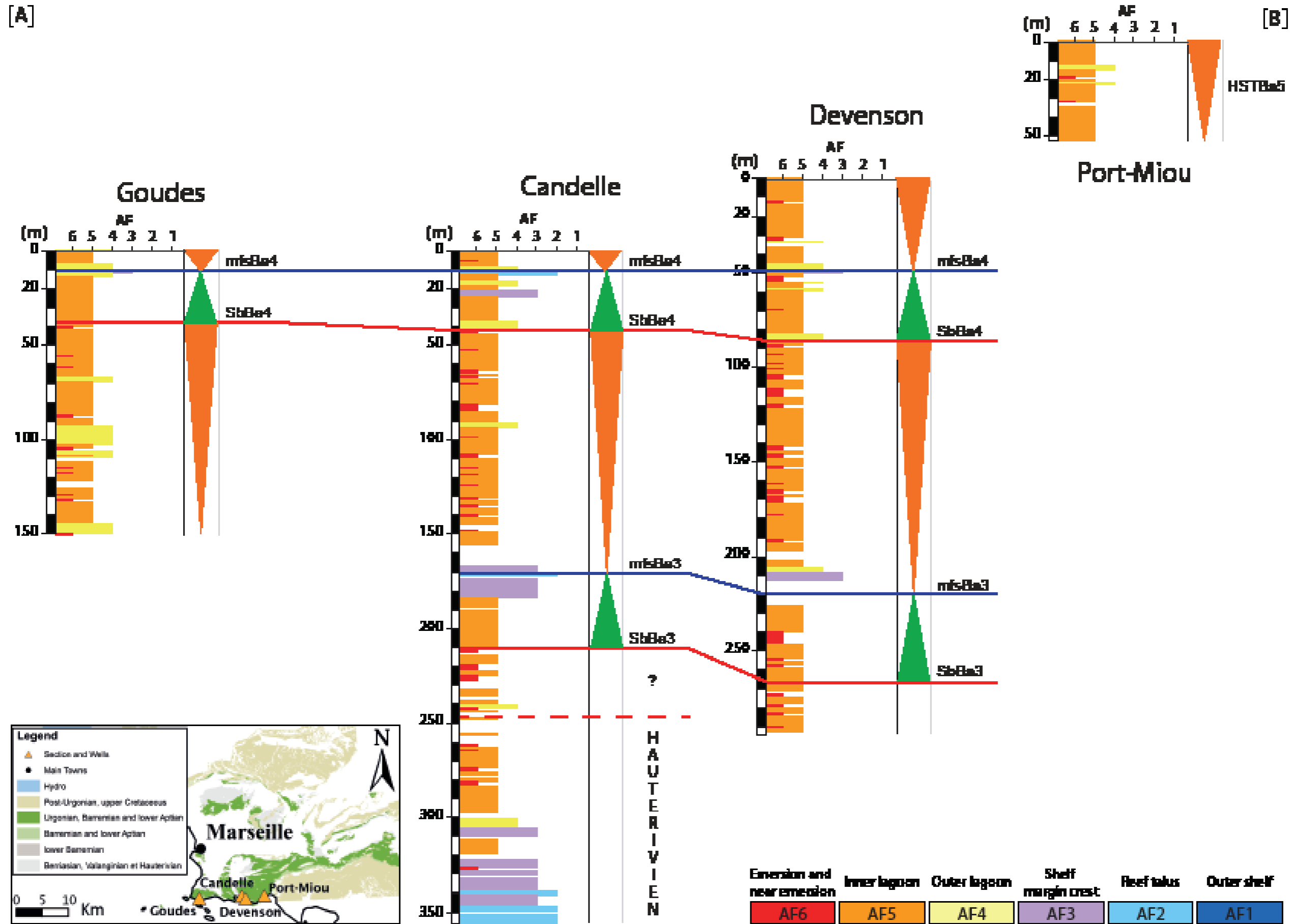
Figure 4-25 : Corrélation des quatre coupes du secteur de la Provence.
