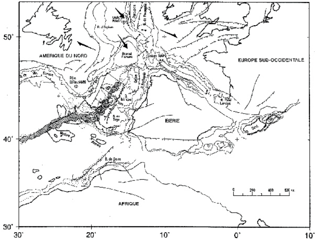
Figure 6-3 : Reconstitution paléogéographique au niveau de l'anomalie M0 d'après Olivet, 1996.
