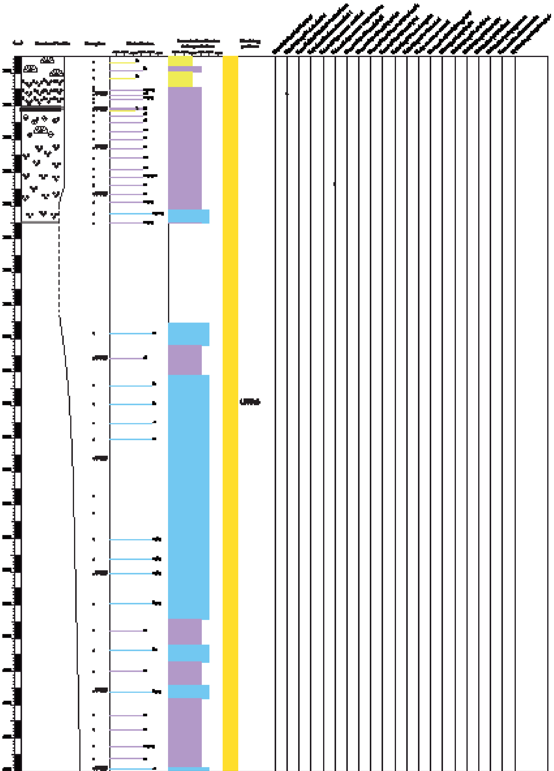
Annexe 35: Partie centrale du log stratigraphique de la coupe de Pont de Laval (Ardèche).
