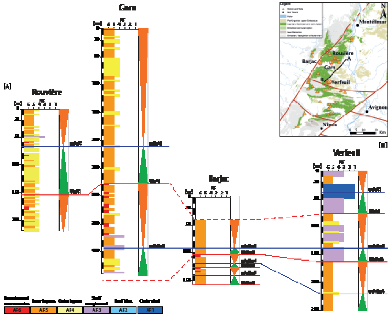
Figure 4-10 : Correlations des coupes du Nord du Gard et de l'Ardèche.
