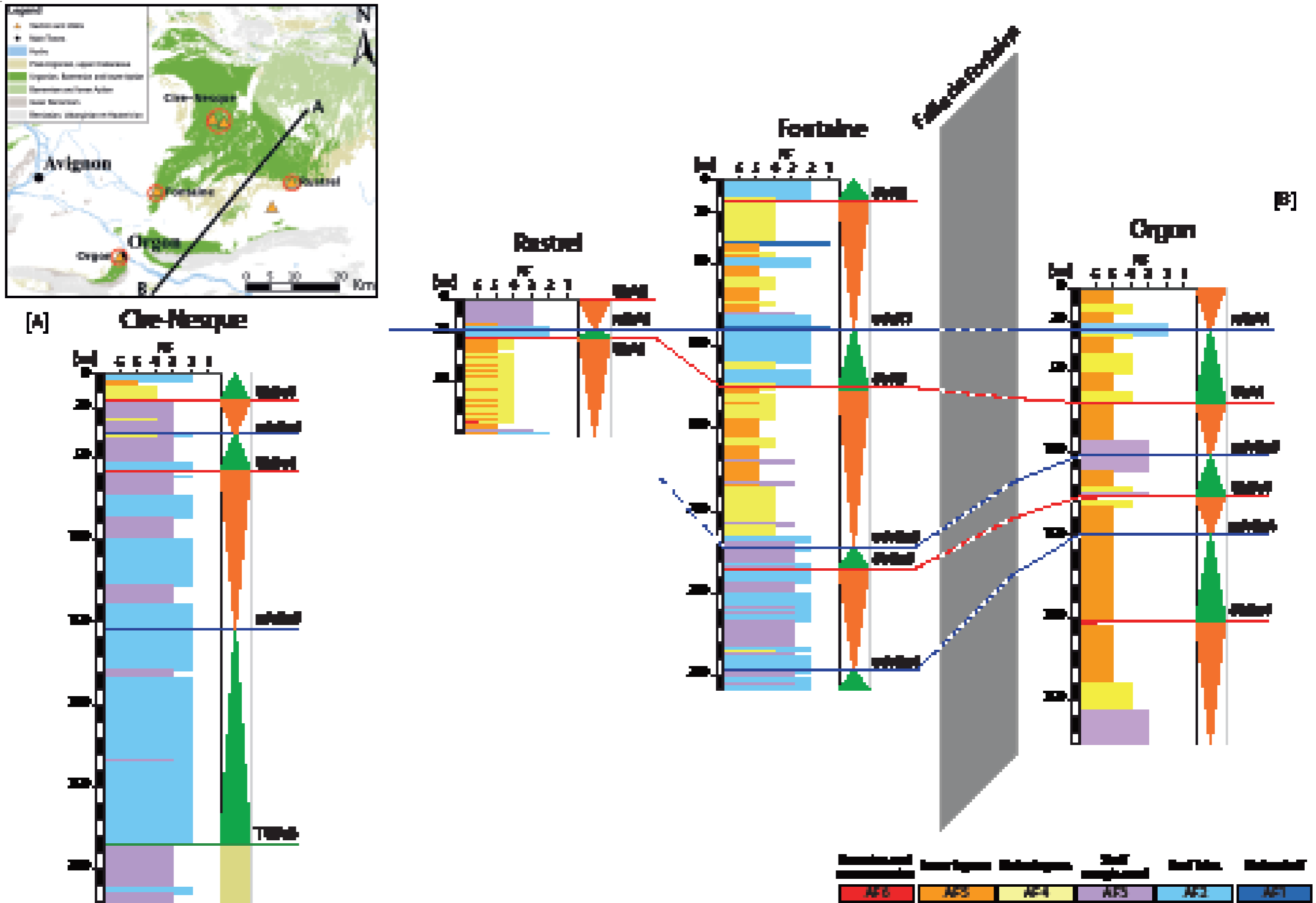
Figure 4-21 : Corrélations des coupes et puits du secteur du Vaucluse.
