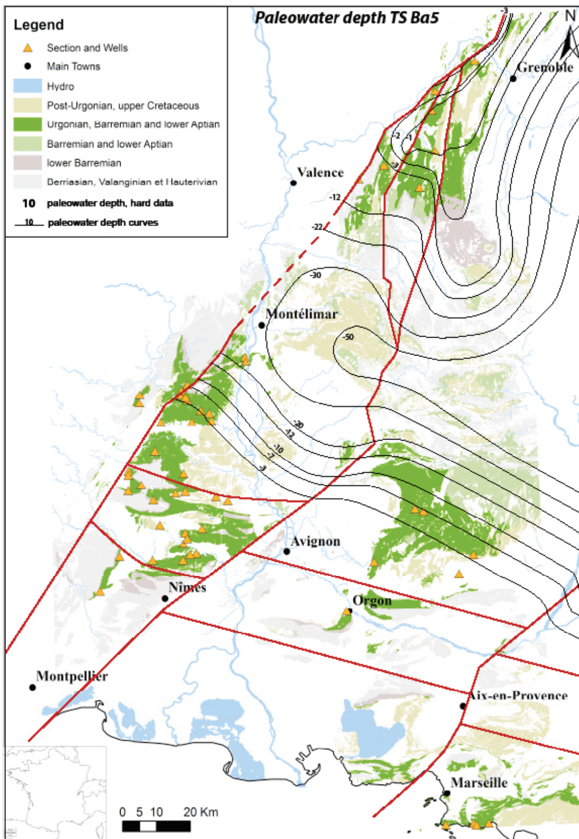
Annexe 84 : Carte de paléopropfondeur d'eau au niveau de la surface transgressive de la séquence Ba5.
