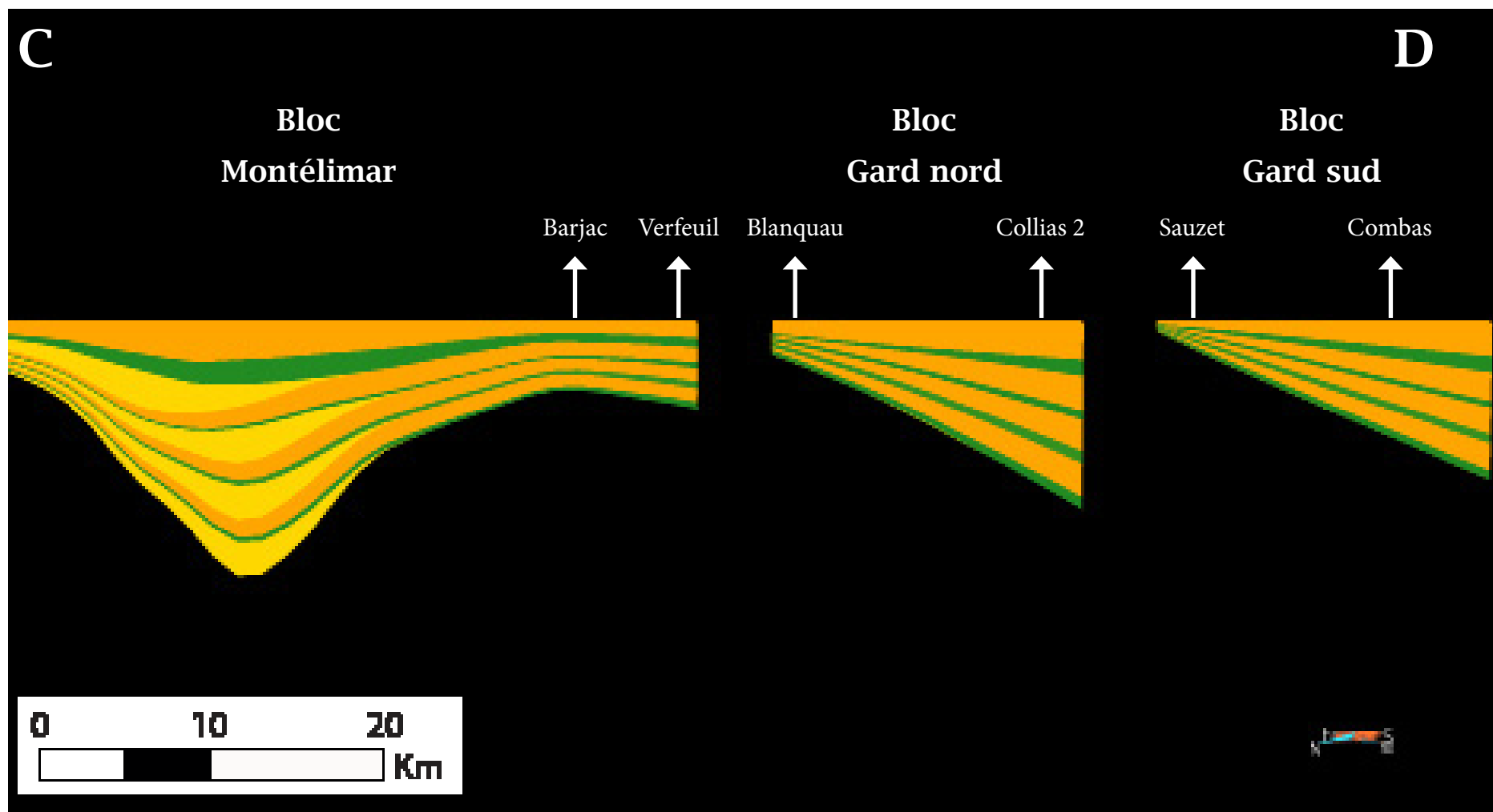
Figure 5-25 : Coupe nord nord-est à travers les blocs du Gard et le sud du bloc Montélimar. Les couches numériques colorées en jaune appartiennent aux cortèges de bas niveau, celles colorées en vert au cortèges transgressifs et celles colorées en orange aux cortèges de haut niveau. L'exagération verticale est de facteur 15.
