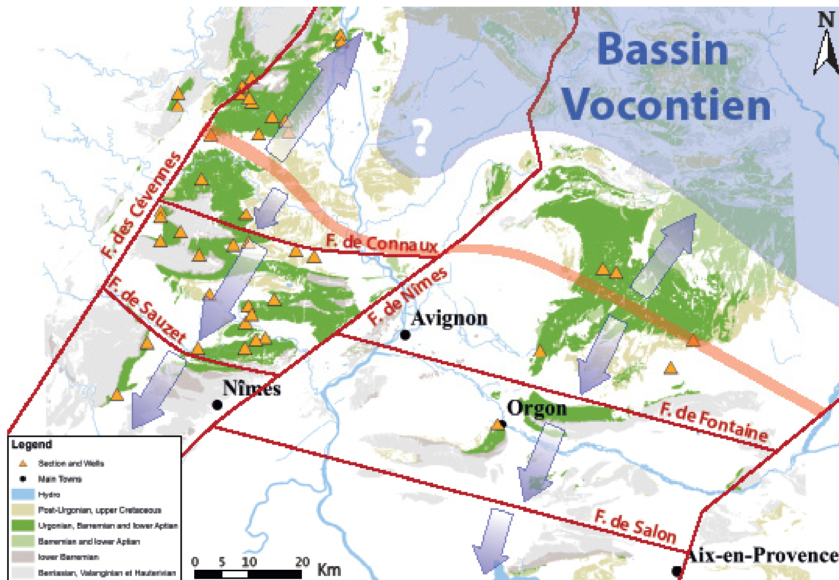
Figure 4-22 : Carte représentant l'organisation de l'Urgonien des secteurs du Gard, de l'Ardèche et du Vaucluse. Les traits rouges représentent les failles délimitant les blocs basculés, les flèches bleues illustrent la subsidence induite par le jeu des failles et les zones rouges représentent les zones de haut-fond.
