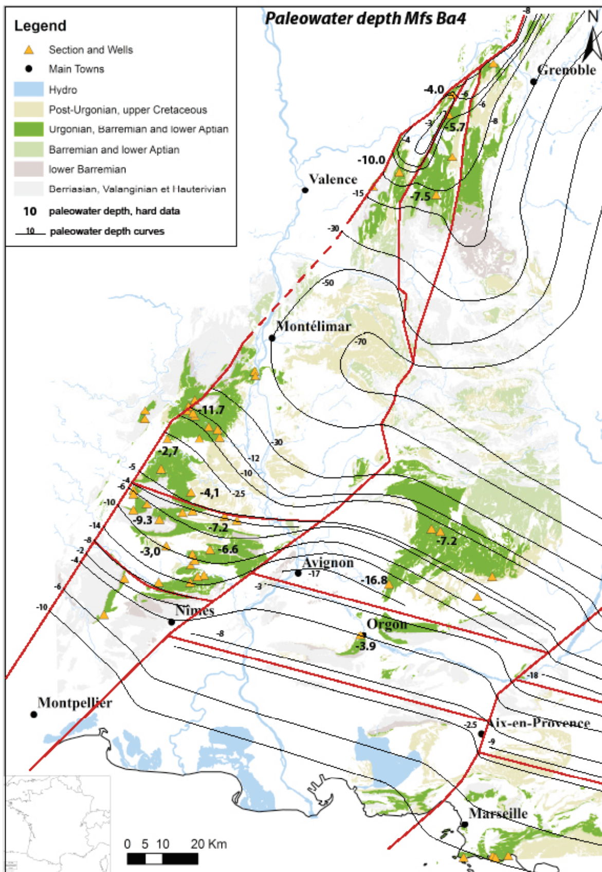
Annexe 82 : Carte de paléoprosfondeur d'eau au niveau de la surface d'inondation maximum de la séquence Ba4.
