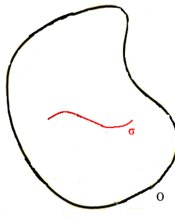
FIGURE 4.1 – Un domaine tridimensionnel \mathcal{O} avec une fracture unidimensionnelle \sigma .
