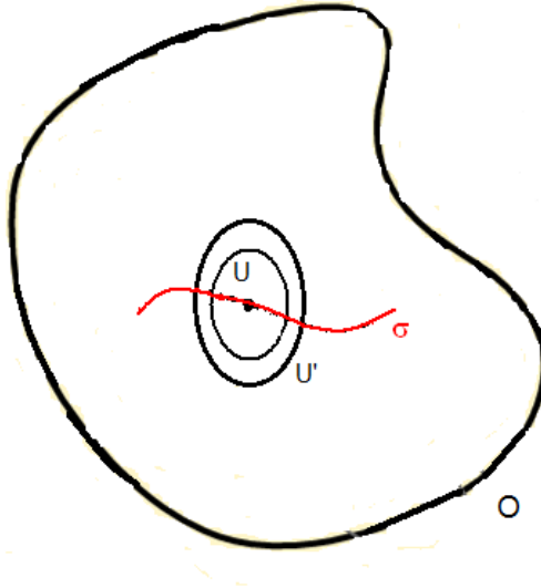
FIGURE 4.2 – Localisation à l'intérieur de \sigma .
