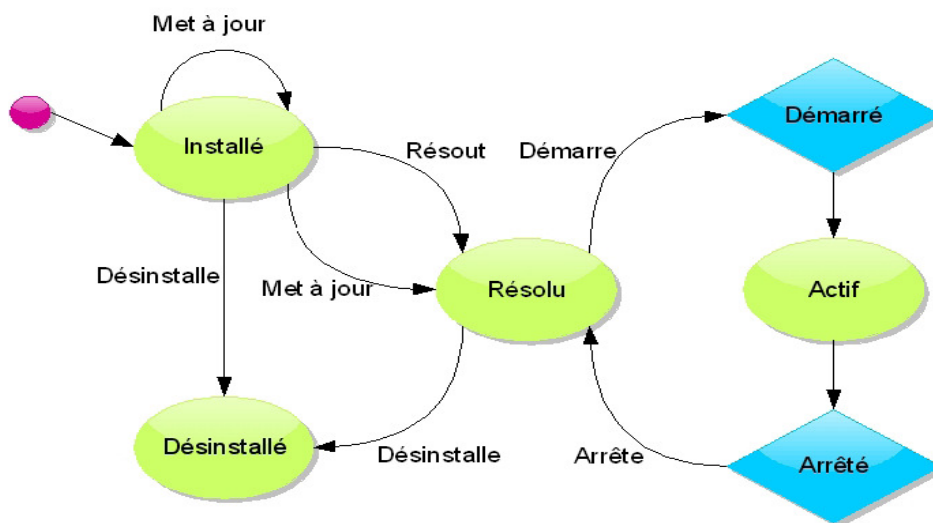
Figure 3.8 : Cycle de vie d'un bundle OSGi [99]
