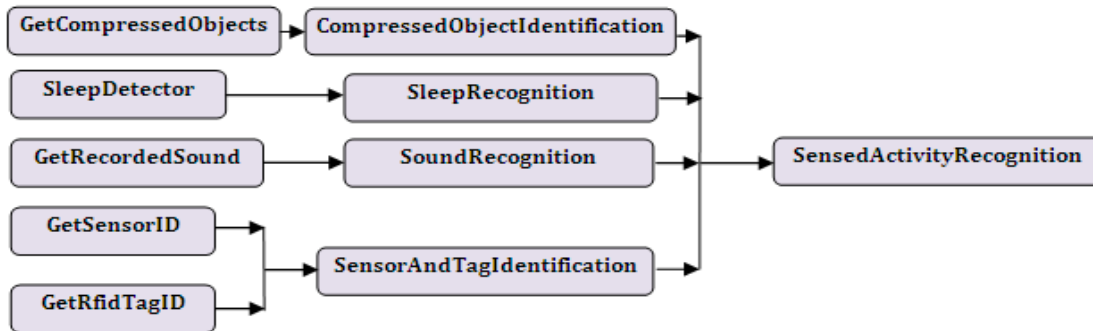
Figure 7.18 : Sous graphe SubGoSC du scénario « Reconnaissance d'activité ».
