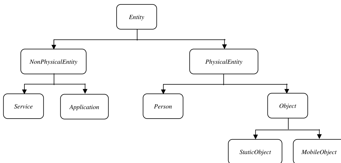
Figure 5.4 : Exemple d'une ontologie du concept « Entité »
