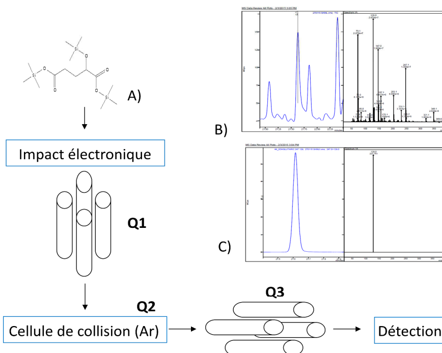
Figure 17 : Schéma explicatif de la spectrométrie de masse en tandem.
