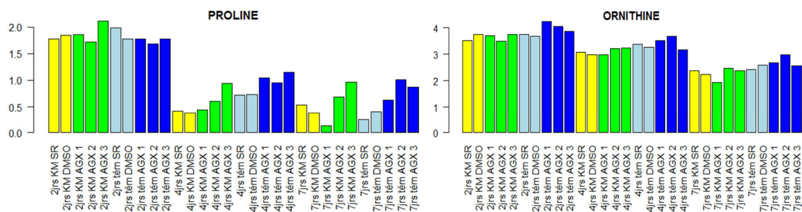
Figure 13 : Effets notoires de l'inhibiteur Agios sur la concentration de certains métabolites..
