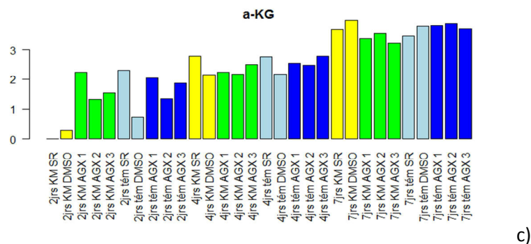
Figure 15 : Etude de l'action de l'inhibiteur sur le flux, par marquage isotopique d'intermédiaire à partir de la glutamine ^{13}\text{C}_5 .
