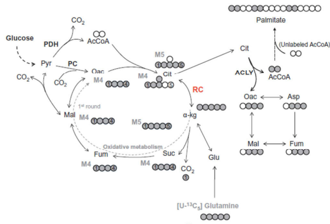
Figure 20 : Carte des composés marqués par la glutamine ^{13}C_5 avec leur nombre de carbones marqués. [Zhang et al. , 2014]
