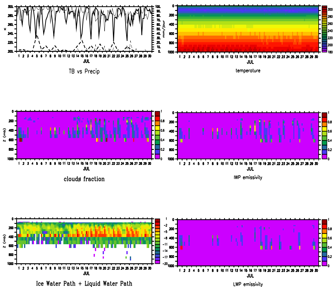
Figure 5.8 – Evolution temporelle de TB (K) de LMDZ (ligne continue fine) et MSG (ligne continue épaisse) et des précipitations (mm/jour) de GPCP (ligne en tireté épaisse) et du modèle LMDZ (ligne en tireté fine), profils de la fraction nuageuse en % (clouds fraction) et les profils d'eau liquide et de la glace (g/kg) représentés en \ln q (Ice Water Path + Liquid Water Path) (à gauche); ainsi que les profils d'émissivités montantes en présence d'eau et de glace et leur température physique (K) sur Niamey pour le mois de Juillet 2006 (à droite).
