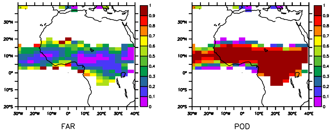
Figure 6.9 – Carte moyenne de FAR et de POD des précipitations GPCP et du modèle LMDZ sur la phase active de la mousson 2006
