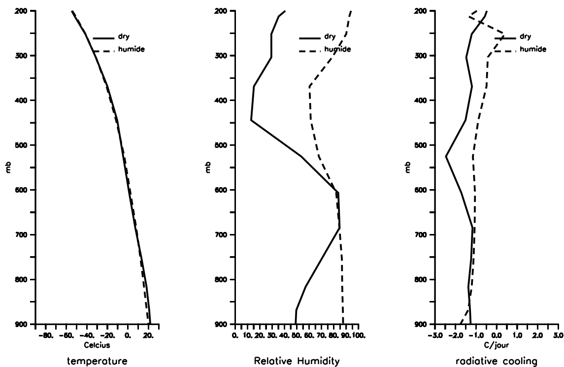
Figure 6.19 – Profil de température ( ^{\circ}C ), de RH (%) ainsi que des tendances radiatives ( ^{\circ}C/jour ) du modèle LMDZ sur l'évènement de "dry intrusion" du 23-sep-2006 à 22 :00 et la période humide du [13 – sep – 2006 : 16 – sep – 2006] au niveau de Dakar.
