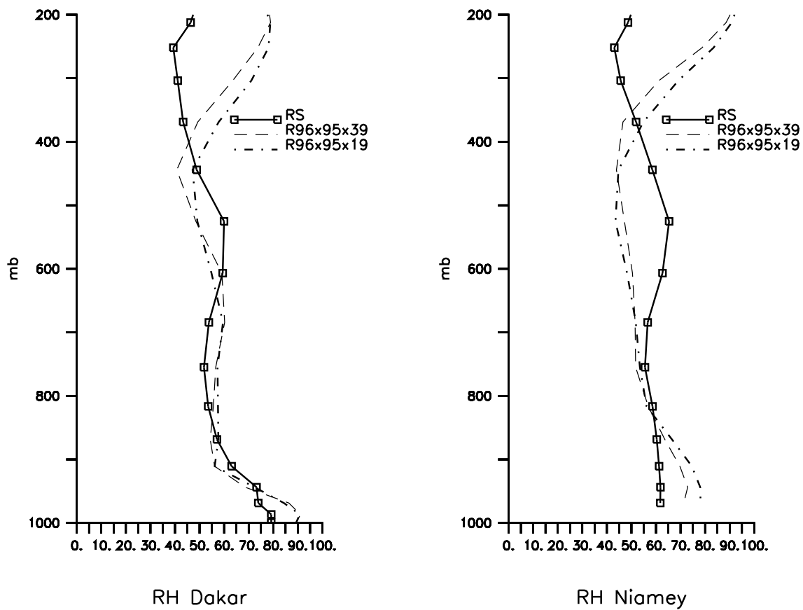
Figure 5.5 – Profils moyens de RH (%) sur la saison de mousson 2006 des radiosondages de AMMA (trait plein et carré) et des deux versions du modèle LMDZ, "R96x95x39" (tirets) et "R96x95x19" (points et tirets) sur les stations de Dakar et Niamey. Les profils sont interpolés sur la grille de résolution à 39 niveaux verticaux.
