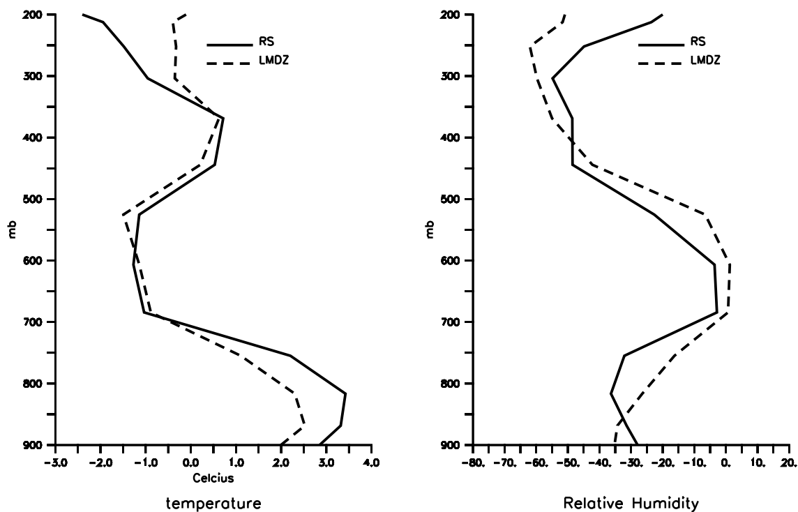
Figure 6.20 – Différence de températures ( ^{\circ}C ), de RH (%) du modèle LMDZ et des observations de radiosondages sur l'évènement de "dry intrusion" du 23-sep-2006 à 22 :00 par rapport à la période humide [13 – sep – 2006 : 16 – sep – 2006] au niveau de Dakar.
