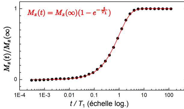
FIGURE 2.3 – Courbe de relaxation T_1 de l'aimantation nucléaire \mathcal{M}_z(t) sur le proton ^1\text{H} (spin I = 1/2 ) après saturation par un pulse " \pi/2 " ( \mathcal{M}_z(0) \approx 0 ) : données expérimentales (cercles pleins) et ajustement par la relaxation théorique, dans ce cas une exponentielle simple (tracé rouge).
