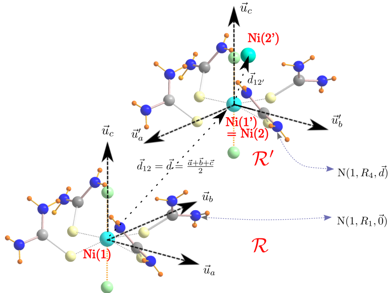
FIGURE D.1 – Opération de passage du repère \mathcal{R} au repère \mathcal{R}' , défini ici par la rotation R_4 et la translation t_{\vec{d}} . On a mis en évidence les azotes \text{N}(1, R_1, \vec{0}) et \text{N}(1, R_4, \vec{d}) . On a dans ce cas particulier \text{O}' = \text{Ni}(2) = \text{Ni}(1') .
