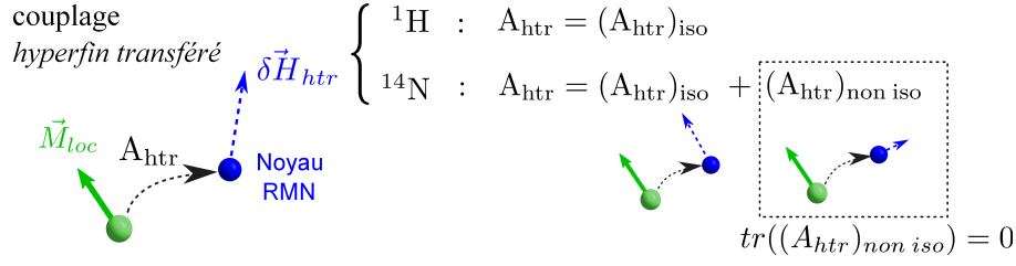
FIGURE 3.2 – Description du mécanisme de couplage hyperfin transféré. La polarisation ( \vec{M}_{\text{loc}} ) se transfère sur les orbitales de valence du site étudié, induisant un champ local RMN \delta\vec{H}_{\text{htr}} . Les propriétés du tenseur A_{\text{htr}} diffèrent entre les protons (couplage isotrope) et l’azote (présence d’une composante anisotrope).
