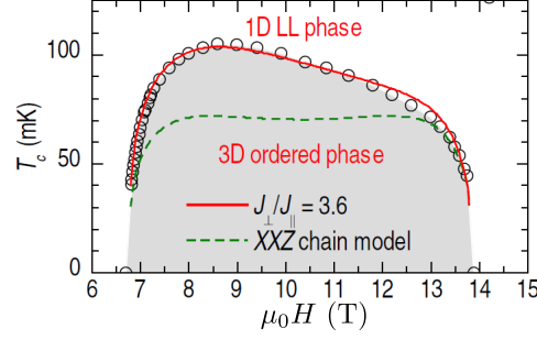
FIGURE 1.6 – Diagramme de phase H - T de BPCB montrant (cercles) la dépendance de la température T_c(H) de transition vers la phase d'ordre AF ("3D ordered phase"), déterminée par RMN. La courbe en tirets verts correspond à la prédiction des paramètres TLL u et K issue du modèle de chaîne XXZ ("XXZ chain model", décrit en section 1.4) ; la courbe en trait rouge continu correspond à la prédiction utilisant le Hamiltonien complet de BPCB avec J_{\perp}/J_{\parallel} = 3.6 [13]. Cette dernière ajuste bien les points expérimentaux.
