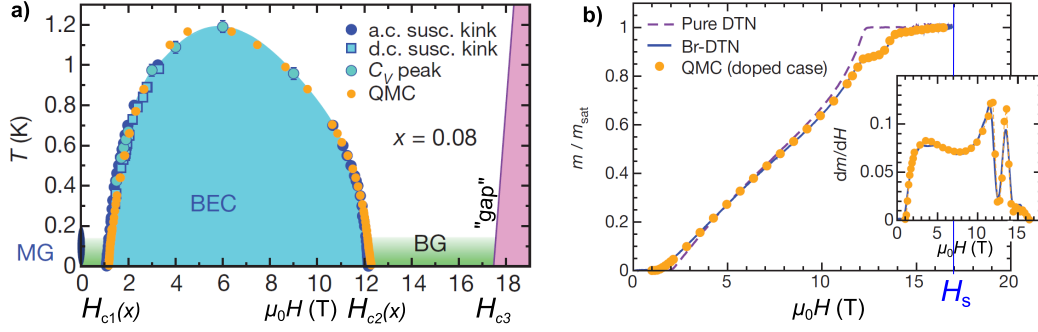
FIGURE 1.11 – Données expérimentales et description du diagramme de phase de \text{Ni}(\text{Cl}_{1-x}\text{Br}_x)_2\cdot 4\text{SC}(\text{NH}_2)_2 (obtenu à partir de DTN, dans lequel on a introduit du désordre par substitution d'une fraction x des chlores par des broles), pour le composé dopé à 8% ( x=0.08 ), adapté d'après [51] : a) Diagramme de phase du composé. La courbe T_c(H) de transition vers la phase BEC inhomogène (BEC) est déterminée par plusieurs techniques expérimentales et simulée par méthode numérique QMC ("Quantum Monte Carlo") avec les paramètres J'_c = 2.35J_c et D' = D/2 . Les champs critiques sont abaissés par rapport au composé DTN pur : H_{c1} = 1.07 T et H_{c2} = 12.15 T. Les régions dans lesquelles on s'attend à observer la phase verre de Bose (BG) se trouvent de part et d'autre de la phase BEC ( H < H_{c1} et H > H_{c2} ), à basse température ( T \lesssim 200 mK). La limite à haut champ de la phase verre de Bose est donnée par l'"ouverture du gap" proposée à H_{c3} = 17.5 T, correspondant approximativement au champ H_s de saturation de l'aimantation b) Comparatif des courbes d'aimantation/susceptibilité à basse température dans DTN pur ( T = 16 mK) et dopé ( T = 19 mK), et simulation QMC de l'aimantation dans le composé dopé (avec les mêmes paramètres qu'en a)). L'aimantation sature à un champ H_s \sim 17 T.
