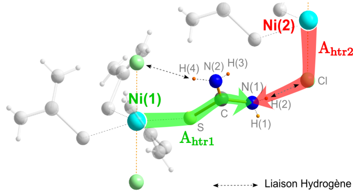
FIGURE 3.3 – Hypothèses de chemins de couplage hyperfin transféré dans la maille élémentaire (illustration pour le site N(1)). Le tenseur A_{\text{htr1}} représente le transfert de polarisation depuis le site Ni(1) à travers le fragment thiourée, tandis que le tenseur A_{\text{htr2}} représente un transfert venant du site Ni(2) via la liaison hydrogène impliquant H(2).
