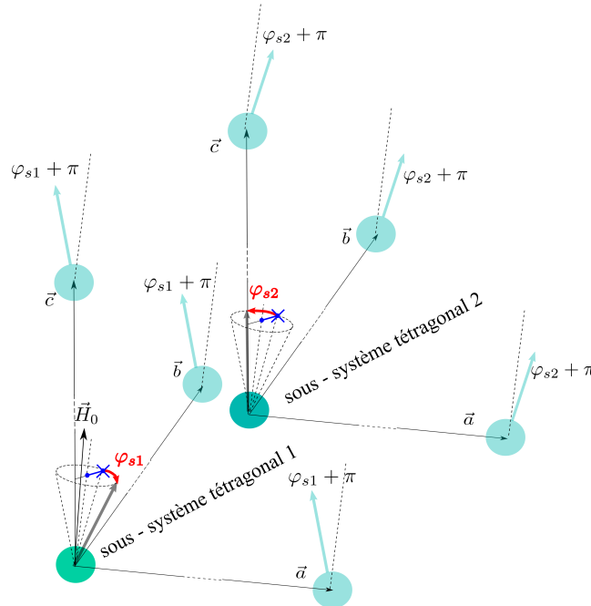
FIGURE A.4 – Description de la phase AF (ici le champ est légèrement désaligné de l'axe \vec{c} ) à l'aide des variables \varphi_{s1}, \varphi_{s2} qui définissent les orientations des composantes antiferromagnétiques.
