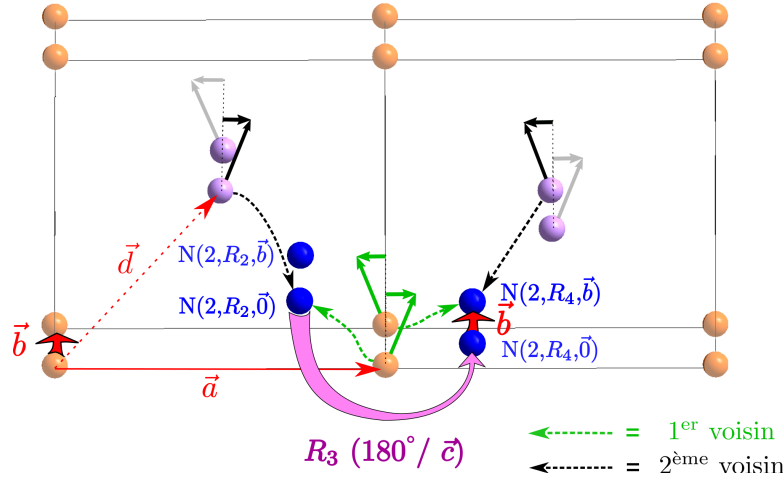
FIGURE 4.6 – Position relative d'un site N(i, R_{k+2}, \vec{v} + \vec{b}) par rapport à un site N(i, R_k, \vec{v}) reliés par l'opération : rotation R_3 (rotation de 180^\circ autour de \vec{c} ) + translation du vecteur \vec{b} . On peut montrer que ces sites subissent le même déplacement lié à la composante AF. Le raisonnement est valable en remplaçant \vec{b} par \vec{a} ou \vec{c} , et pour les sites de proton également (voir texte).
