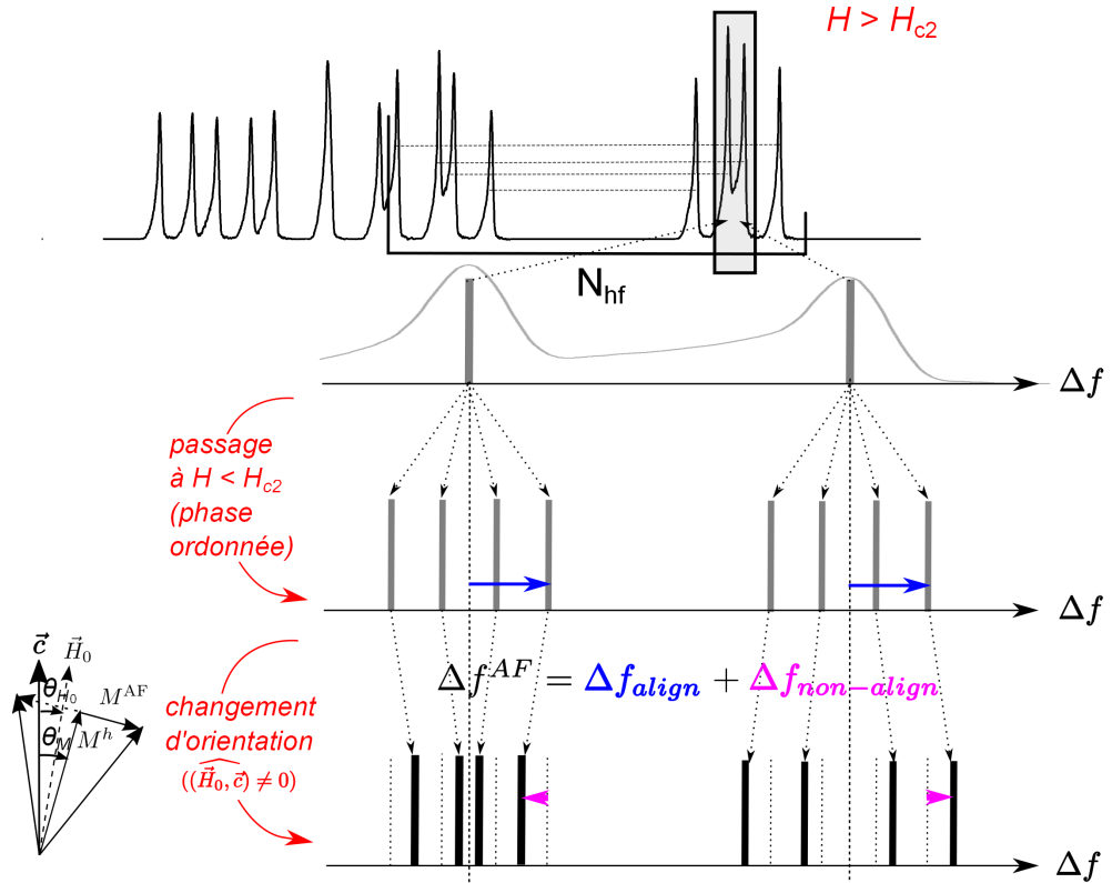
FIGURE E.1 — Prédiction d'une perturbation de la similitude des séparations AF de l'azote décrite en section 4.3, pour le site haute fréquence ( N_{hf} ), dans l'hypothèse d'une forte inclinaison du champ par rapport à l'axe \vec{c} .
