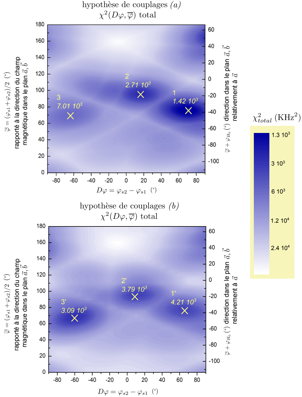
FIGURE 4.9 – Résultat des ajustements des séparations AF de l'azote dans la phase ordonnée, pour chaque hypothèse relative aux couplages hyperfins. Les graphes 2D représentent \chi^2_{total}(D\varphi, \bar{\varphi}) , obtenu en minimisant \chi^2 (en fonction des paramètres restants) pour chaque valeur des angles D\varphi, \bar{\varphi} , fixant les orientations des composantes AF sur chaque sous-système tétragonal. Les croix marquent les différents minima de \chi^2_{total} (valeurs écrites en italique). Les minima 1,2 et 1',2',3' vérifient \chi^2_{total} < 4.2 \cdot 10^3 KHz 2 .
