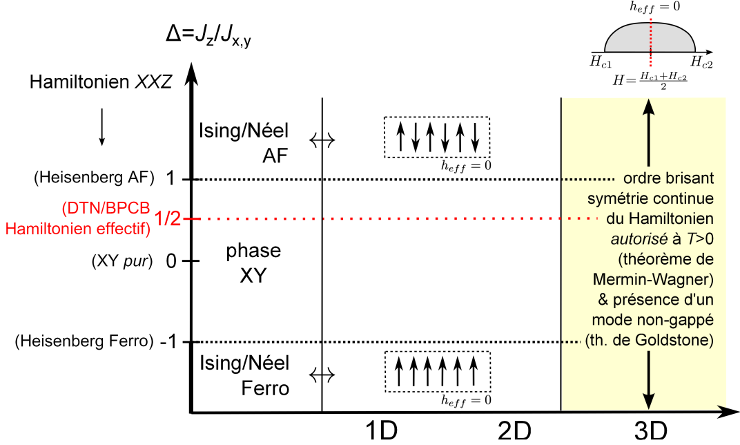
FIGURE 1.9 – "Diagramme de phase" du Hamiltonien XXZ tel que défini dans l'équation (1.7) en fonction de la dimensionalité du système et de la valeur du paramètre \Delta , en champ effectif nul, h_{eff} = 0 (ce qui correspond pour DTN et BPCB à un champ réel H situé entre la prédiction des deux champs critiques, voir figure en haut à droite), en supposant J_{x,y} > 0 (noté J dans le texte). Le Hamiltonien de DTN et BPCB a été rapporté au Hamiltonien XXZ pour \Delta = 1/2 . Pour le cas 1D et \Delta > 1 (Ising/Néel AF) nous avons représenté l'ordre présent à h_{eff} = 0 . Pour les cas 2D/3D, nous supposons que le couplage entre les chaînes est non-frustré. Le cas \Delta < 0 peut-être identifié à un Hamiltonien de spins 1/2 de type ferromagnétique après une transformation sur les opérateurs de spin (du type S_i^{x,y} \leftarrow (-1)^i S_i^{x,y} ) de sorte que dans ce cas les observables du système (comme les moments magnétiques locaux) ne peuvent pas être extrait directement. Le théorème de Mermin-Wagner exclut dans les cas 1D et 2D tout ordre à longue distance à T > 0 brisant la symétrie continue du Hamiltonien : symétrie axiale d'axe z (ou symétrie rotationnelle complète dans les cas particuliers \Delta = \pm 1 ). Un tel ordre est donc possible seulement dans le cas 3D, le théorème de Goldstone prédit alors la présence d'un mode à énergie nulle (ou non-gappé).
