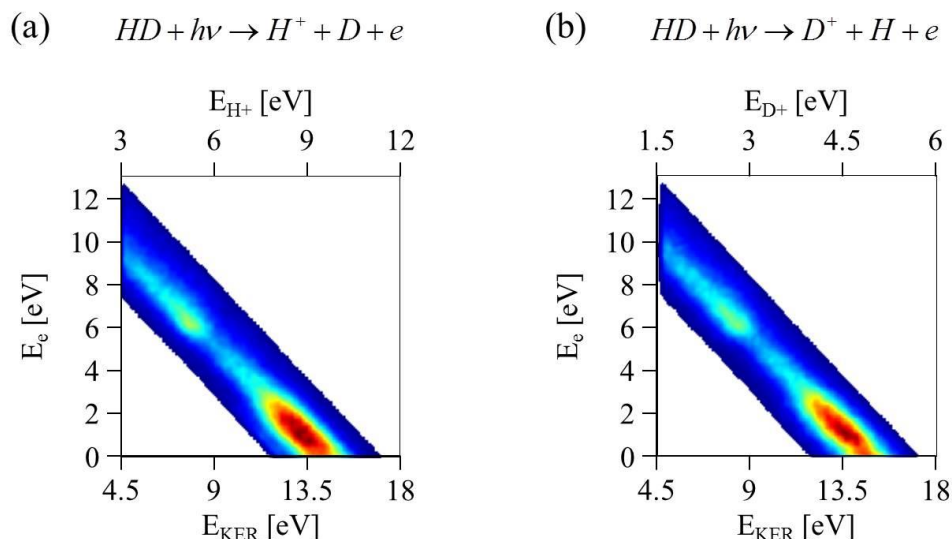
Figure VI-15 : KECDs des événements coïncidents ( H^+ , e ) (a) et ( D^+ , e ) (b) issus de la PID de la molécule HD induite à h\nu = 32.5 eV, pour une sélection en énergie des KERs telle que KER > 4.5 eV. L'énergie correspondante E_{H^+/D^+} des ions fragments est également reportée en abscisse au sommet du graphe.
