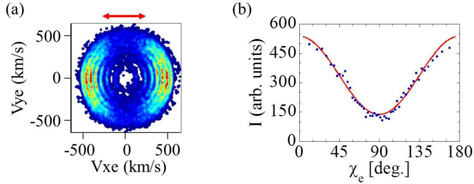
Figure III-4 : Diagramme bidimensionnel ( V_{xe}, V_{ye} ) représentant la distribution de vitesse des photoélectrons émis par la PI de O_2 vers l'état B^2\Sigma_g^- , induite par une lumière polarisée linéairement ( h\nu = 21.15 eV). L'axe de la polarisation est représenté par la flèche rouge (a). Distribution en angle polaire correspondante, où l'angle \chi_e repère la direction du vecteur vitesse du photoélectron par rapport à l'axe de polarisation de la lumière (b).
