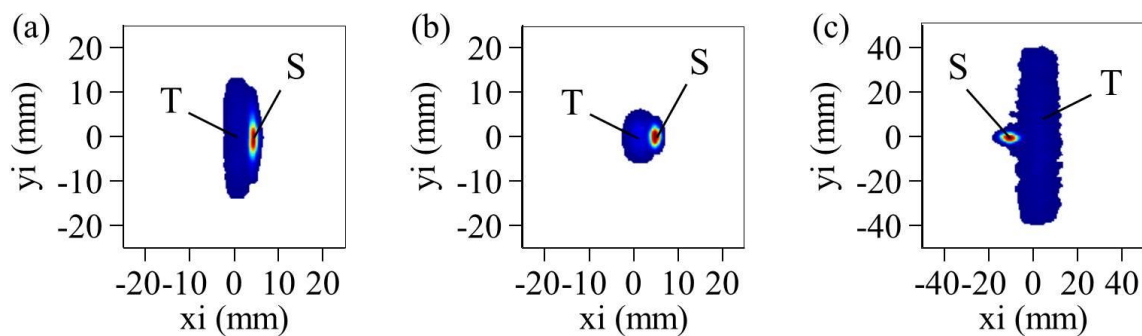
Figure I-8 : Diagrammes bidimensionnels ( x_i, y_i ) représentant les coordonnées d'impact sur le détecteur des ions \text{NO}^+ issus de la photoionisation non dissociative (PIND) de la molécule \text{NO} induite : par le rayonnement synchrotron à h\nu = 23.65 eV dans CV-40 avec E_{ext} = 60 V/cm sans focalisation (a) et E_{ext} = 30 V/cm avec focalisation (b), et par un rayonnement harmonique dans CV^B-80 avec E_{ext} = 8 V/cm sans focalisation et B = 8 G (c). Les contributions supersonique et thermique sont respectivement notées « S » et « T ».
