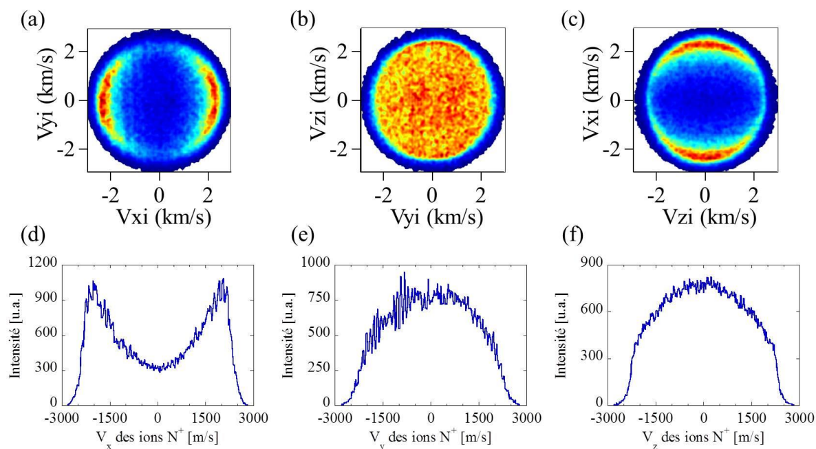
Figure II-5 : Diagrammes bidimensionnels (V_{xi}, V_{yi}) , (V_{yi}, V_{zi}) et (V_{zi}, V_{xi}) des ions N^+ produits par la PID de NO à h\nu = 23.65 eV (a-c). La projection de ces diagrammes, sur les axes des abscisses et des ordonnées, fournit la distribution de chaque composante V_{xi} , V_{yi} et V_{zi} (d-f).
