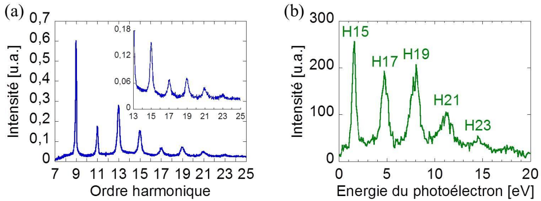
Figure V-22 : Spectre d'harmoniques d'ordre élevé générées dans des molécules de SF 6 par des impulsions IR polarisées elliptiquement, \varepsilon_{IR} = +0.2 (a). Spectre d'énergie cinétique des photoélectrons issus de la PID de NO correspondant (b).
