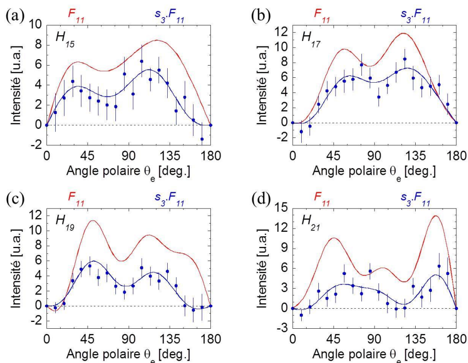
Figure V-24 : Produits s_3F_{11} (en bleu) et fonctions F_{11} de référence (en rouge) pour les harmoniques H15 (a), H17 (b), H19 (c) et H21 (d), générées dans des molécules de SF_6 par des impulsions IR polarisées elliptiquement ( \varepsilon_{IR} = 0.2 ). Le trait plein bleu est un ajustement du produit s_3F_{11} par un développement en polynômes de Legendre.
