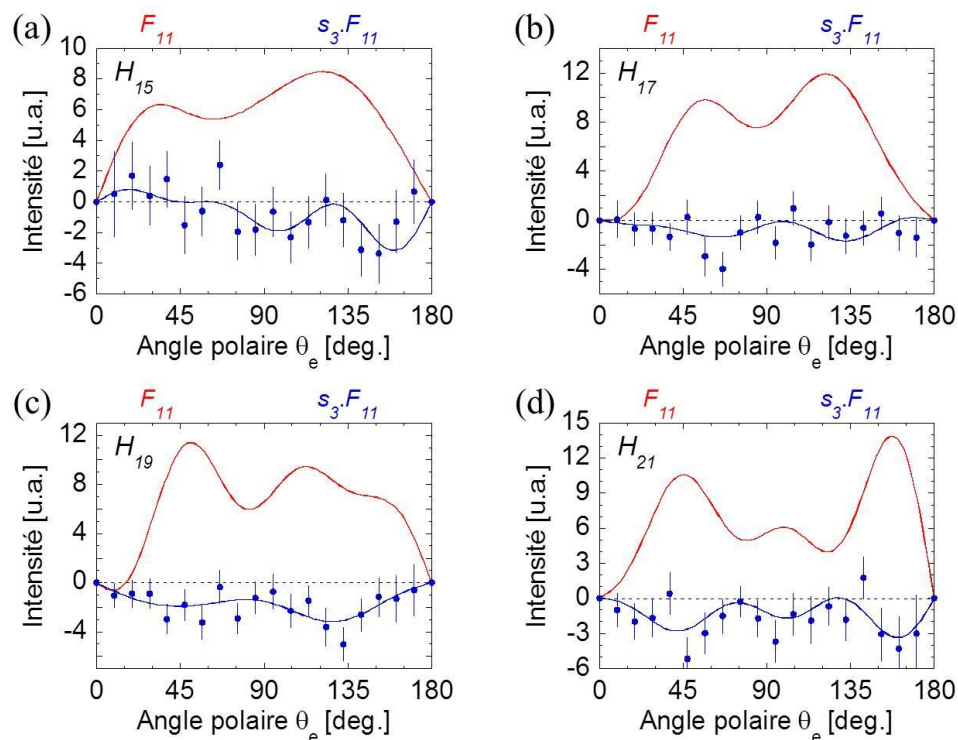
Figure V-19 : Produits s_3F_{11} (en bleu) et fonctions F_{11} de référence (en rouge) pour les harmoniques H15 (a), H17 (b), H19 (c) et H21 (d). Le trait plein bleu est un ajustement du produit s_3F_{11} par un développement en polynômes de Legendre.
