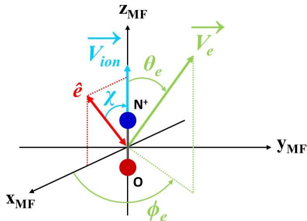
Figure III-2 : Définition des coordonnées sphériques (\theta_e, \phi_e) repérant l'émission du photoélectron dans le référentiel moléculaire.
