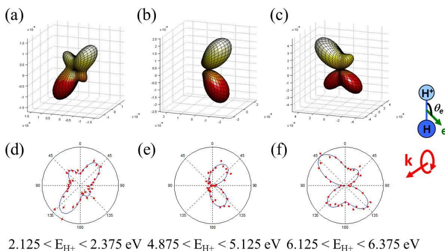
Figure VI-6 : MFPADs induites dans la PID de la molécule H_2 par une lumière polarisée circulairement à h\nu = 32.5 \text{ eV} , caractérisant le dichroïsme circulaire dans le référentiel moléculaire et correspondant aux énergies de l'ion fragment E_{H^+} = 2.25 (a), 5 (b) et 6.25 eV (c). Coupes correspondantes dans le plan de polarisation (d-f). L'axe moléculaire est perpendiculaire à la direction de propagation de la lumière et l'ion H^+ est émis vers le haut. Les MFPADs sont extraites des événements coïncidents ( H^+ , e^- ) contenus dans les bandes d'énergie centrées sur les valeurs E_{H^+} choisies, et d'une largeur de 0.25 eV cohérente avec la résolution sur l'énergie des ions dans ces expériences.
