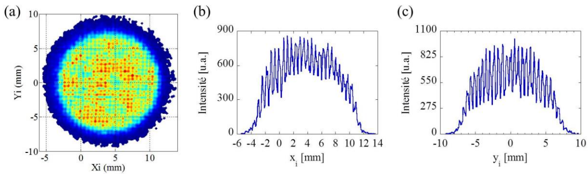
Figure I-11 : Image (x_i, y_i) des ions \text{N}^+ produits par la PID de la molécule NO (a), et distributions monodimensionnelles en x (b) et en y (c) obtenues par projection, en présence d'une grille spécifique de pas 550 \mu\text{m} .
