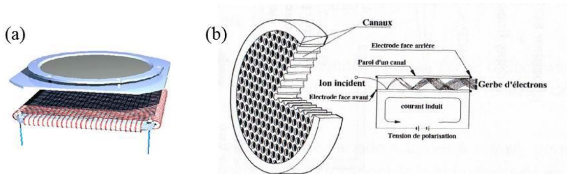
Figure I-5 : Schéma d'un détecteur sensible en temps et en position (a), et principe d'amplification d'une MCP (b).
