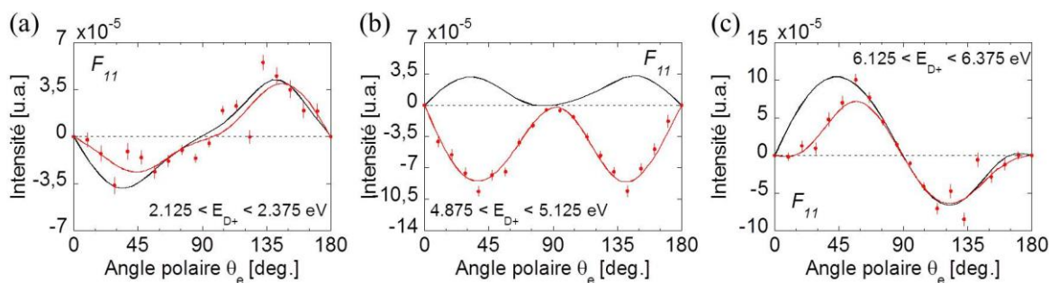
Figure VI-11 : Fonctions F_{11}(\theta_e) caractérisant les réactions de PID de la molécule D_2 produisant des ions fragments d'énergie E_{D^+} = 2.25 (a), 5 (b) et 6.25 eV (c) : expérience (points rouges) et théorie convoluée avec la fonction d'appareil (trait plein noir).
