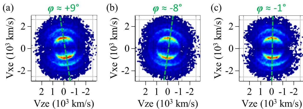
Figure V-14 : Diagrammes bidimensionnels ( V_{ze} , V_{xe} ) mesurés pour la PI de l'hélium induite par des harmoniques générées dans des molécules de N_2 alignées à +60^\circ (a), -60^\circ (b) et 0^\circ (c). La direction de l'axe principal de l'ellipse de polarisation est représentée par le trait vert en pointillé et repérée par rapport à la verticale par l'angle \varphi .
