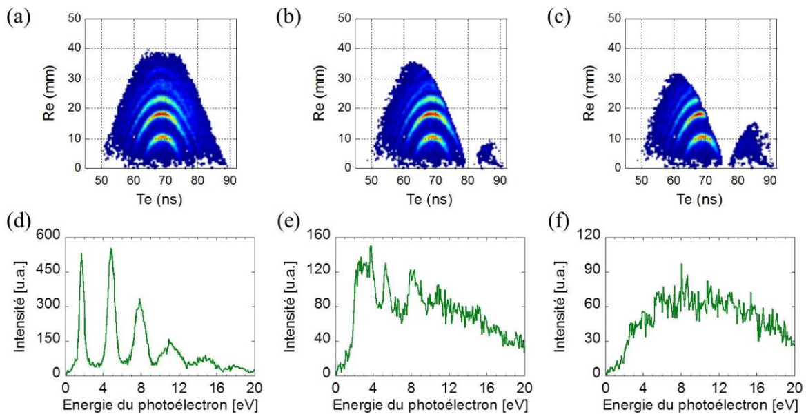
Figure II-7 : Diagrammes bidimensionnels ( T_e , R_e ) des événements coïncidents ( \text{He}^+ , e), issus de la PI d'atomes d'hélium induite par un train d'impulsions attosecondes contenant plusieurs longueurs d'onde, pour différentes amplitudes du champ magnétique renseignées dans le traitement : B = 7.9 G (a), B = 8.9 G (b) et B = 9.4 G (c). Spectres d'énergie cinétique des photoélectrons associés (d-f).
