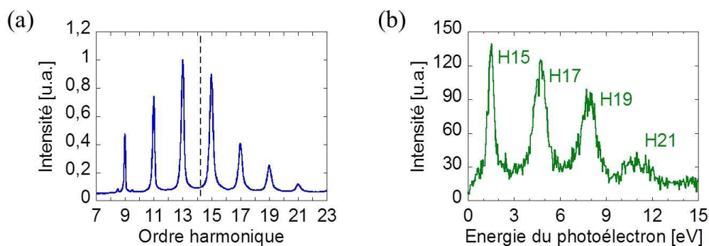
Figure V-16 : Spectre d'harmoniques d'ordre élevé générées dans des molécules de N_2 alignées à 60° par rapport à la polarisation verticale du laser de génération. Seules les harmoniques situées à droite de la ligne en pointillé, dont l'énergie est supérieure au potentiel d'ionisation de l'état c^3\Pi de la molécule cible NO, participent au processus de photoionisation (a). Spectre d'énergie cinétique des photoélectrons issus de la PID de NO correspondant (b).
