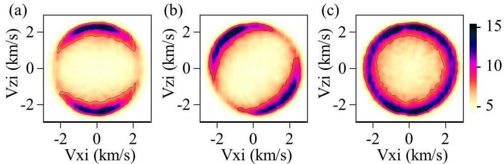
Figure IV-5 : Diagrammes bidimensionnels (V_{xi}, V_{zi}) des événements (N^+, e) représentant la projection de la sphère des vitesses des ions N^+ dans le plan de polarisation, pour différents états de polarisation de la lumière : linéaire (a), elliptique (b) et circulaire (c).
