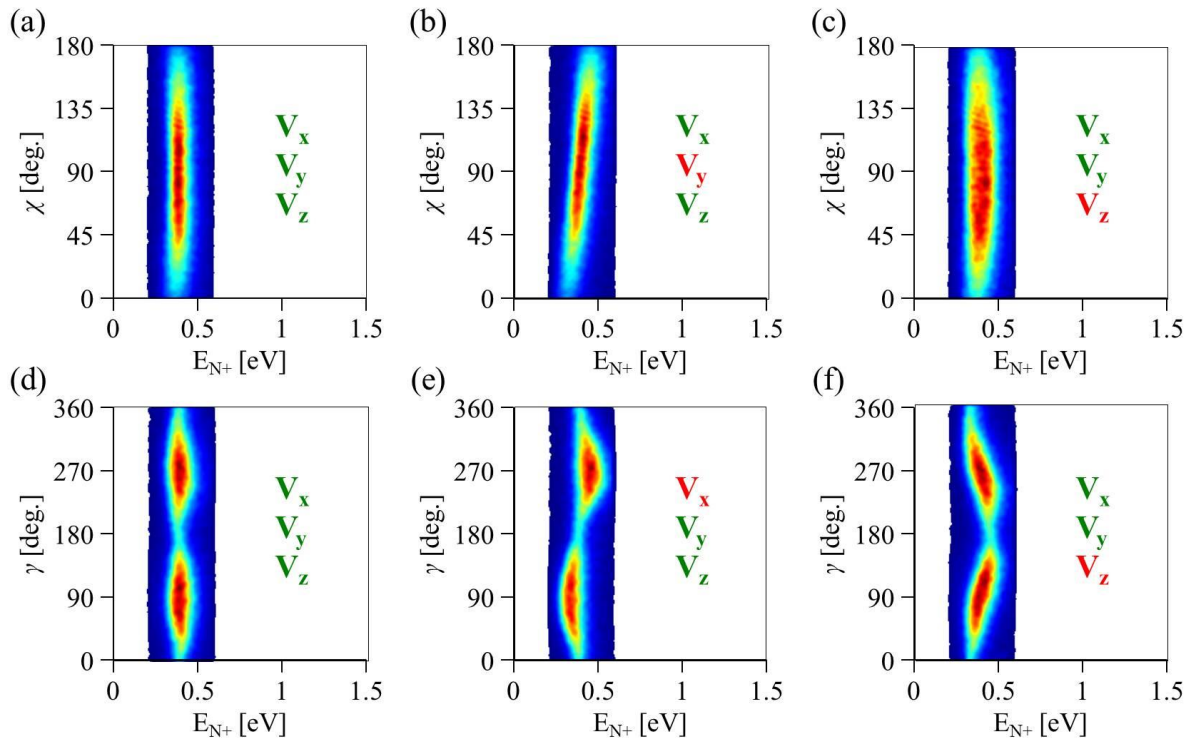
Figure II-6 : Diagrammes bidimensionnels (E_{N^+}, \chi) et (E_{N^+}, \gamma) pour différents centrages des trois composantes du vecteur vitesse des ions fragments N^+ : optimisés en vert et décentrés en rouge.
