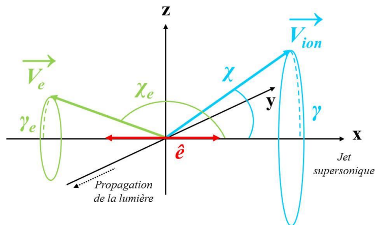
Figure III-1 : Emission d'un ion et d'un électron dans le référentiel du laboratoire induite par une lumière polarisée linéairement selon l'axe x .
