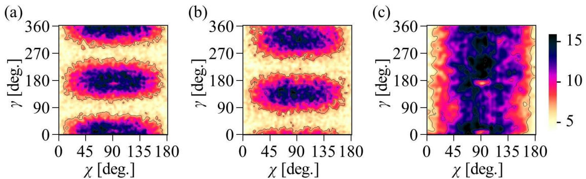
Figure IV-6 : Diagrammes bidimensionnels I(\chi, \gamma) des événements (N^+, e) induits par les trois états de polarisation mentionnés dans la Figure IV-5 : linéaire (a), elliptique (b) et circulaire (c).
