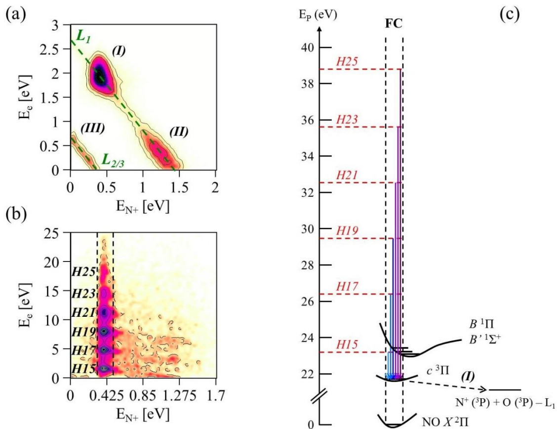
Figure V-4: KECDs résultant de la PID de la molécule NO induite par : le rayonnement synchrotron à une énergie de photon h\nu = 23.65 eV (a), un TIA contenant les harmoniques H15 à H25 (les traits verticaux en pointillé indiquent la sélection en énergie des événements associés au processus (I) induit par chaque harmonique) (b). Schéma présentant des courbes de potentiel de l'état fondamental de la molécule NO et des premiers états de l'ion moléculaire \text{NO}^+ , la première limite de dissociation ( L_1 ) et l'énergie des harmoniques utilisées (c).
