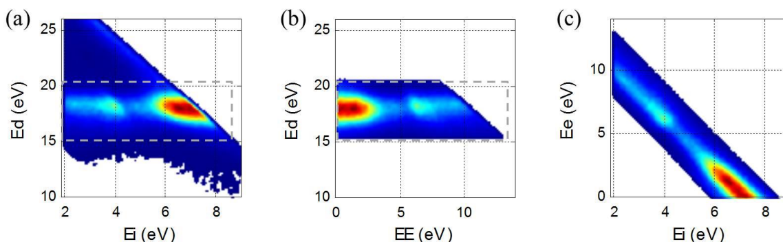
Figure II-9 : Diagrammes bidimensionnels (E_{H^+}, E_D) sans sélection (a) et (E_e, E_D) avec sélection en énergie (b), des événements ( H^+ , e ) issus de la PID de H_2 induite à h\nu = 32.5 eV. KECD (E_{H^+}, E_e) correspondant après avoir effectué la sélection en énergie définie par les cadres en pointillé (c).
