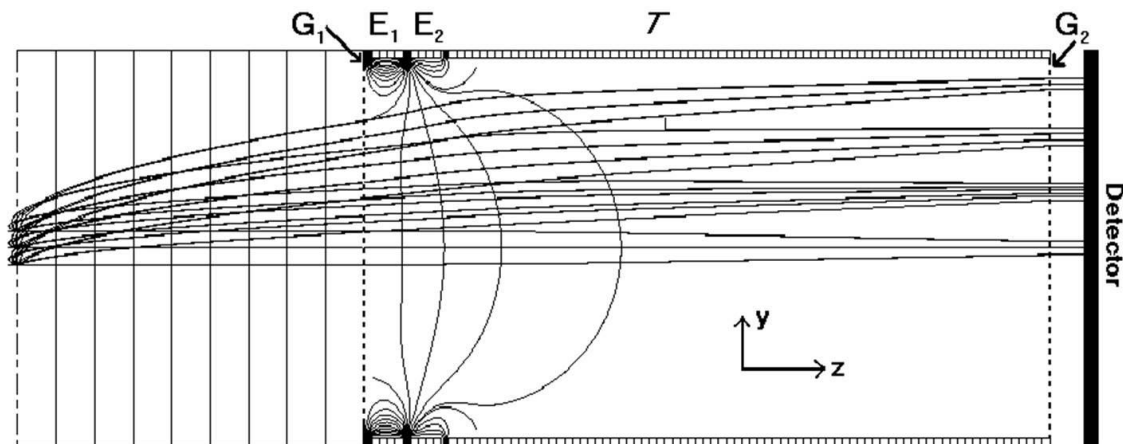
Figure I-3 : Simulation des trajectoires dans CV-40 avec les potentiels optimisés pour la focalisation.
