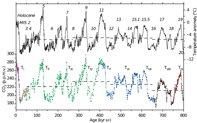
FIGURE 1.5 – Compilation de l’enregistrement de la concentration de CO 2 et de l’anomalie de température (par rapport à l’actuel) à EPICA Dôme C. Sur la courbe de la température sont indiqués les stades isotopiques. Les terminaisons sont indiquées sur la courbe du CO 2 . Figure provenant de Lüthi et al. (2008).
