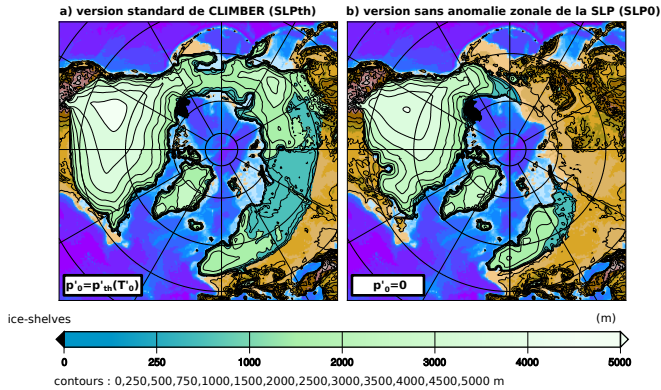
FIGURE 2.5 – Hauteur et géométrie des calottes simulées par CLIMBER-GRISLI à 21ka (a) avec la version d'origine de CLIMBER et (b) avec la version où la paramétrisation des ondes stationnaires a été supprimée.
