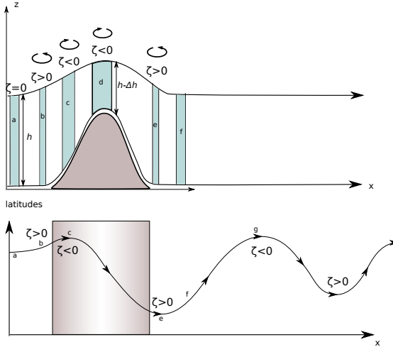
FIGURE 1.14 – Formation d'une onde de Rossby forcée par un relief : a) La vorticité relative étant nulle, la conservation de la vorticité potentielle indique : f/h = K , avec K une constante.
