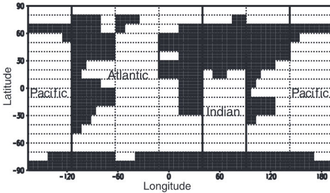
FIGURE 2.1 – Représentation de la géographie de CLIMBER : les tirets représentent la grille atmosphérique tandis que les lignes pleines délimitent les trois bassins océaniques. Source : (Petoukhov et al. 2000)
