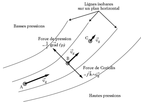
FIGURE 1.11 – Le vent géostrophique est tangent aux lignes isobares sur un plan horizontal. Son intensité est proportionnelle au gradient de pression. (D'après Malardel (2005))
