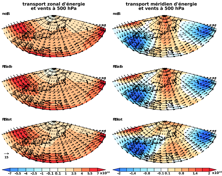
FIGURE 4.9 – Transport d'énergie zonal (à gauche) et méridien (à droite) pour chaque expérience en moyenne sur l'hiver ( \text{J}\cdot\text{m}^{-1}\cdot\text{s}^{-1} ). Winter zonal (left) and meridional (right) energy transport for the three experiments ( \text{J}\cdot\text{m}^{-1}\cdot\text{s}^{-1} ).
