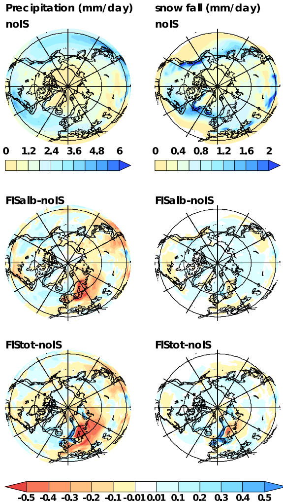
FIGURE 4.5 – Similaire à la figure 4.4 pour la précipitation (liquide et solide) et les chutes neigeuses en moyenne annuelle (mm/jour). Same as figure 4.4 for annual precipitation (liquid and solid) and annual snowfall (mm/day).
