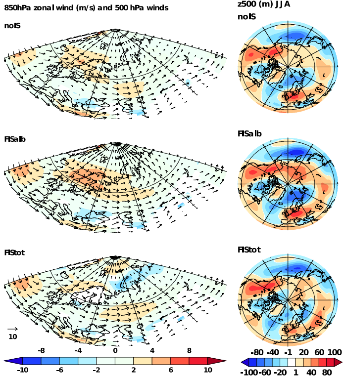
FIGURE 4.10 – Gauche : Vent zonal à 850 hPa (couleurs) et vent moyen à 500 hPa (flèches) en moyenne estivale (juin-juillet-août) ( m \cdot s^{-1} ). Droite : anomalie zonale de la hauteur de géopotential à 500 hPa en moyenne estivale (m).
