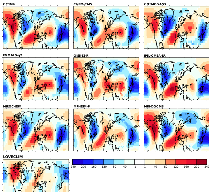
FIGURE 3.3 – Anomalie zonale de la hauteur de géopotential à 500 hPa (m) en hiver boréal (DJF) pour chaque modèle participant à PMIP 3 pour la simulation du dernier maximum glaciaire (DMG). Zonal anomaly of 500 hPa geopotential height (m) in winter (DJF) coming from each PMIP 3 model for Last Glacial Maximum (LGM).
