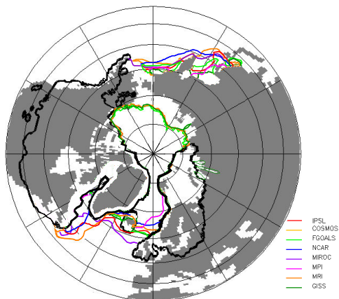
FIGURE 3.5 – Limite où la fraction de glace de mer est supérieure à 50% dans une maille du modèle en hiver pendant le DMG. Cette variable n'était pas accessible pour COSMOS.
