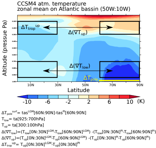
FIGURE 3.11 – Schéma expliquant les différents champs de température testés pour trouver une explication au décalage du jet. Visualization of the temperature differences tested in order to find a correlation with the jet stream shift between LGM and PI.
