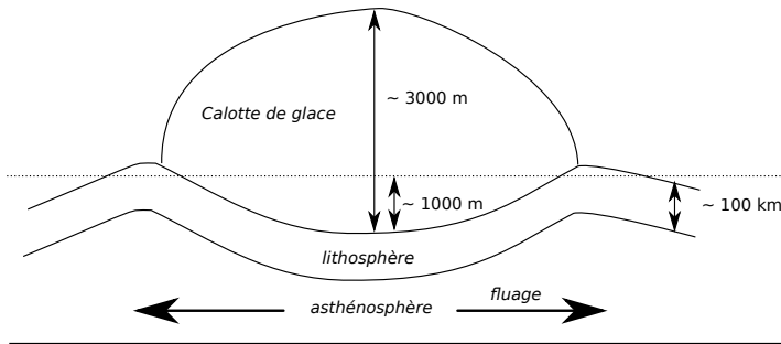
FIGURE 2.3 – Schéma expliquant le phénomène d'ajustement isostatique sous une calotte de glace.
