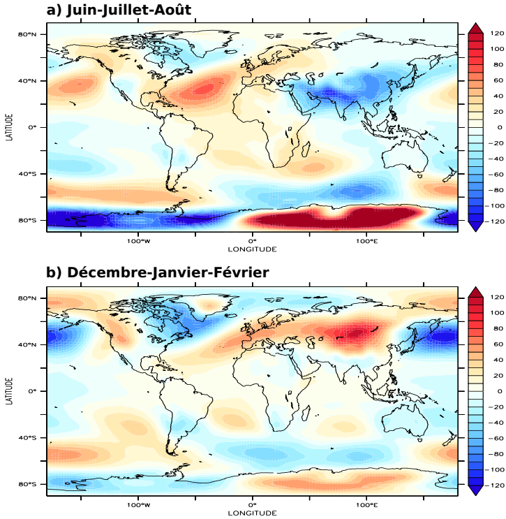
FIGURE 1.15 – Anomalie zonale de la hauteur de géopotential à 850 hPa (m) pour (a) l'été boréal et (b) l'hiver boréal : moyenne sur 1950-2000. (Données : réanalyses NCEP)
