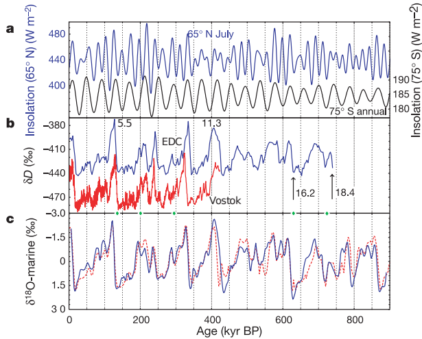
FIGURE 1.4 – Comparaison des données d’EPICA Dôme C avec l’insolation et d’autres types d’enregistrements (EPICA members 2004). (a) courbe bleue : insolation à 65^\circ\text{N} en juillet, courbe noire : insolation annuelle moyenne à 75^\circ\text{S} , à la latitude de Dôme C. (b) traceur de la température, le ratio deutérium/hydrogène ( \delta D ) dans la glace à Dôme C (courbe bleue) et à Vostok (courbe rouge), ces deux stations étant situées en Antarctique. (c) Enregistrement du rapport isotopique de l’oxygène de carottes marines de basses latitudes, traceur de l’évolution du niveau marin. Courbe bleue : Bassinot et al. (1994), courbe en pointillés rouge : Imbrie et al. (1993).
