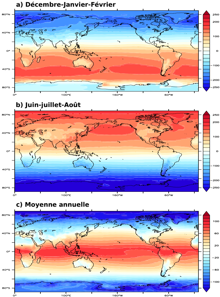
FIGURE 1.9 – Bilan radiatif au sommet de l’atmosphère avec un ciel sans nuages : différence entre le flux solaire incident et les flux sortants (infrarouge et solaire), en W \cdot m^{-2} . Moyenne sur l’hiver boréal (a), l’été boréal (b) et annuelle (c) sur la période 1960-2010.
