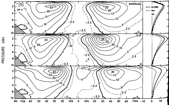
FIGURE 1.13 – Coupe méridienne de la moyenne zonale de la composante zonale du vent en \text{m}\cdot\text{s}^{-1} en moyenne annuelle (panneau du haut), en DJF (moyenne sur Décembre-Janvier-Février) (panneau du milieu) et JJA (moyenne sur Juin-Juillet-Aout) (panneau du bas). À droite, les profils verticaux en moyenne sur les latitudes du globe (trait plein gras), de l'hémisphère nord (trait plein fin) et de l'hémisphère sud (tiretés) ((Peixoto et Oort 1992) pages 154 figure 7.15).
