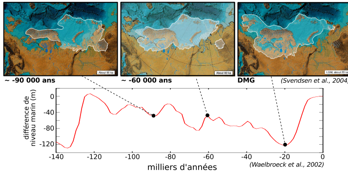
FIGURE 4.12 – Extension de la calotte eurásienne à différents stades de la glaciation d'après les reconstructions de Svendsen et al. (2004), et différence de niveau marin par rapport au présent provenant de Waelbroeck et al. (2002).
