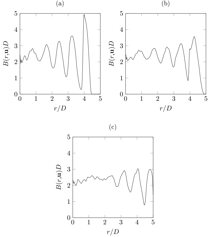
FIGURE 3.17 – Coefficients radiatifs B pour l'empilement B , pour \mathbf{u} = \mathbf{e}_r (a), (\mathbf{u}, \mathbf{e}_r) = 0.5 et \varphi = 0 (b), et \mathbf{u} = -\mathbf{e}_r (c).
