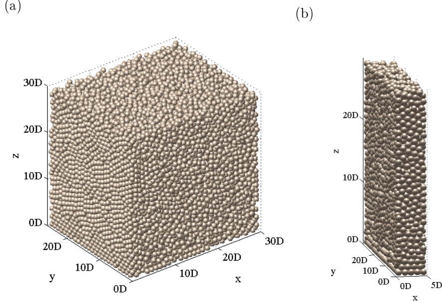
FIGURE 2.2 – Empilement de sphères entre deux plans d'équations x = 0 et x = L_x engendrés numériquement pour : Figure(a) L_x \simeq 30D ; Figure(b) L_x \simeq 5D
