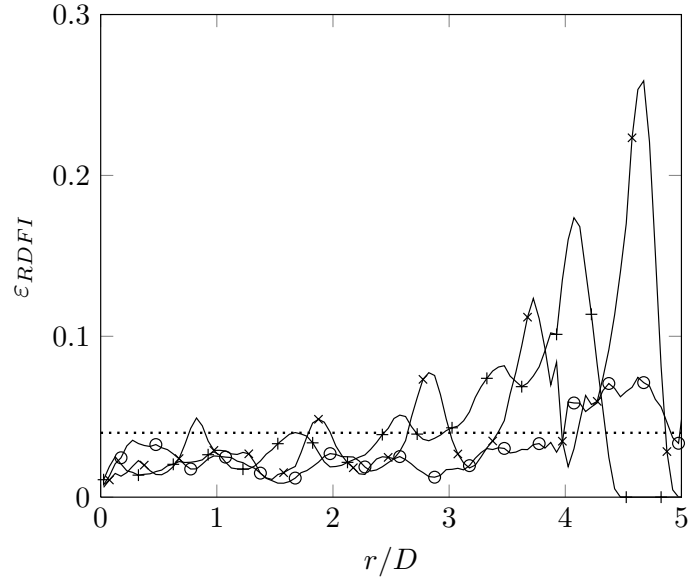
FIGURE 3.20 – Empilement B : valeur du critère \varepsilon_{RDFI}(r, \mathbf{u}) pour \varphi = 0 et \mathbf{u} = \mathbf{e}_r (+) ; (\mathbf{u}, \mathbf{e}_r) = -0.2 (×) ; \mathbf{u} = -\mathbf{e}_r (o) et limite de validité \varepsilon_{RDFI}(x, \mathbf{u}) = 4\% (courbe pointillée).
