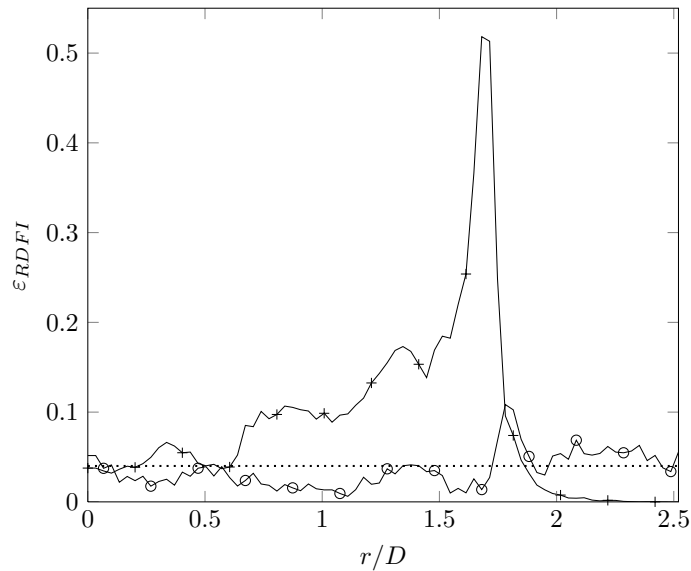
FIGURE 3.21 – Empilement C : valeur du critère \varepsilon_{RDFI}(r, \mathbf{u}) pour \varphi = 0 et \mathbf{u} = \mathbf{e}_r (+) ; (\mathbf{u} \cdot \mathbf{e}_r) = -0.6 (o) et limite de validité \varepsilon_{RDFI}(x, \mathbf{u}) = 4\% (courbe pointillée).
