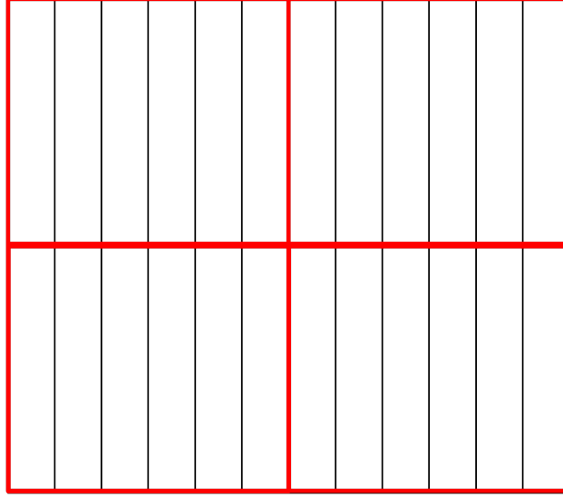
FIGURE 2.6 – En 2D, 4 zones délimitées par les traits rouges sont représentées. Ces zones peuvent contenir plusieurs particules ; les volumes élémentaires, délimités par des traits noirs, sont eux petits par rapport à la taille des particules. Les zones n’ont pas d’autre utilité que de diminuer les temps de calcul lorsque l’empilement est de grande taille.
