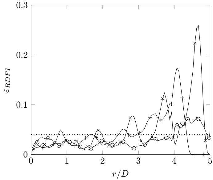
FIGURE 3.20 – Empilement B : valeur du critère \varepsilon_{RDFI}(r, \mathbf{u}) pour \varphi = 0 et \mathbf{u} = \mathbf{e}_r (+) ; (\mathbf{u} \cdot \mathbf{e}_r) = -0.2 (x) ; \mathbf{u} = -\mathbf{e}_r (o) et limite de validité \varepsilon_{RDFI}(x, \mathbf{u}) = 4\% (courbe pointillée).
